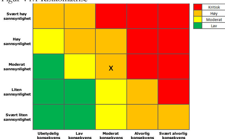
Figur V1.1 Risikomatrise
