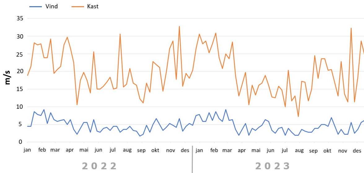
Figur 6. Gjenomsnitt av daglig maksimal vindhastighet (m/s, blå linje) og maksimalt vindkast (m/s, oransje linje) per uke i perioden 1. januar 2022 til 31. desember 2023 (ett datapunkt per uke). Maksimal vindhastighet i denne perioden ble målt i november 2022 og var 32.8 m/s (118 km/t). Vinden blåste 16.7 m/s (60 km/t) eller mer på 207 av disse dagene, og oversteget 10 m/s (36 km/t) hele 515 dager. Vindhastigheten på avlsstasjonen er målt ved bruk av en Netatmo værstasjonen med tilkoblet anemometer (nøyaktighet = 0.5 m/s).
