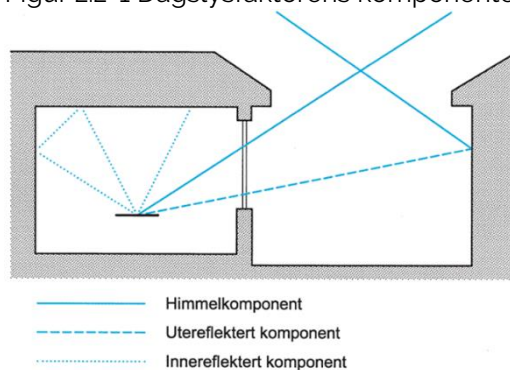
Figur 2.2-1 Dagslysfaktorens komponenter 8
