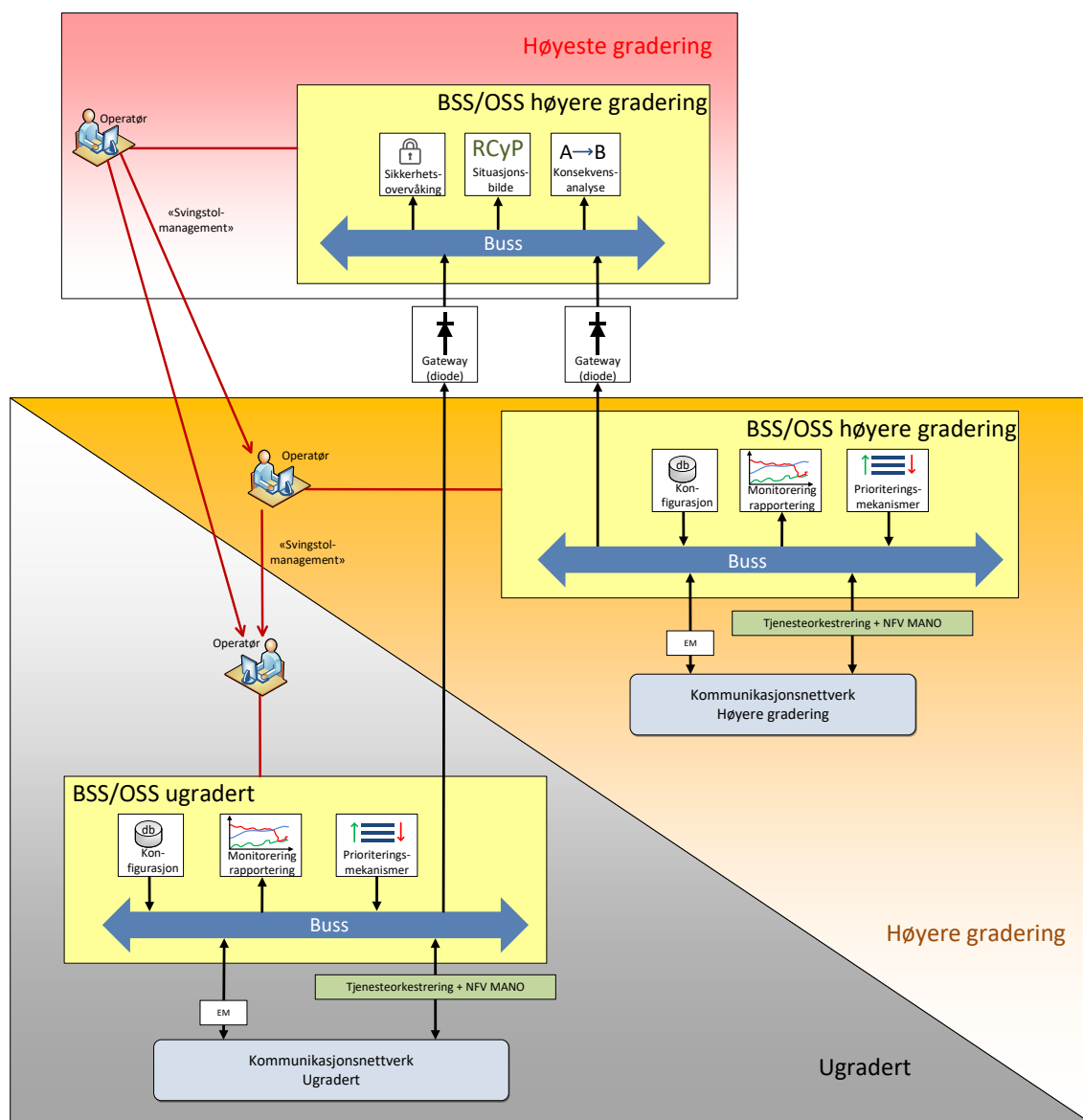
Figur 5.2 Helhetlig løsning for managementløsninger for stasjonær kommunikasjonsinfrastruktur.
