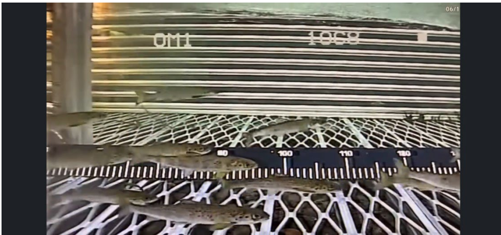
Figur 8.1. Skjerm bilde fra videoovervåkingen av fangstkammeret i Kongsfjordelva, som viser en stim med smolt som har svømt mellom spilene på vei mot havet. Foto: Håvard Vistnes
