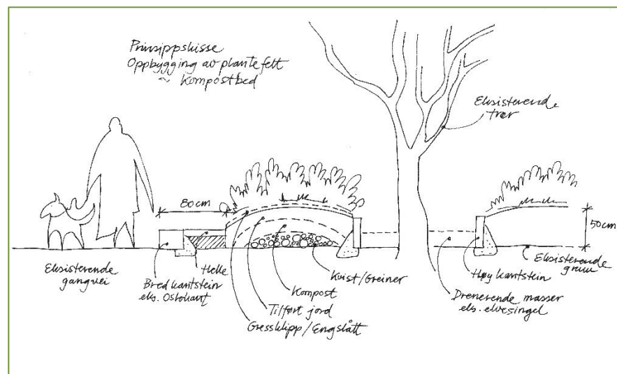
FIGUR 81 PRINSSNITT FOR OPPBYGGING AV PLANTEFELT, KOMPOSTBED.
