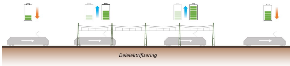
Figur 19 Prinsippsskisse av deelektrifisering.
