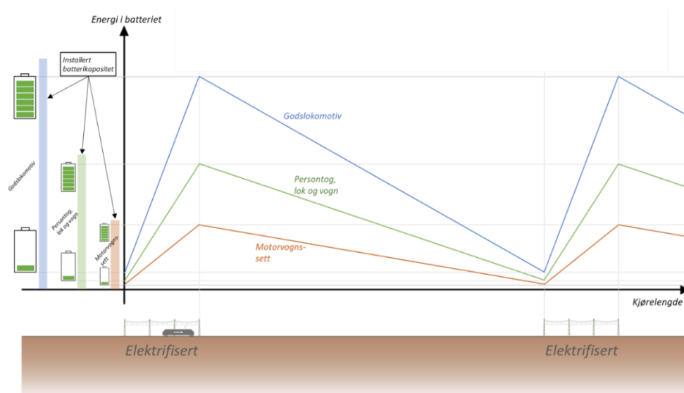
Figur 17: Prinsipper for hvordan installert energimengde og ladeeffekt vil optimaliseres i sammenheng med deelelektrifiseringen for å oppnå en gunstig utnyttelse av batterikapasiteten i de forskjellige kjøretøyene. Merk at stigningen på kurvene som viser aktuell ladestatus for de tre forskjellige kjøretøyene representerer ladeeffekten og forbrukseffekten, der godstoget (trukket av godsløkomotivet) vil ha den høyeste effekten. I dette eksemplet er det illustrert en margin i den brukte batterikapasiteten i forhold til den installerte batterikapasiteten.
