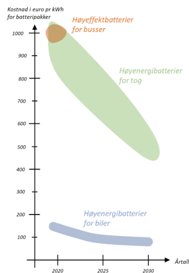
Figur 16: Forventet prisutvikling frem mot 2030 for batteripakker til henholdsvis tog og biler. Figur er basert på informasjon i delrapport 1.
