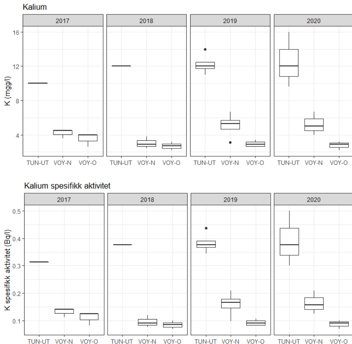
Figur 29. Boksdiagram med minimum-, 25% kvartil-, median-, 75% kvartil- og maksimum konsentrasjoner av kalium (mg/L) og kalium spesifikk aktivitet (Bq/l) i Vøyenbekken opp- og nedstrøms, samt TUN-UT fra 2017-2020. Punkter viser minimum eller maksimum utliggere.
