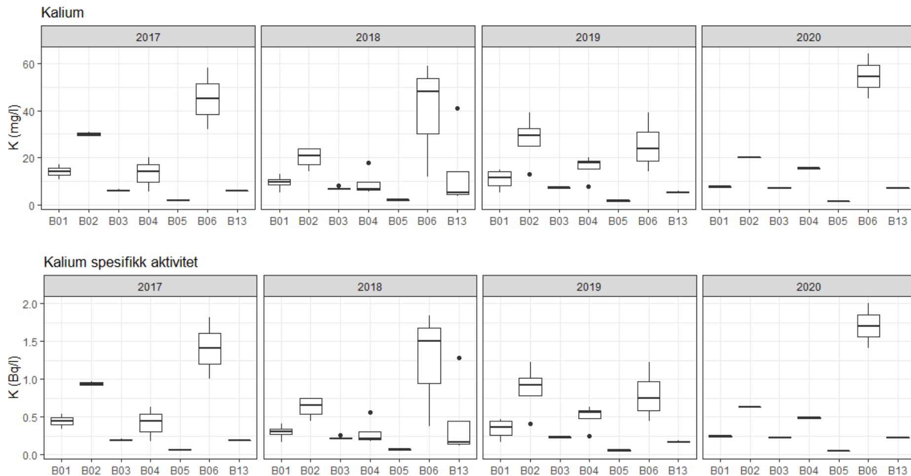
Figur 23. Boksdiagrammet minimum-, 25% kvartil-, median-, 75% kvartil- og maksimum verdier for kalium (mg/l) og kalium spesifikk aktivitet (Bq/l), i brønnene B01 til B13 fordelt på år. Punkter viser minimum eller maksimum utliggere.
