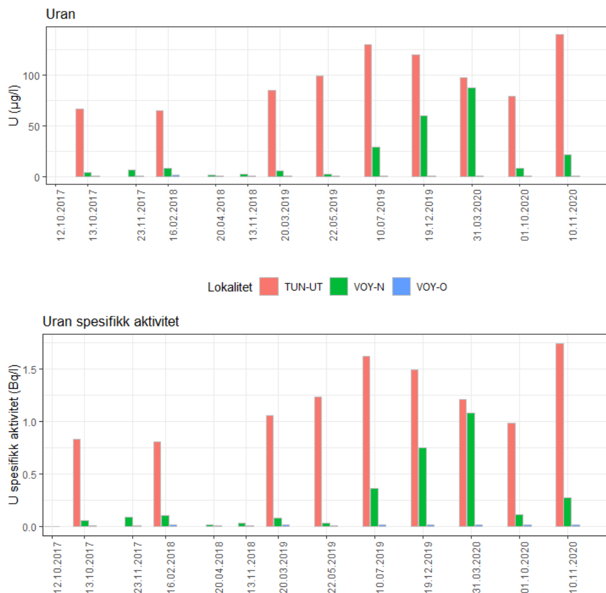
Figur 26. Søylediagram med konsentrasjoner av uran ( \mu\text{g/l} ) og uran spesifikk aktivitet (Bq/l) i Vøyenbekken opp- og nedstrøms, samt TUN-UT i perioden 2017-2020.
