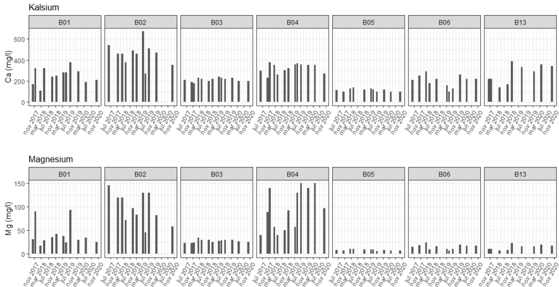
Figur II_1. Konsentrasjoner av kalsium (mg/l) og magnesium (mg/l) i brønnene B01-B13 fra 2017-2020.
