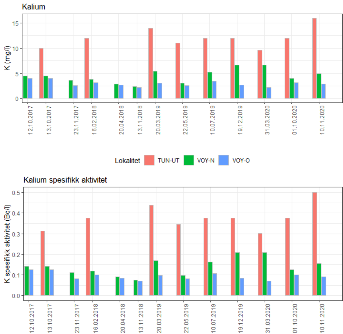
Figur 28. Søylediagram med konsentrasjoner av kalium (mg/L) og kalium spesifikk aktivitet (Bq/l) i Vøyenbekken opp- og nedstrøms, samt TUN-UT i perioden 2017-2020.
