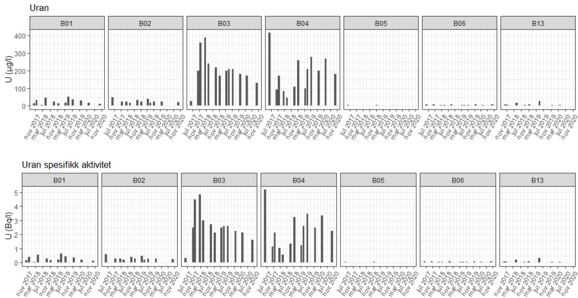
Figur 20. Søylediagram med uran ( \mu\text{g/L} ) og uran spesifikk aktivitet ( \text{Bq/l} ) i brønnene B01-B13 fra perioden 2017-2020.
