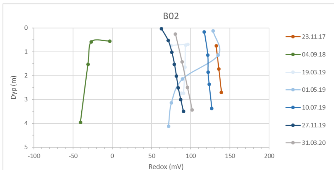
Figur 9. Redokspotensiale i brønnen B02 for alle prøvetakingsrunder fra 2017-2020.
