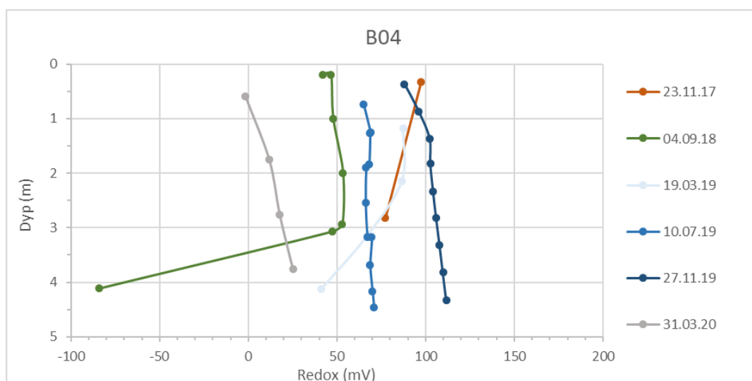
Figur 11. Redokspotensiale i brønnen B04 for alle prøvetakingsrunder fra 2017-2020.
