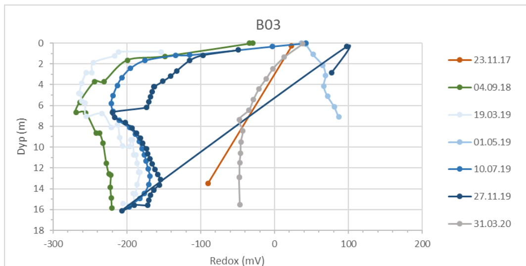
Figur 10. Redokspotensiale i brønnen B03 for alle prøvetakingsrunder fra 2017-2020.
