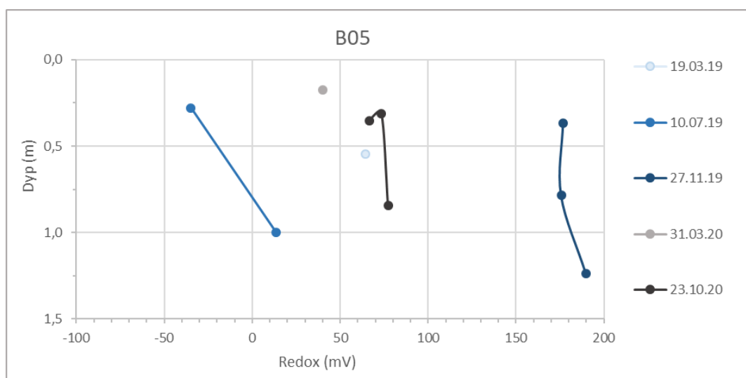
Figur 12. Redokspotensiale i brønnen B05 for alle prøvetakingsrunder fra 2019-2020.
