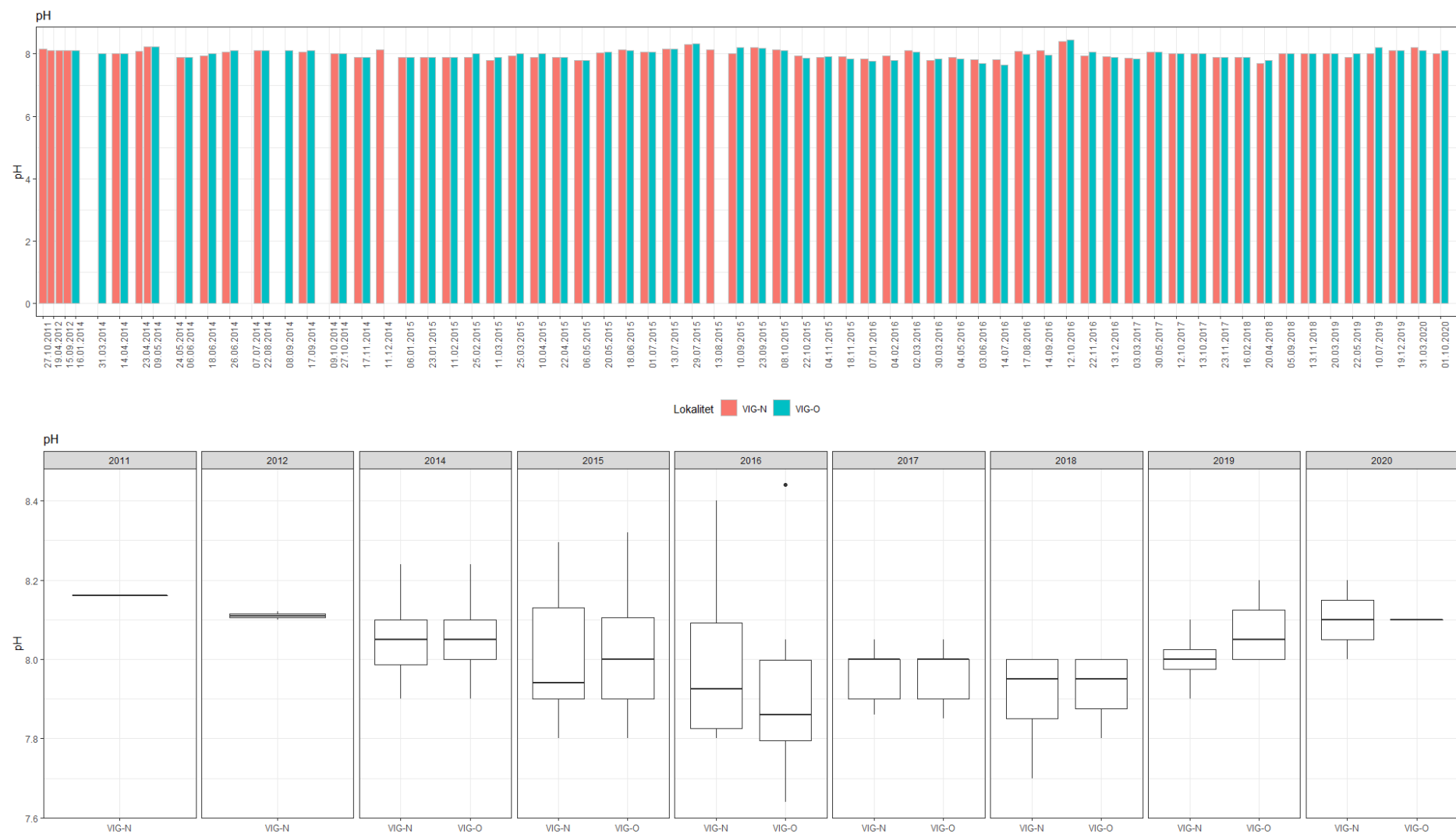
Figur IV_5. Barplot med pH og boksplot med minimum-, 25% kvartil-, median-, 75% kvartil- og maksimum pH i Vigga opp- og nedstrøms deponiet fra 2011-2020. Punkter viser minimum eller maksimum utliggere.
