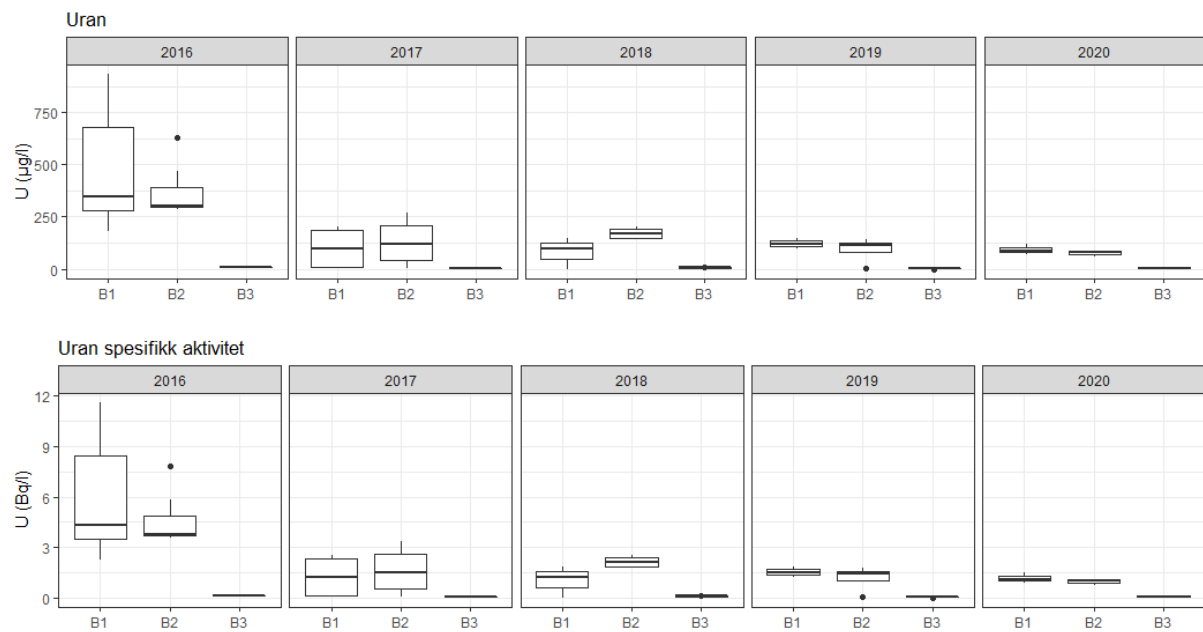
Figur 16. Boksdiagram med minimum-, 25% kvartil-, median-, 75% kvartil- og maksimum verdier for Uran (µg/l) og Uran spesifikk aktivitet (Bq/l), i brønnene B1-B3 fordelt på år. Punkter viser minimum eller maksimum utliggere.
