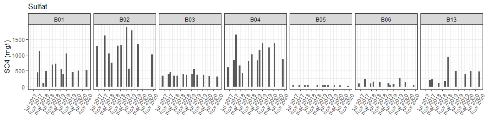
Figur 25. Søylediagram med konsentrasjoner av sulfat (mg/l) i brønnene B01-B13 fra 2017-2020.
