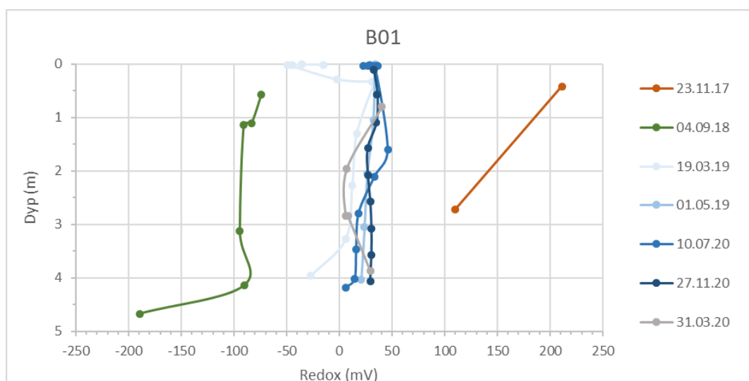
Figur 8. Redokspotensiale i brønnen B01 for alle prøvetakingsrunder fra 2017-2020.
