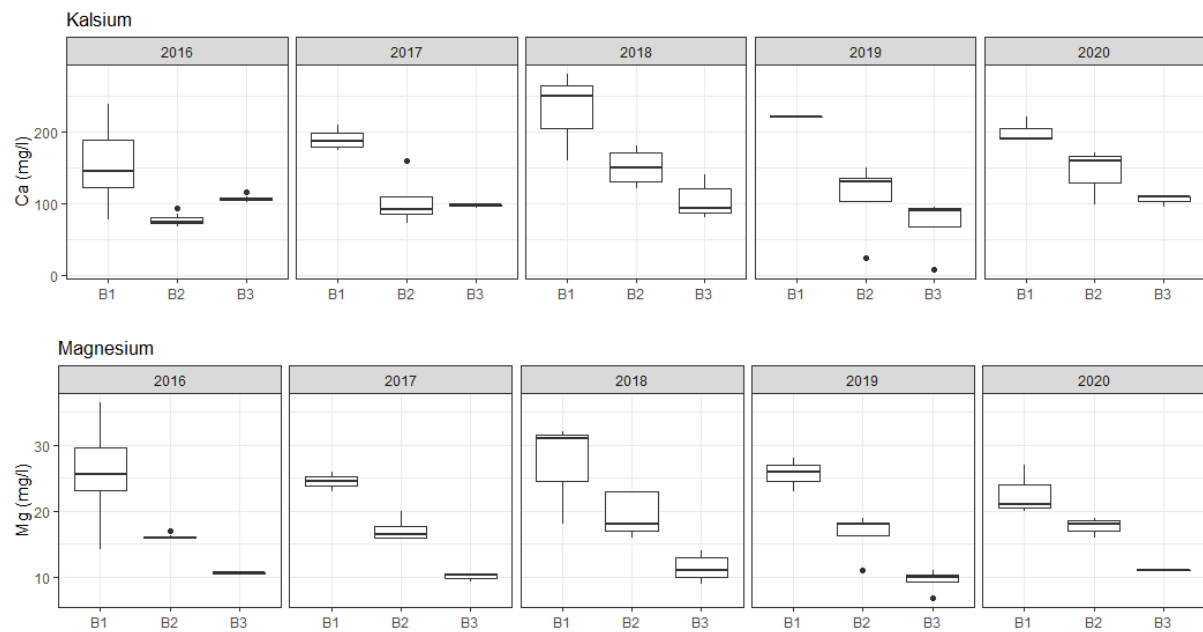
Figur I_2. Boksplot med minimum-, 25% kvartil-, median-, 75% kvartil- og maksimum verdier for U og SO 4 , i brønnene B1-B3 for hele prøvetaksperioden. Punkter viser minimum eller maksimum utliggere.
