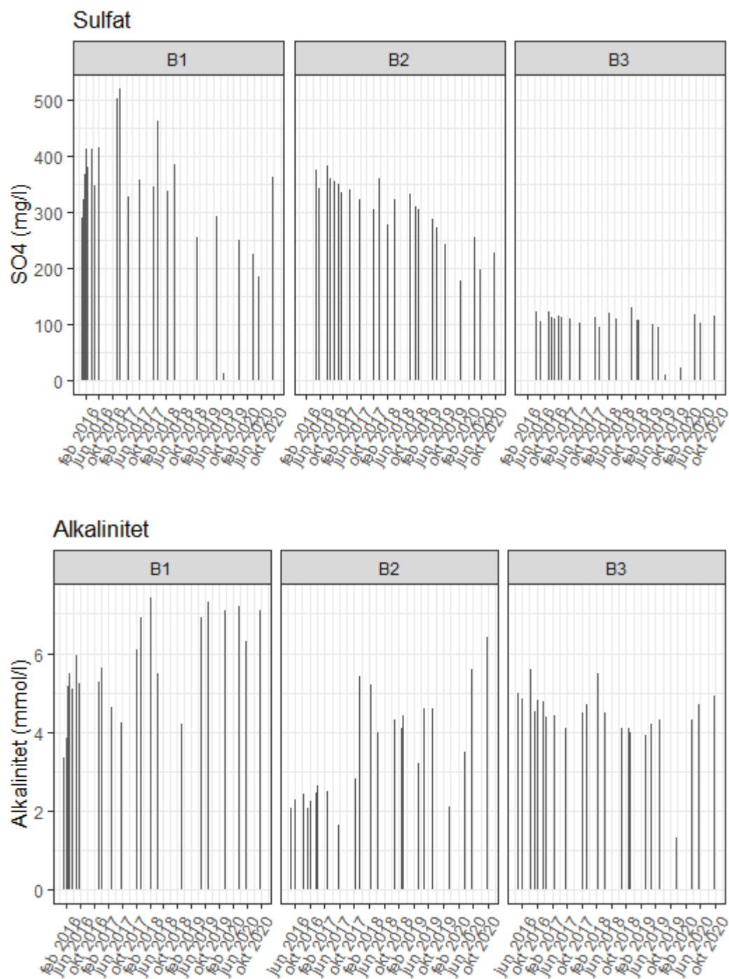
Figur I_3. Konsentrasjon av sulfat (mg/l) og alkalinitet (mmol/L) i brønnene B1 til B3 fra 2016-2020.
