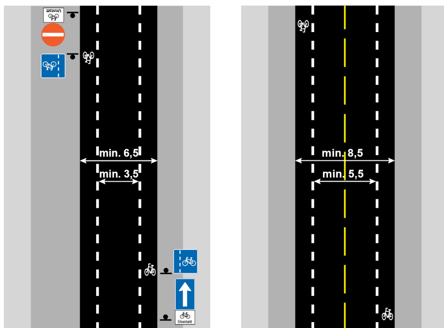
Figur 8.2—1 — Minimum veg- og kjørefeltbredde ved oppmerking av sykkelfelt i gate med henholdsvis ett (envegsregulert) og 2 kjørefelt
