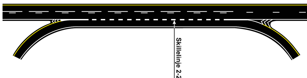
Figur 7.6.8—1 — Oppmerking av vekslingsstrekning
