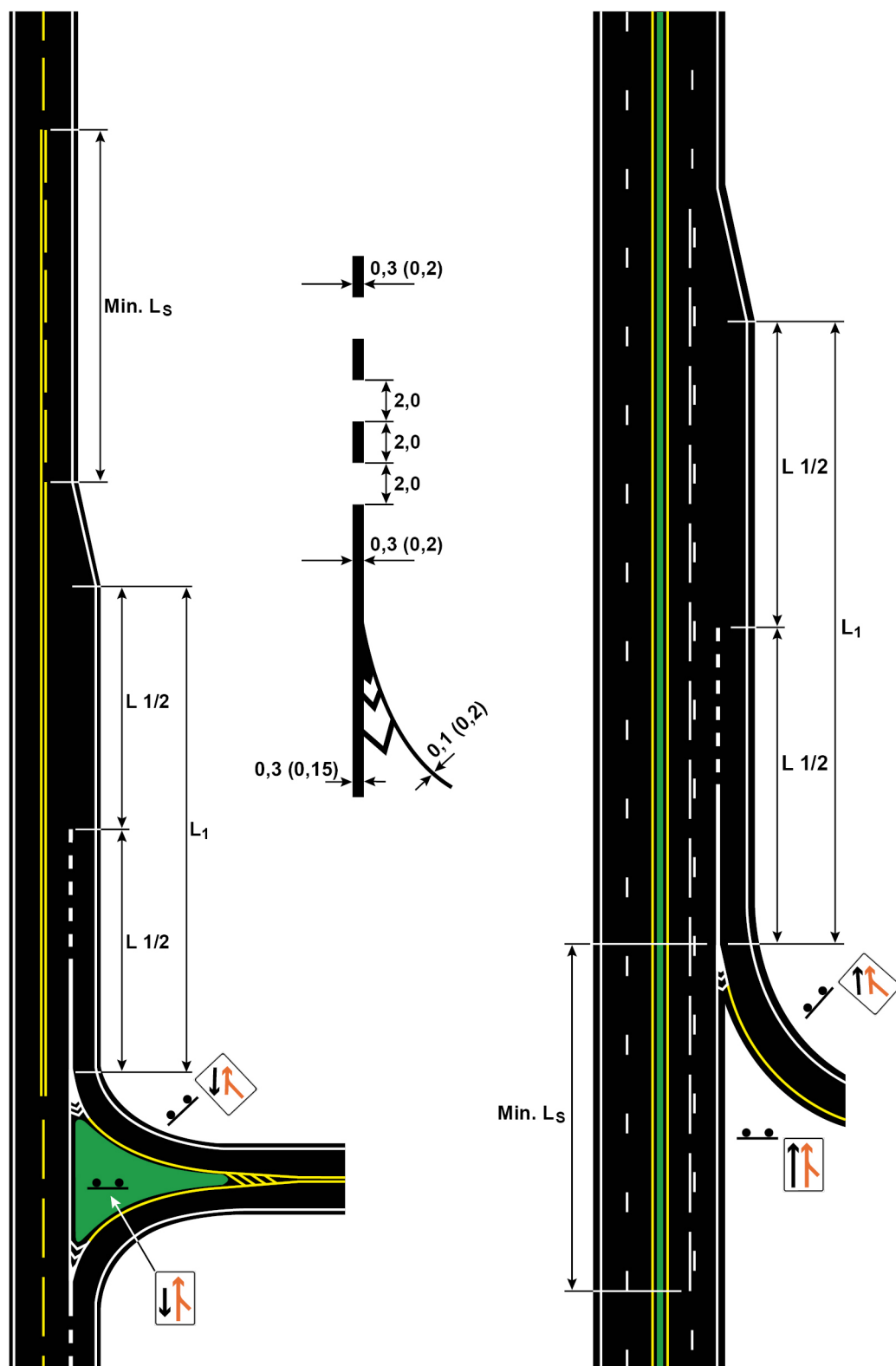
Figur 7.6.5—1 — Oppmerking av akselerasjonsfelt
