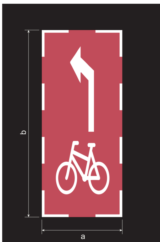
Figur 8.5—2 — Dimensjoner for venteboks
