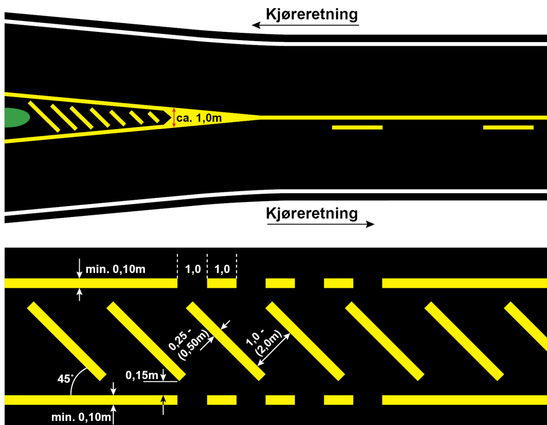
Figur 3.2—2 — Utforming og dimensjoner for sperreområder som skiller kjøreretningene
