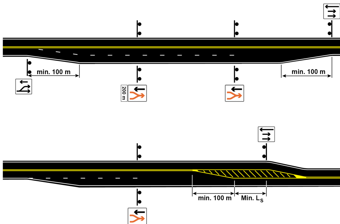
Figur 5.5—1 — Krav til oppmerking av forbikjøringsfelt
