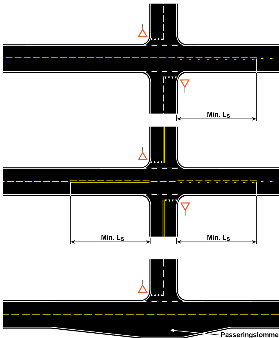
Figur 7.3.1—1 — Eksempler på oppmerking i vikepliktsregulerte kryss uten kanalisering
