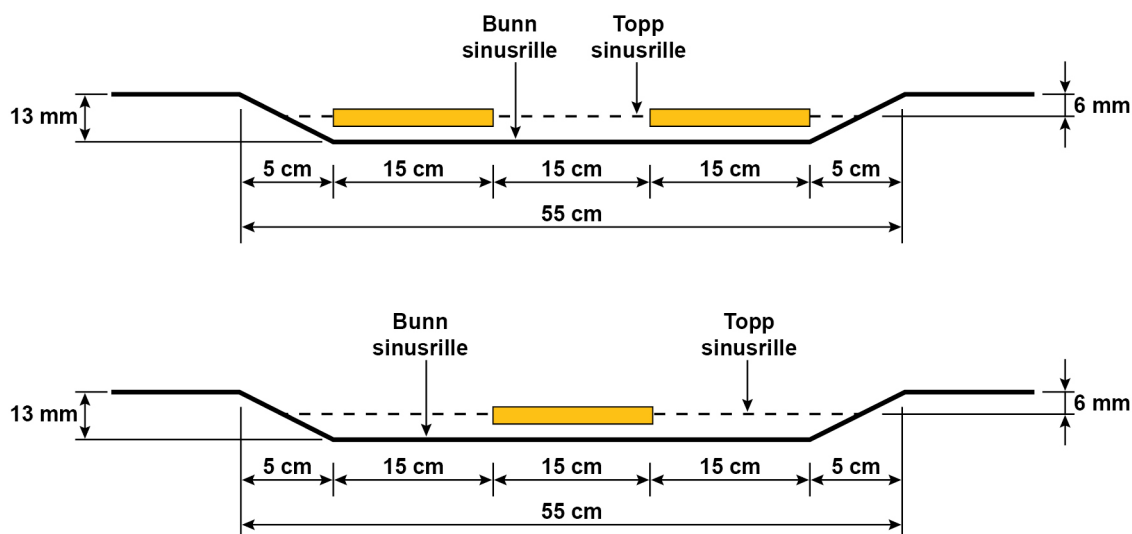
Figur 6.3.1—2 — Utforming av fresespor med 0,55 m bredde med henholdsvis dobbel sperrelinje og varsellinje/kjørefeltlinje
