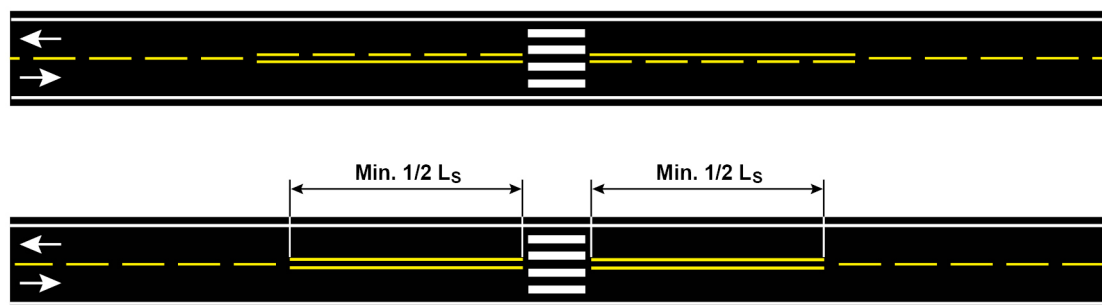
Figur 8.1—5 — Middlinje foran gangfelt ved fartsgrense 60 km/t
