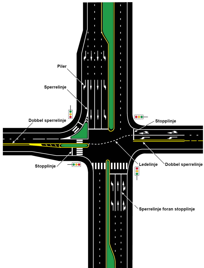
Figur 7.5—1 — Oppmerking i signalregulert kryss
