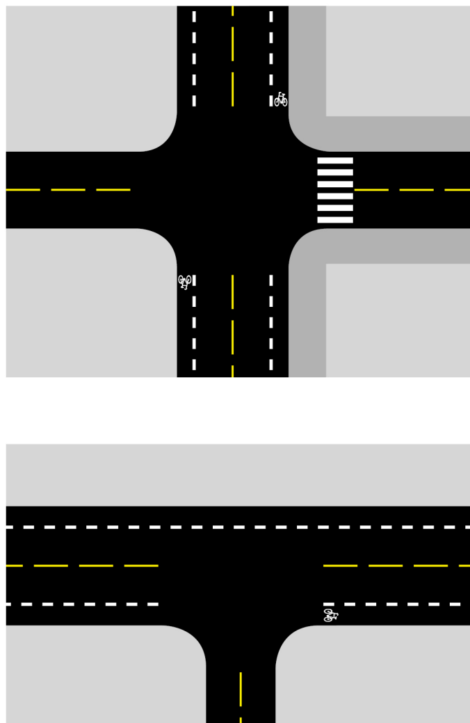
Figur 8.3—1 — Oppmerking av sykkelfelt i høyreregulerte T- og X-kryss
