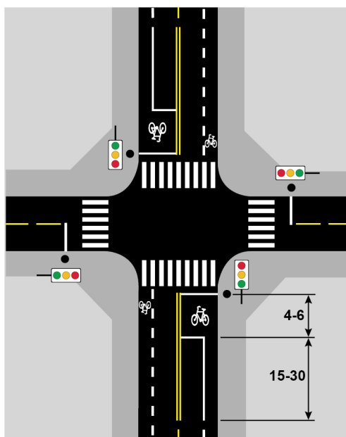
Figur 8.4—2 — Sykkelboks i signalregulert kryss - ikke forkjørsveg
