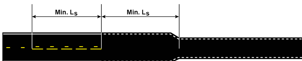
Figur 5.4—1 — Overgang mellom 2-feltsveg og 1-feltsveg
