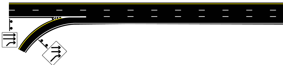
Figur 7.6.7—1 — Oppmerking av feltaddisjon
