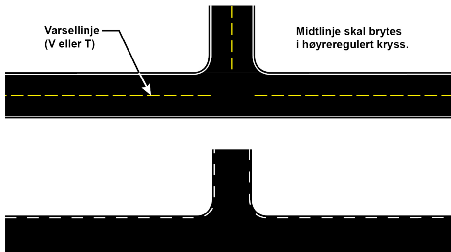
Figur 7.2—1 — Høyreregulert kryss
