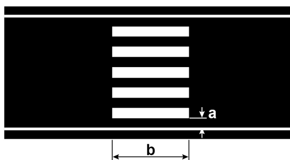
Figur 8.1—1 — Utforming av gangfelt
