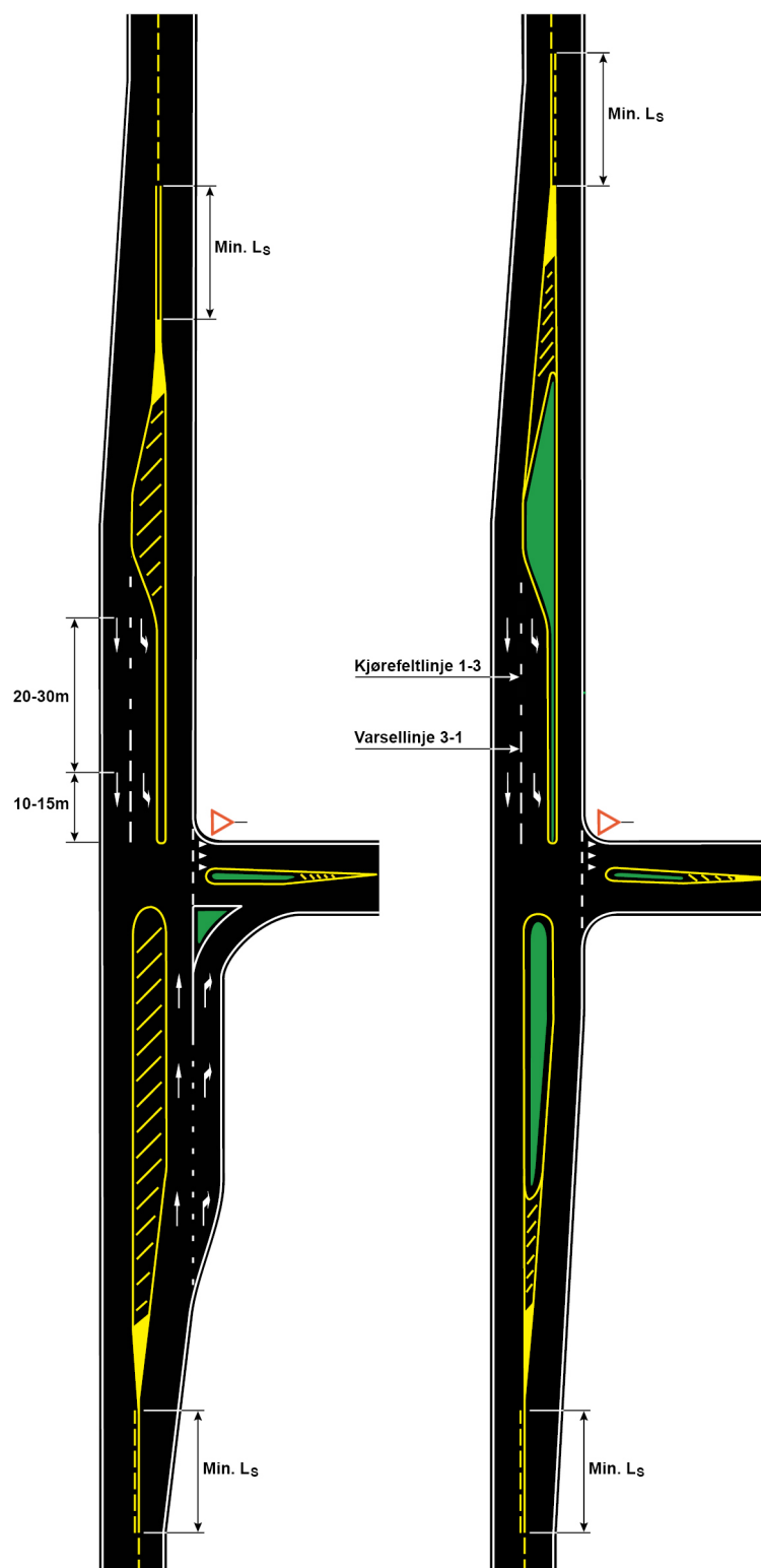
Figur 7.3.2—1 — Vikepliktsregulerte kryss med kanalisering ved fartsgrense \geq 60 km/t
