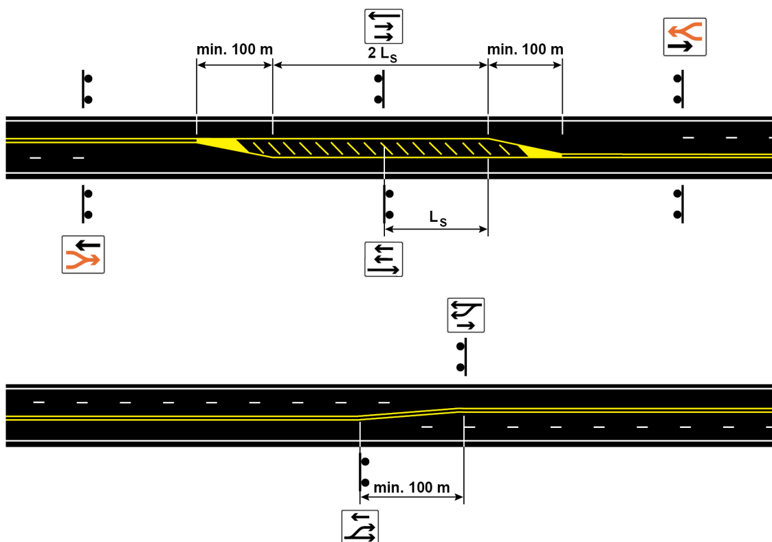
Figur 5.5—2 — Krav til oppmerking ved veksling av kjøreretning i midtfeltet på 3-feltsveg
