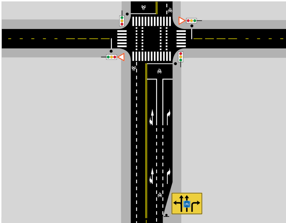
Figur 8.4—4 — Signalregulert kryss med sykkelboks og midtstilt sykkelfelt
