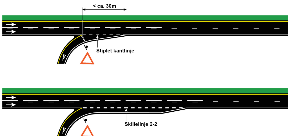
Figur 7.6.6—1 — Oppmerking med vikeplikt av ufullstendig påkjøringsfelt
