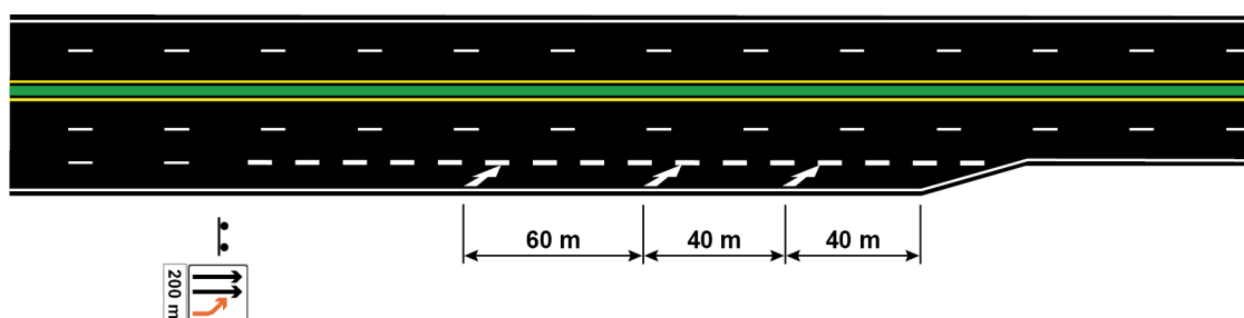
Figur 5.7—1 — Oppmerking av kjørefeltavslutning utenfor vegkryss
