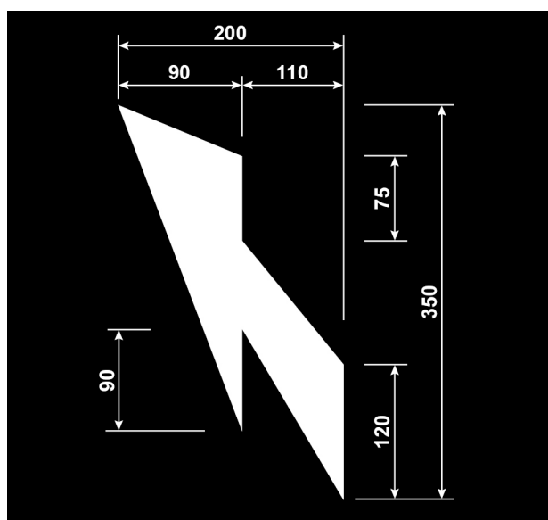
Figur 3.4—3 — Utforming og dimensjoner for 1034.F piler for feltskifte (mål i cm)
