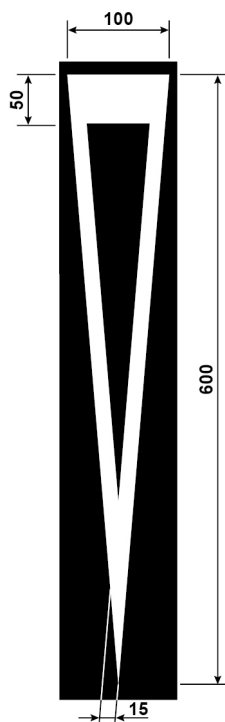
Figur 3.5—1 — Utforming av vikesymbol
