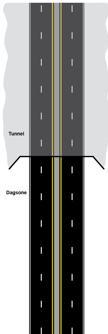
Figur 5.9—2 — Oppmerking i 2-løps tunnel
