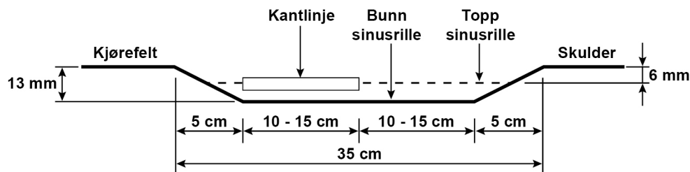
Figur 6.3.2—1 — Utforming av fresepor med 0,35 m bredde
