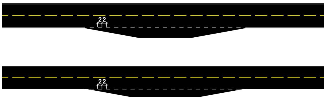
Figur 9.1—1 — Oppmerking av busslomme
