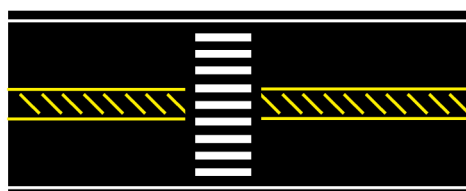
Figur 8.1—2 — Gangfelt ved trafikkøy og sperreområde
