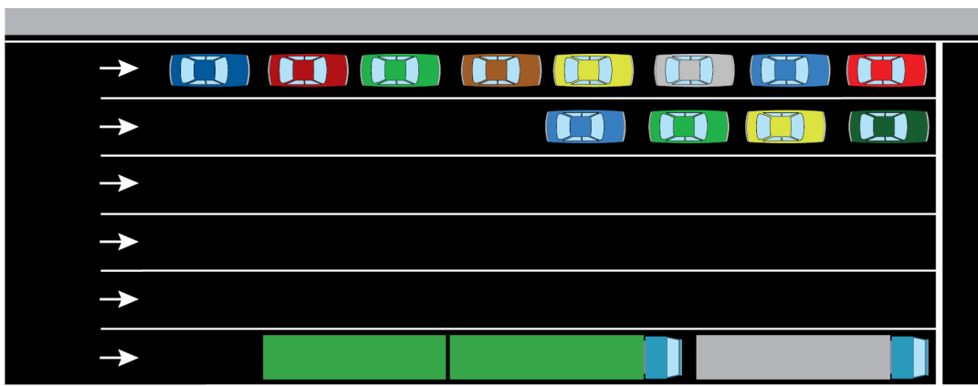
Figur 10.5—1 — Eksempel på oppmerking på ferjekaier
