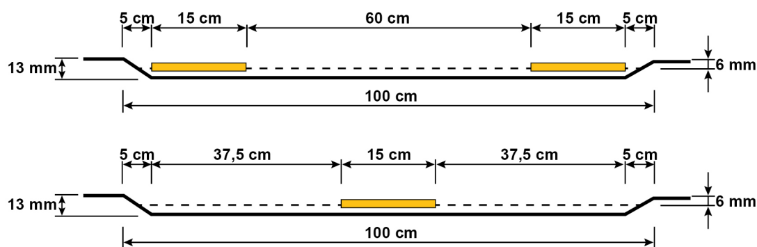
Figur 6.3.1—3 — Utforming av fresespor med 1 m bredde med henholdsvis dobbel sperrelinje og varsellinje/kjørefeltlinje
