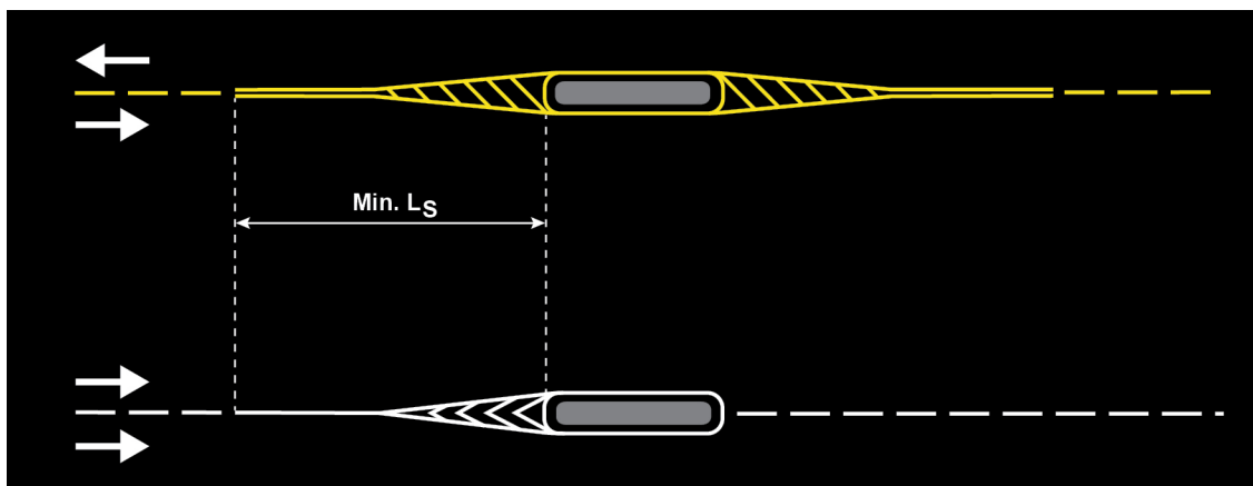
Figur 5.8.2—1 — Oppmerking foran hindringer i vegbanen (fartsgrense \geq 60 km/t)
