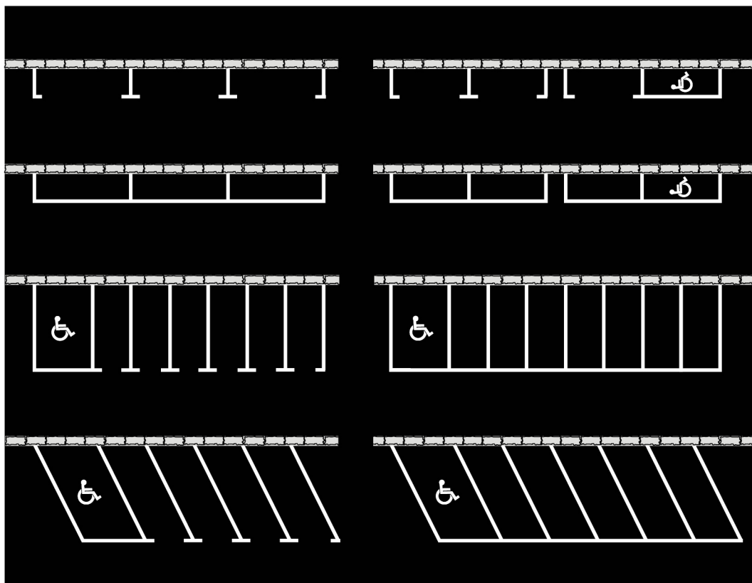
Figur 10.4—1 — Eksempler på parkeringsoppmerking
