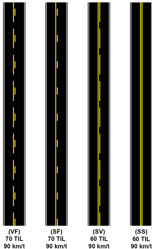
Figur 5.3.2—4 — Kombinert linje
