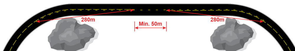
Figur 4.3—1 — Kjørefeltlinje mellom kombinasjonslinjer
