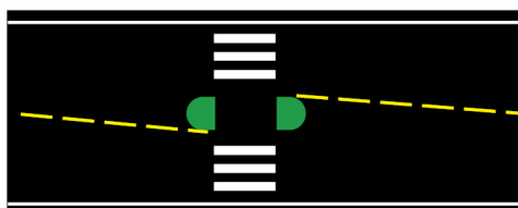
Figur 8.1—2 — Gangfelt ved trafikkøy og sperreområde
