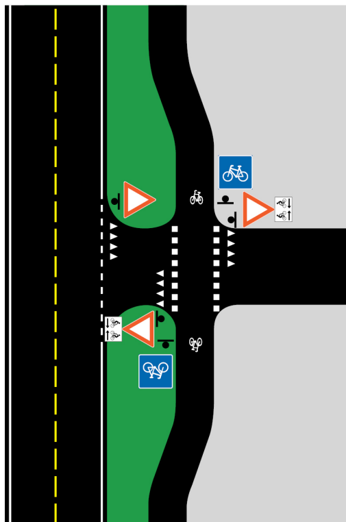
Figur 8.8—2 — Oppmerking når kjørende på sekundærveg har vikeplikt for syklende
