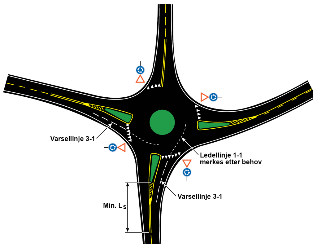
Figur 7.4—1 — Oppmerking av rundkjøring på 2-feltsveg
