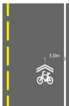
Figur 8.11—2 — Plassering av 1038 delesymbol
