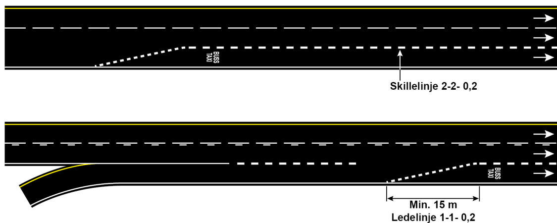
Figur 9.4.1—1 — Oppmerking ved starten på kollektivfelt
