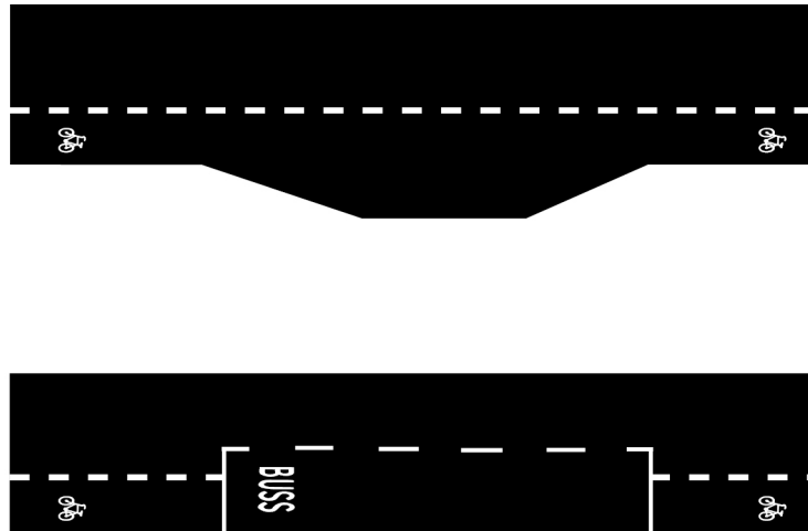
Figur 8.2—3 — Oppmerking av sykkelfelt ved busslomme og kantstopp for buss
