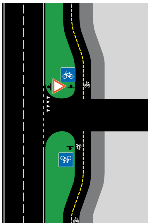
Figur 8.7—1 — Oppmerking når kjørende på sekundærvegen ikke har vikeplikt for syklende og gående (trafikkreglene § 7 nr. 4 annet ledd og § 19 nr. 2 annet ledd)
