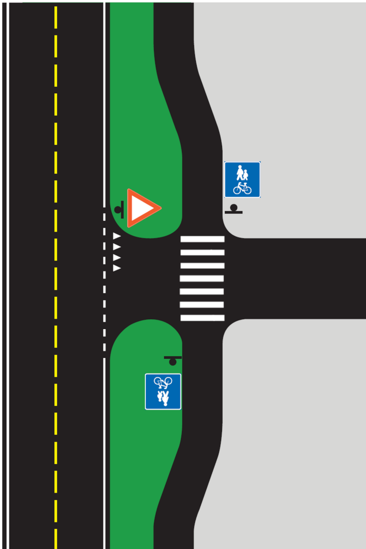
Figur 8.6—2 — Oppmerking når gang og sykkelveg krysser sekundærvæg med gangfelt
