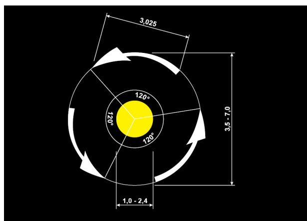
Figur 3.4—4 — Utforming og dimensjoner for piler i minirundkjøring (mål i m)
