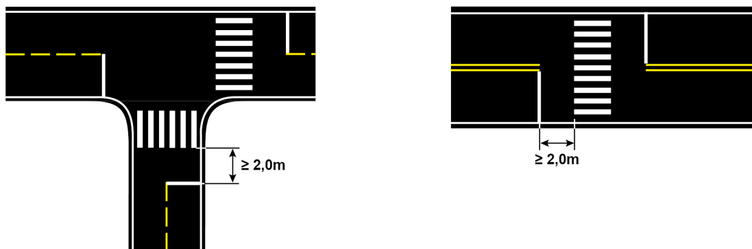
Figur 8.1—4 — Gangfelt ved signalregulering
