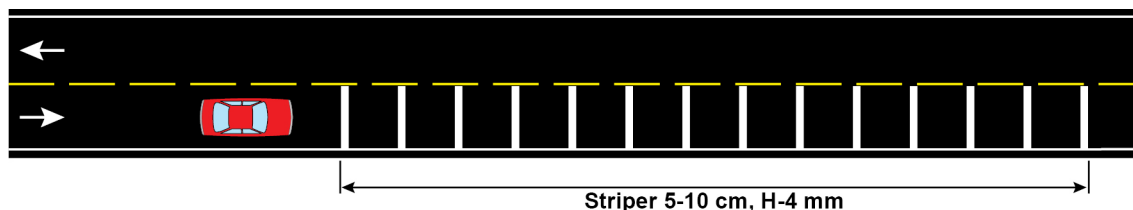
Figur 10.3—1 — Oppmerking av rumlefelt
