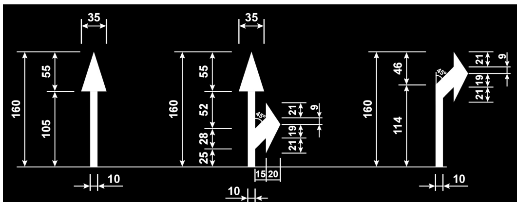
Figur 3.4—2 — Utforming og dimensjoner for piler for sykkeltrafikk (mål i cm)
