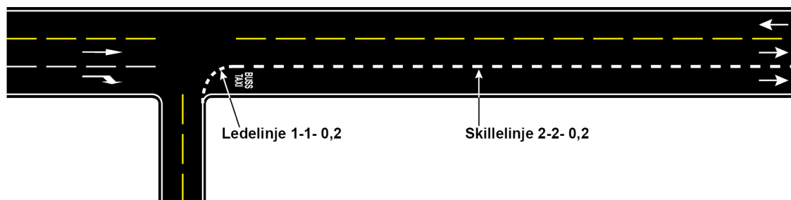
Figur 9.4.2—1 — Oppmerking av start på kollektivfelt i kryss
