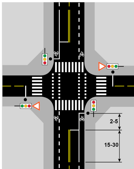
Figur 8.4—3 — Signalregulert kryss på forkjørsveg med tilbaketrukket stopplinje uten sykkelboks
