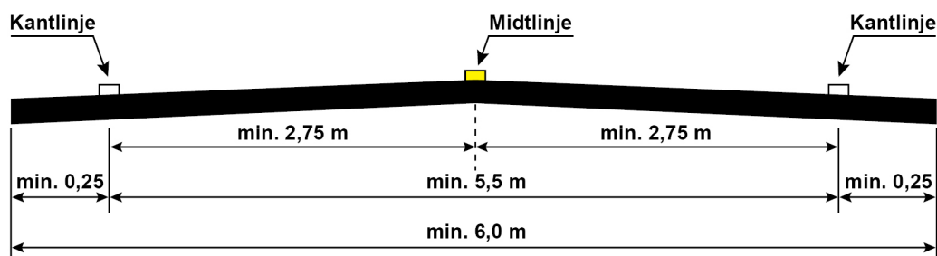
Figur 5.3—1 — Minste breddekrav for oppmerking av midtlinje
