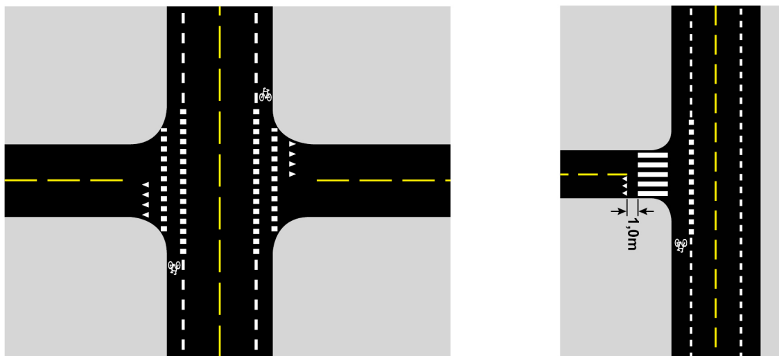
Figur 8.3—2 — Oppmerking av sykkelfelt og sykkelkryssing på forkjørsveg
