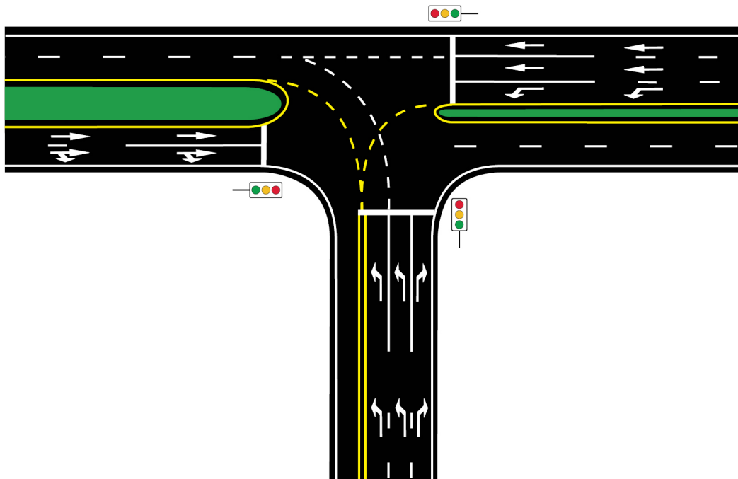
Figur 7.5—2 — Bruk av ledelinjer i signalregulert kryss
