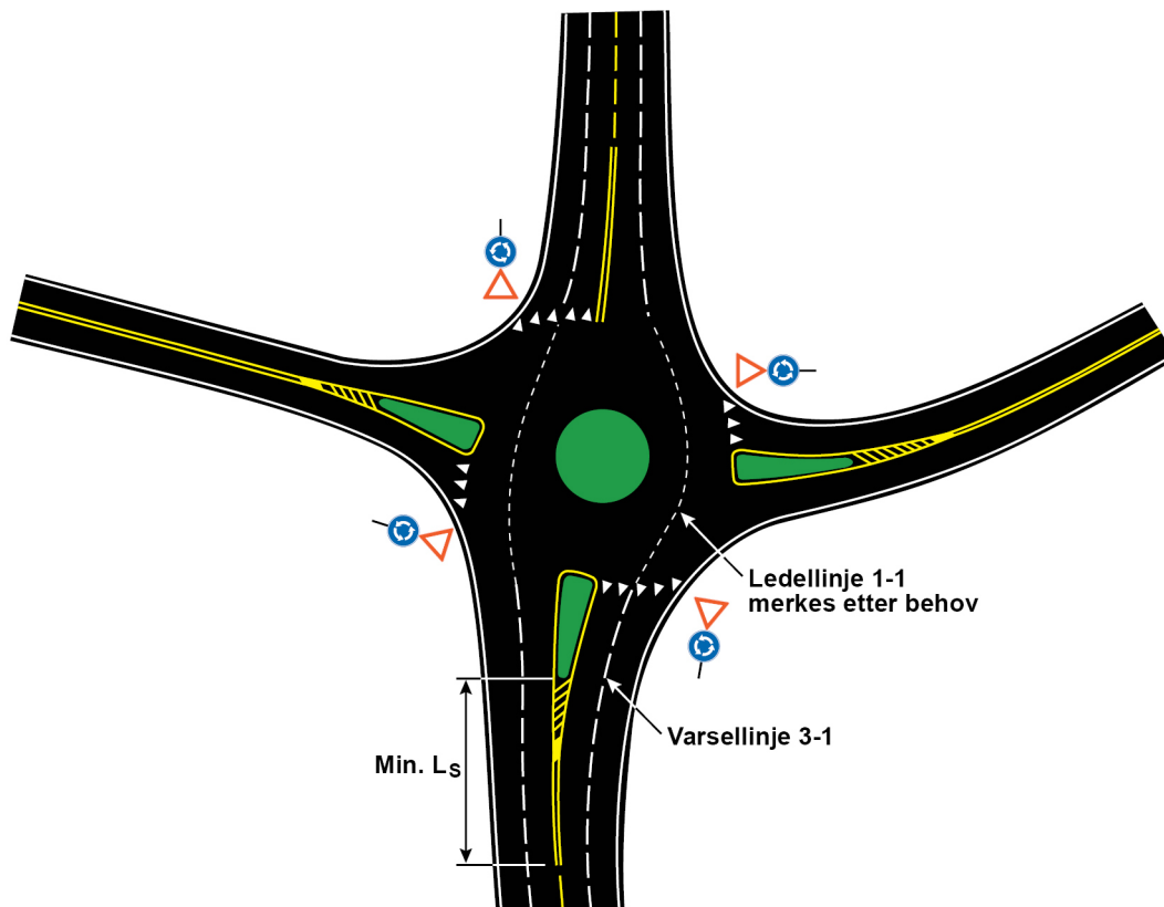
Figur 7.4—2 — Oppmerking av rundkjøring på 4-feltsveg
