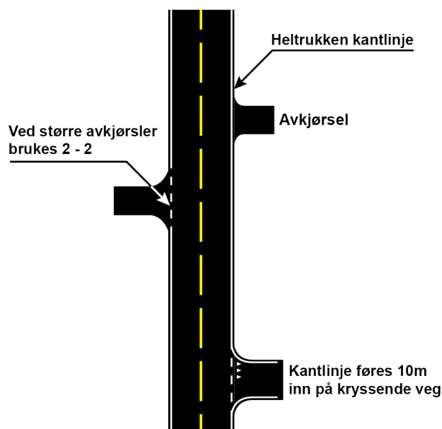
Figur 5.3.2—1 — Anvendelse av kantlinjer på 2-feltsveg
