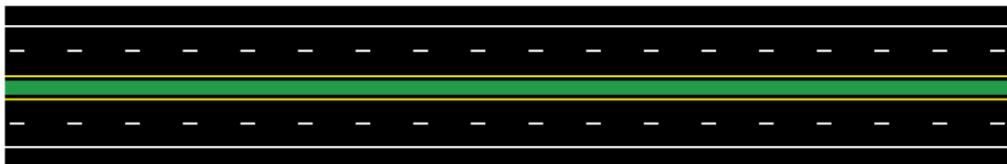
Figur 5.5—3 — Oppmerking på 4-feltsveg
