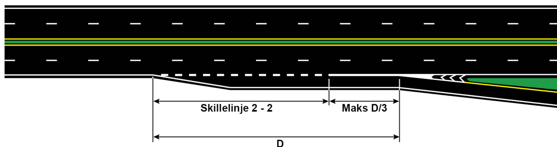
Figur 7.6.3—1 — Oppmerking av retardasjonsfelt
