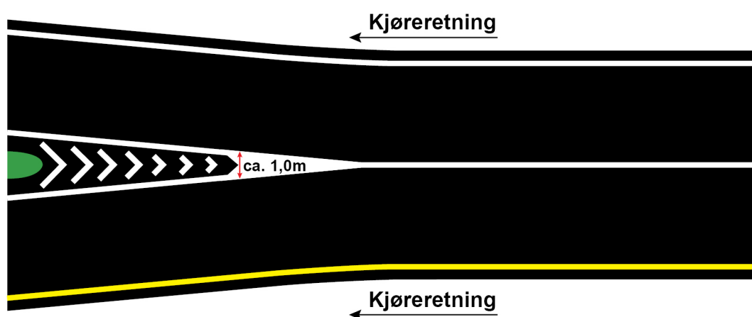
Figur 3.2—1 — Utforming og dimensjoner for sperreområde mellom trafikk i samme kjøreretning
