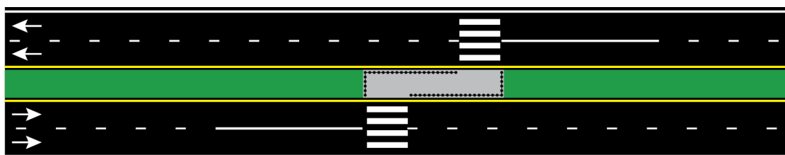
Figur 8.1—7 — Delelinje foran gangfelt på 4-feltsveg ved fartsgrense \leq 60 km/t
