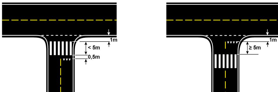
Figur 8.1—3 — Gangfelt over vikepliktig sideveg
