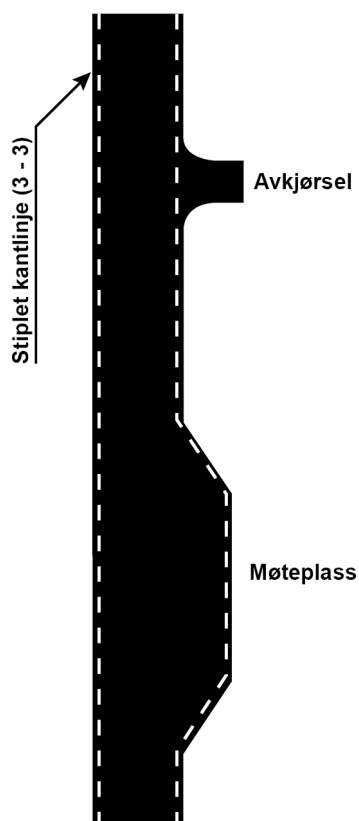
Figur 5.3.1—1 — Anvendelse av kantlinjer på 1-feltsveg
