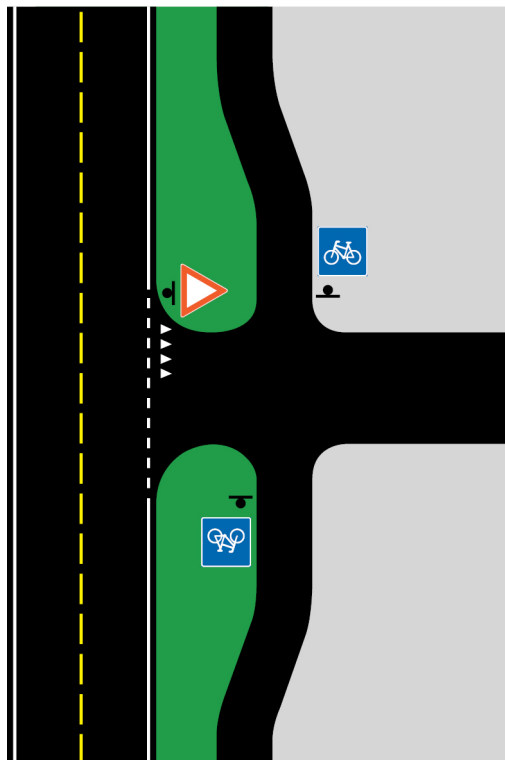
Figur 8.8—1 — Oppmerking når kjørende på sekundærveg ikke har vikeplikt for syklende (trafikkreglene § 7 nr. 4 annet ledd)
