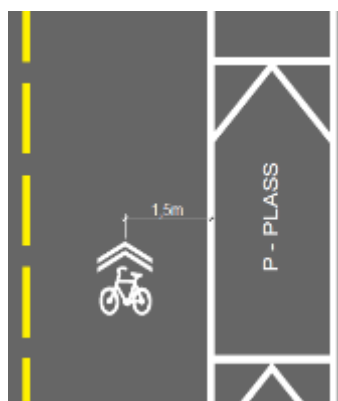
Figur 8.11—3 — Plassering av 1038 delesymbol ved langsgående gateparkering
