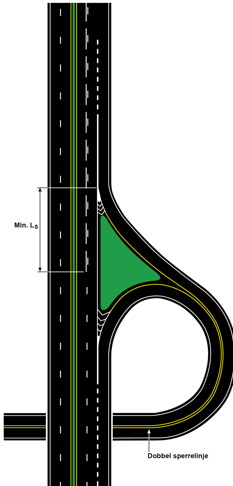
Figur 7.6.9—1 — Oppmerking av rampe med tovegstrafikk
