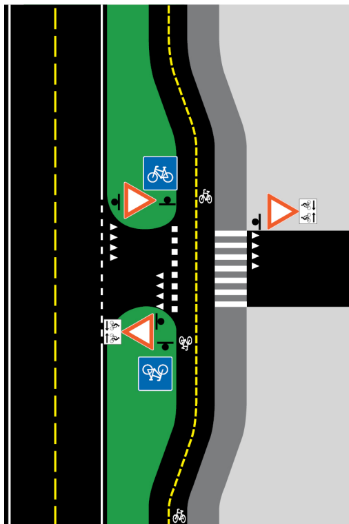
Figur 8.7—2 — Oppmerking når kjørende på sekundærvegen har vikeplikt for syklende og gående
