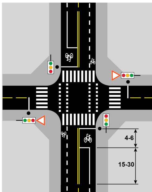
Figur 8.4—1 — Sykkelboks i signalregulert kryss - forkjørsveg
