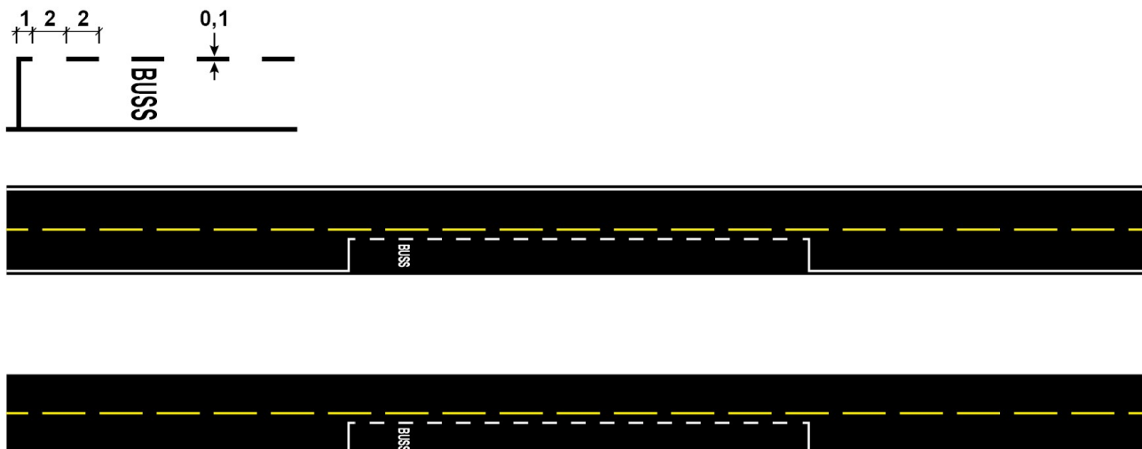
Figur 9.2—1 — Oppmerking av kantstopp
