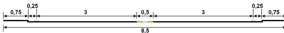
Figur 6.3.3—3 — Forsterket midtoppmerking i tunnel for tunnelprofil T8,5 (mål i m)
