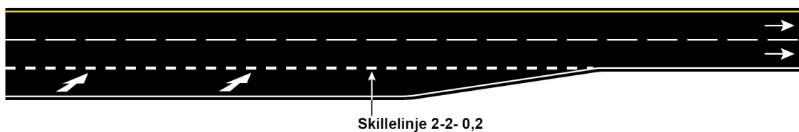
Figur 9.4.3—1 — Avslutning av kollektivfelt på vegstrekning
