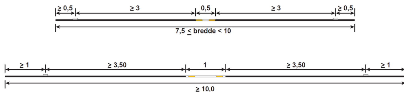
Figur 6.3.1—1 — Tverrprofil ved forsterket vegoppmerking (mål i m)
