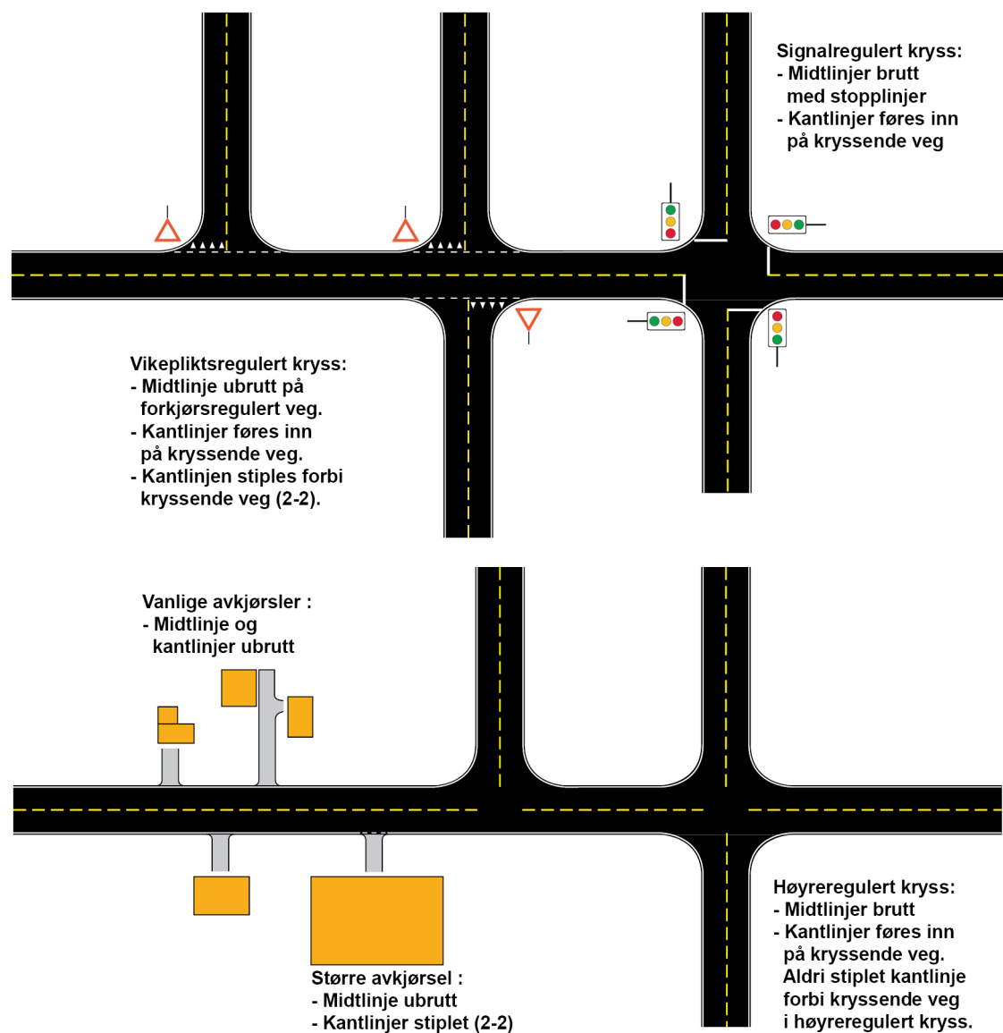
Figur 7.1—1 — Langsgående oppmerking i kryss og avkjørsler
