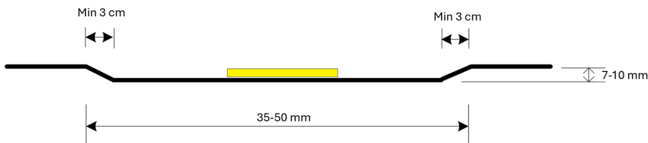
Figur 6.2—1 — Eksempel på utforming av fresespor
