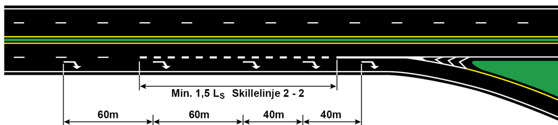
Figur 7.6.4—1 — Eksempel på oppmerking av feltsubtraksjon
