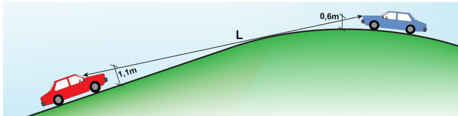
Figur 4.2—1 — Siktkontroll i vertikalkurvatur
