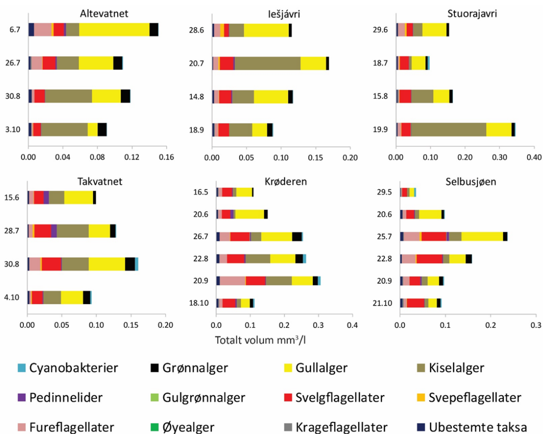
Figur F.2. Kvantitativ fordeling av planteplanktonklasser oppgitt som totalt volum \text{mm}^3/\text{l} ( \approx \text{mg/l} ) gjennom vekstsesongen i alle innsjøene i ØKOSTOR 2022. Merk ulik skala på x-aksen.
