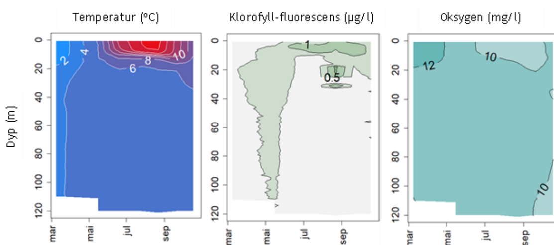
Figur 3. Vertikalprofiler av temperatur (venstre), klorofyll fluorescens (midten) og oksygen (høyre) i hele vannsøylen (0-130 m) på den pelagiske stasjonen over dypeste punkt i Krøderen fra mai til oktober 2022. I Vedlegg D er tilsvarende figurer vist for dyp 0-50 m.
