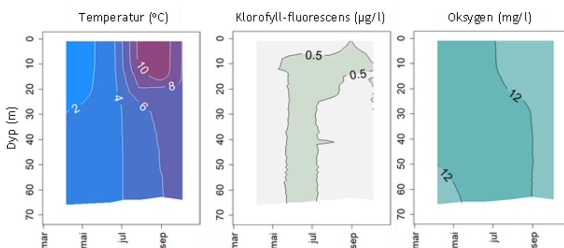
Figur 8. Vertikalprofiler av temperatur (venstre) og klorofyll fluorescens (µg/l, midten) og oksygen (høyre) målt på den pelagiske stasjonen over dypeste punkt i Takvatnet fra april til september 2022.
