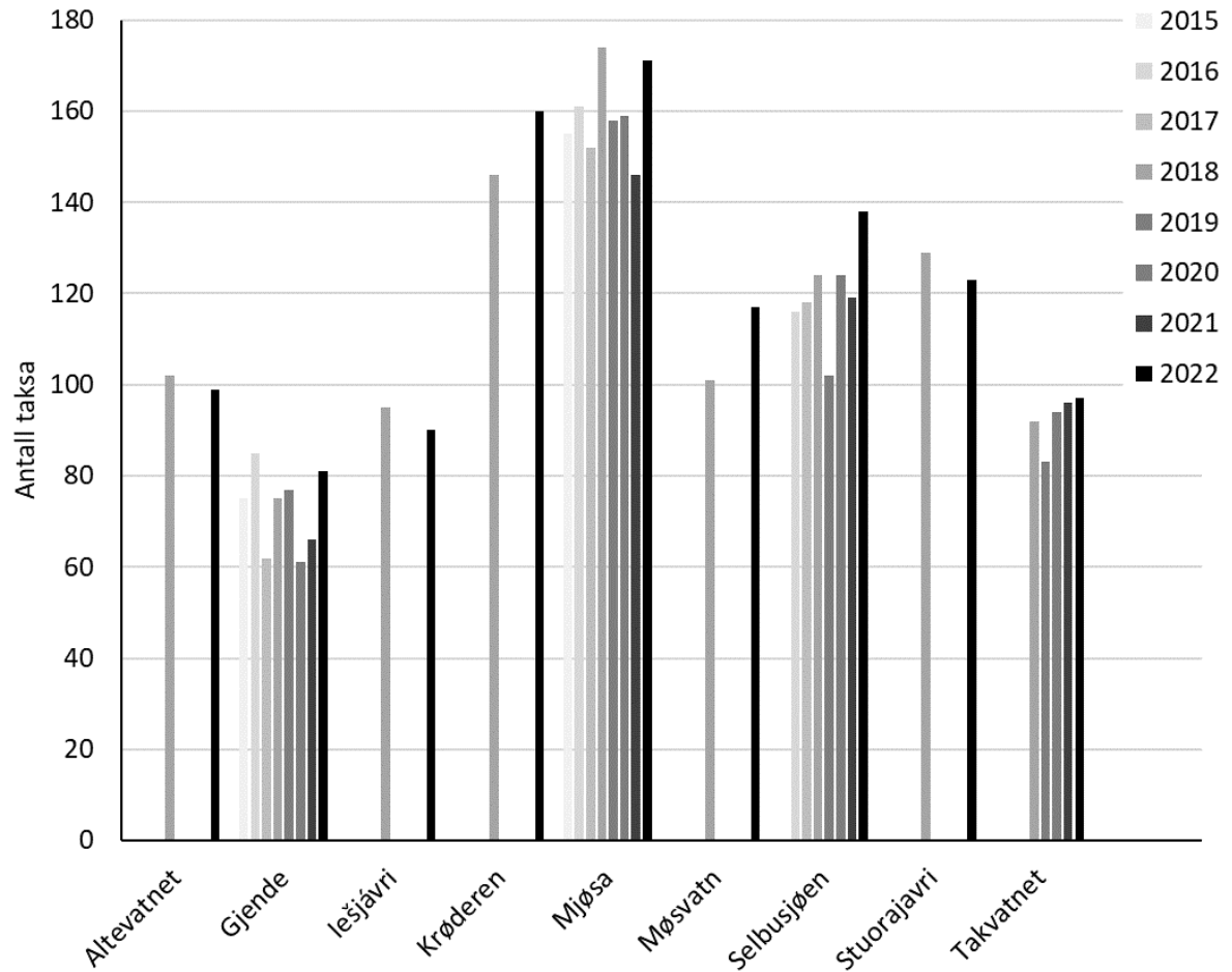
Figur F.1. Antall taksa som ble observert i innsjøene som var med i 2022-overvåkingen de årene de har vært med i ØKOSTOR. Hovedstasjonen i Mjøsa, Skreia, har flere prøver pr år enn de andre innsjøene.
