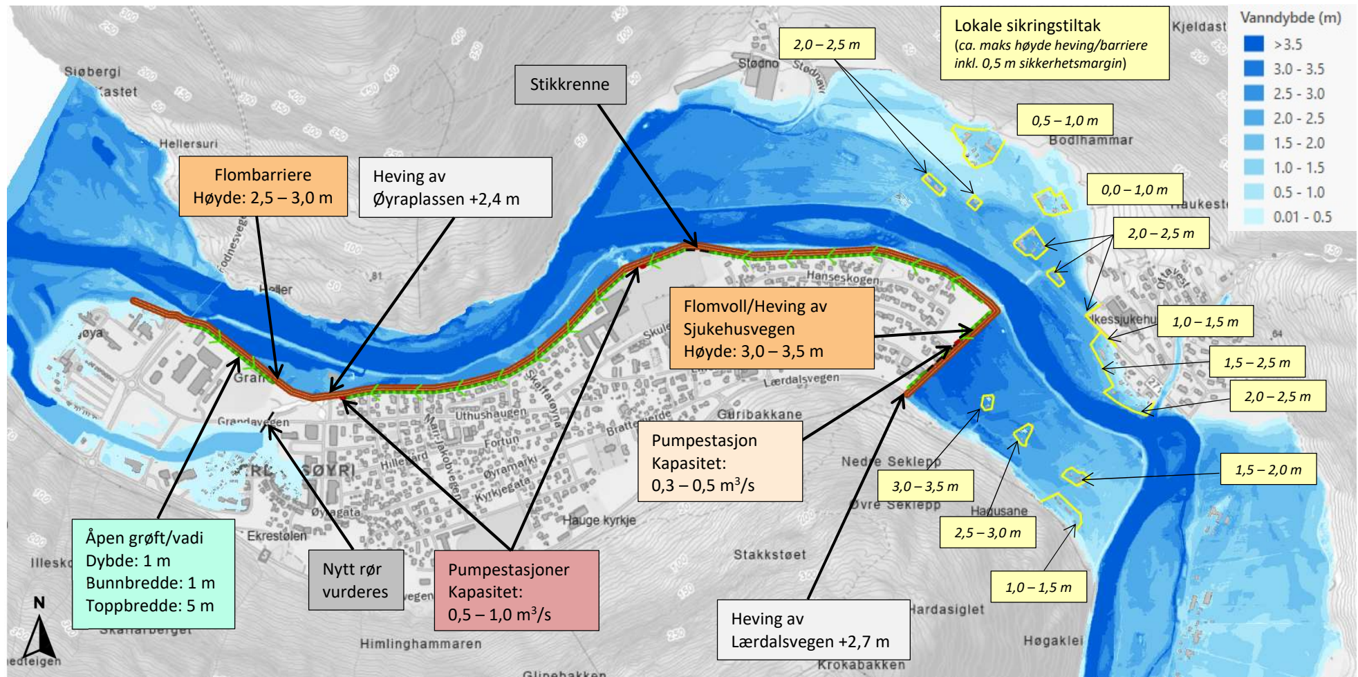
Figur 6-9: Oversiktskart over kombinerte tiltak for å sikre Lærdalsøyri ved en 1000-årsflom med 20% klimapåslag i tiltakskombinasjon 3.
