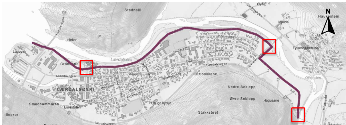
Figur 5-11: Oversikt over flombarrierens kryssinger ved kjøreveier: veien til Lærdal kulturhus (t.v.), Sjukehusvegen (midt) og Lærdalsvegen (t.h.).
