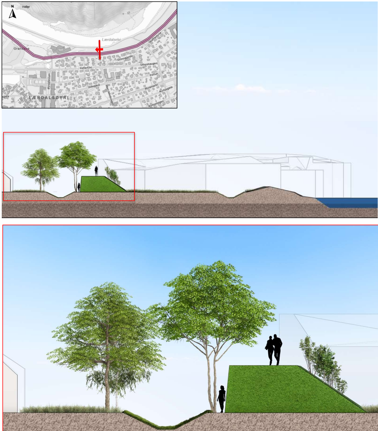
Figur 2-12: Snitt av planlagt flombarriere og grøft i tiltakskombinasjon 2A ved jordbruksarealet oppstrøms Lærdal kulturhus.
