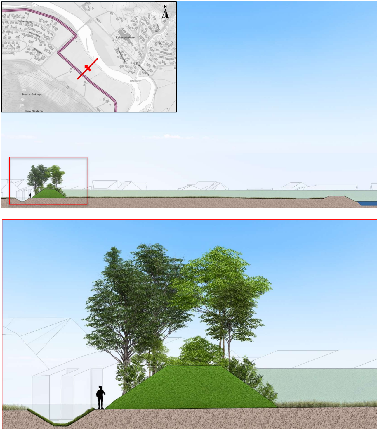
Figur 2-15: Snitt av planlagt flombarriere og grøft i tiltakskombinasjon 2A ved jordbruksarealet oppstrøms Sjukehusvegen.
