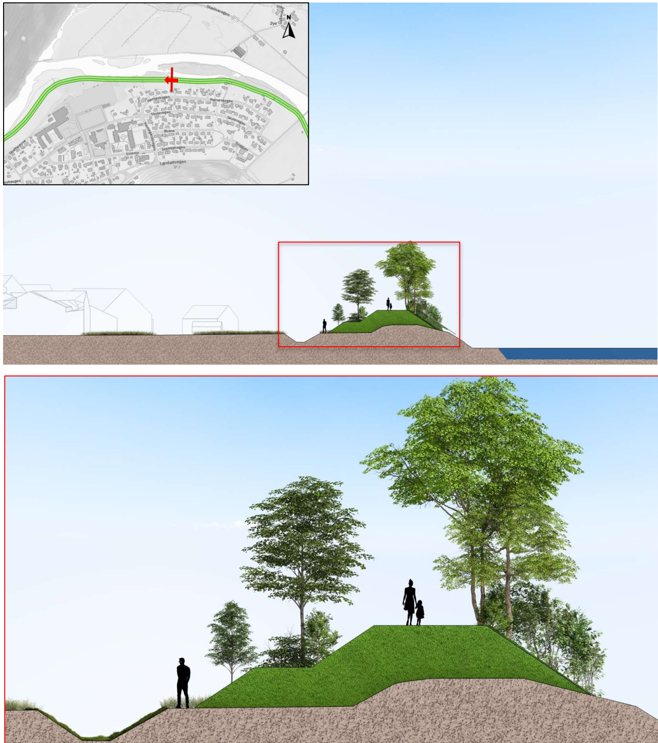
Figur 3-14: Snitt av planlagt flombarriere og grøft i tiltakskombinasjon 2B ved Hanseskogen.
