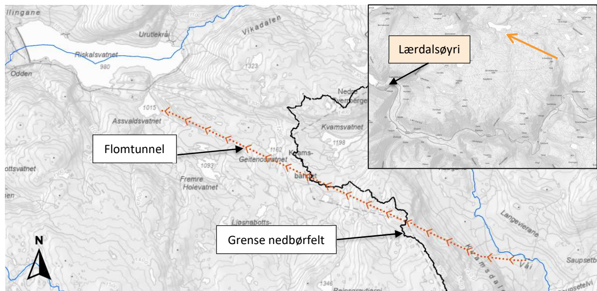
Figur 5-30: Oversiktskart som viser foreslått trase til tunnelen fra Kvemma til nabovassdraget.
