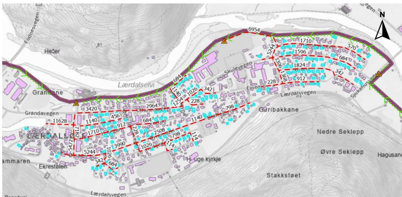
Figur 2-5: Vurdering av nytt dreneringssystem ved 3 meter grunnvannssenkning. Røde linjer viser plassering til de nye ledningene og tallene viser dimensjonerende vannmengde i l/s. Med lyseblå vises bygninger med kjeller.
