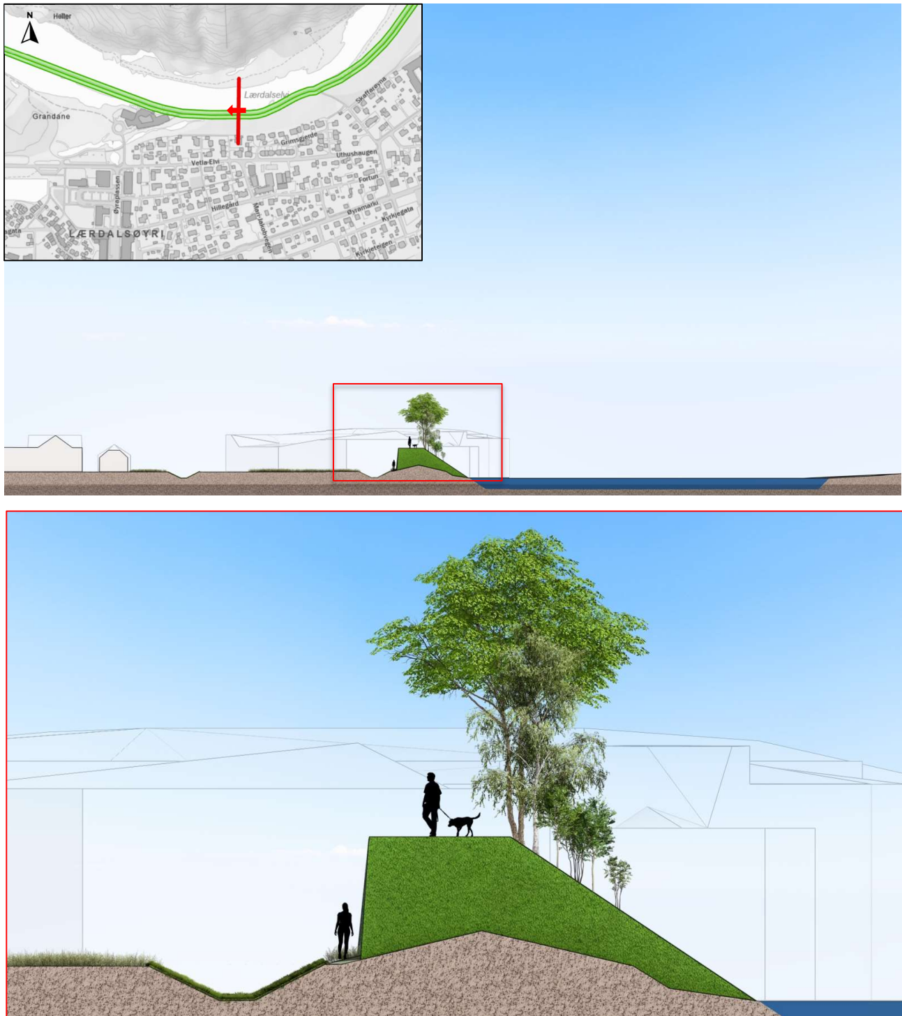
Figur 3-12: Snitt av planlagt flombarriere og grøft i tiltakskombinasjon 2B ved jordbruksarealet oppstrøms Lærdal kulturhus.
