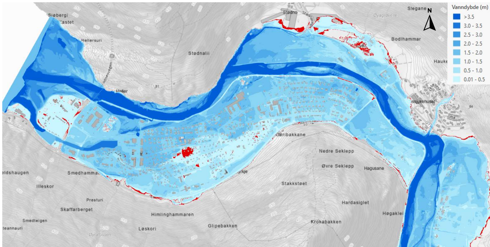
Figur 6-1: Flomsonekart ved en 200-årsflom med 20% klimapåslag i tiltakskombinasjon 0. Røde områder viser ytterligere oversvømt areal ved en 1000-årsflom med 20% klimapåslag.
