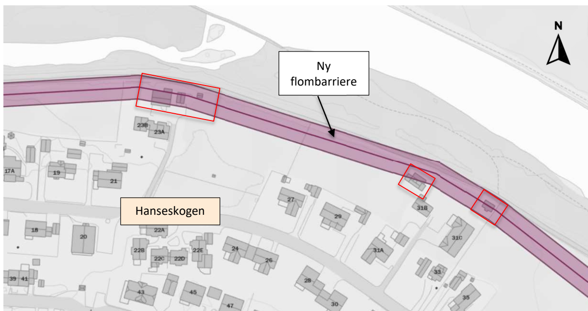
Figur 5-12: Oversikt over bygninger som må rives ved etablering av tiltak 2A.
