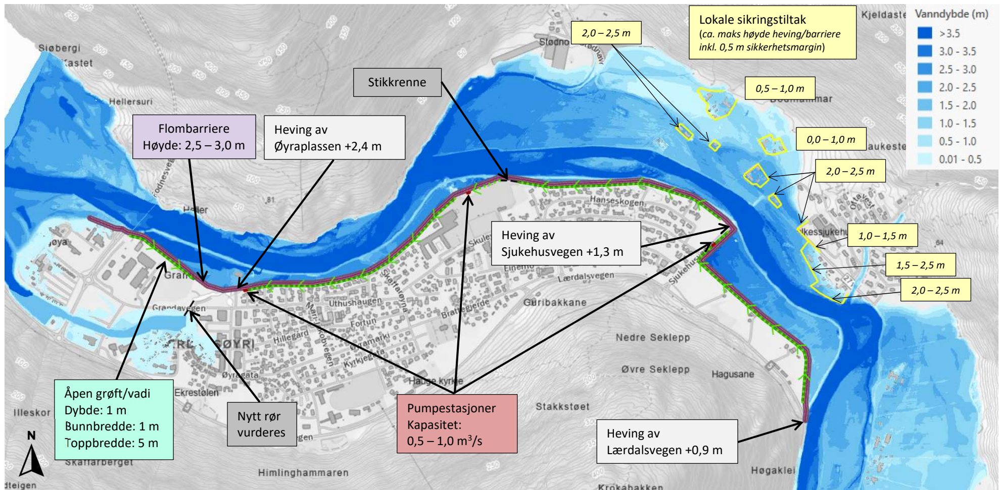
Figur 6-5: Oversiktskart over kombinerte tiltak for å sikre Lærdalsøyri ved en 1000-årsflom med 20% klimapåslag i tiltakskombinasjon 2A.
