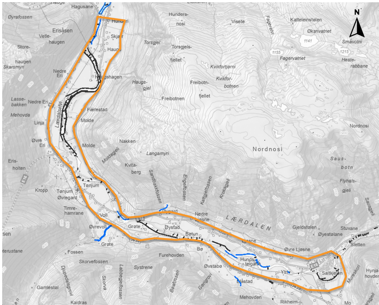
Figur 5-31: Oversiktskart over tiltakets påvirkningsområde. Blåe og svarte linjer viser eksisterende sikringstiltak.
