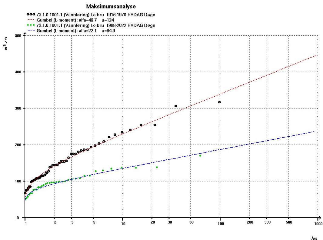
Figur 3-10: Flomfrekvensanalyse for flom ved Lo bru før og etter vassdraget ble utbygget.
