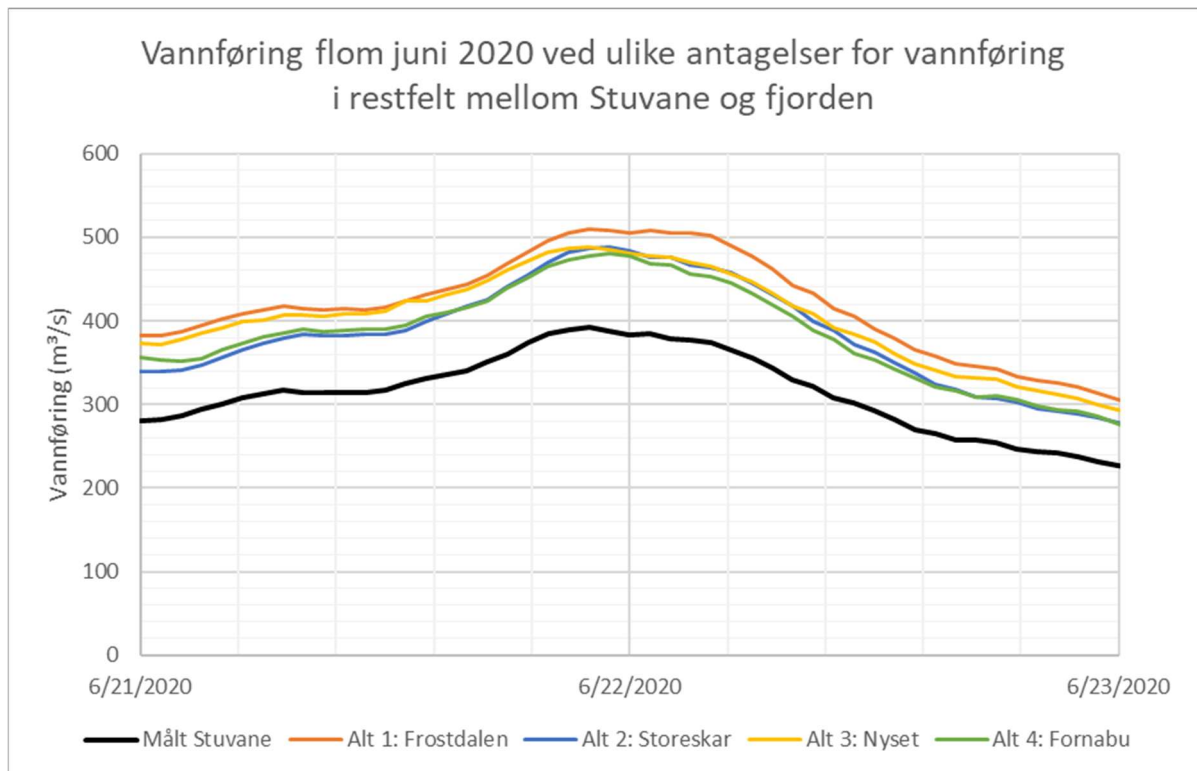
Figur 2-11: Estimert vannføring ved Lærdalsøyri (fargede linjer) ved flommen i 2020.
