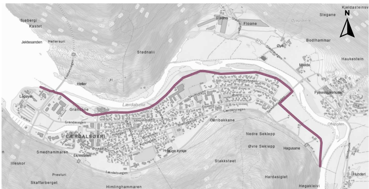
Figur 5-8: Oversiktskart som viser plassering og trase til flombarrieren i alternativ A.
