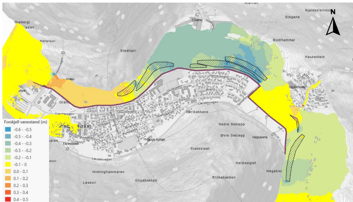
Figur 6-15: Sammenligning av flomvannstand ved en klimajustert 1000-årsflom: tiltakskombinasjon 6 minus tiltakskombinasjon 2A. Negative verdier indikerer lavere flomvannstand i tiltakskombinasjon 6 sammenlignet med tiltakskombinasjon 2A. Svarte polygoner viser hvor masseuttaket er utført.
