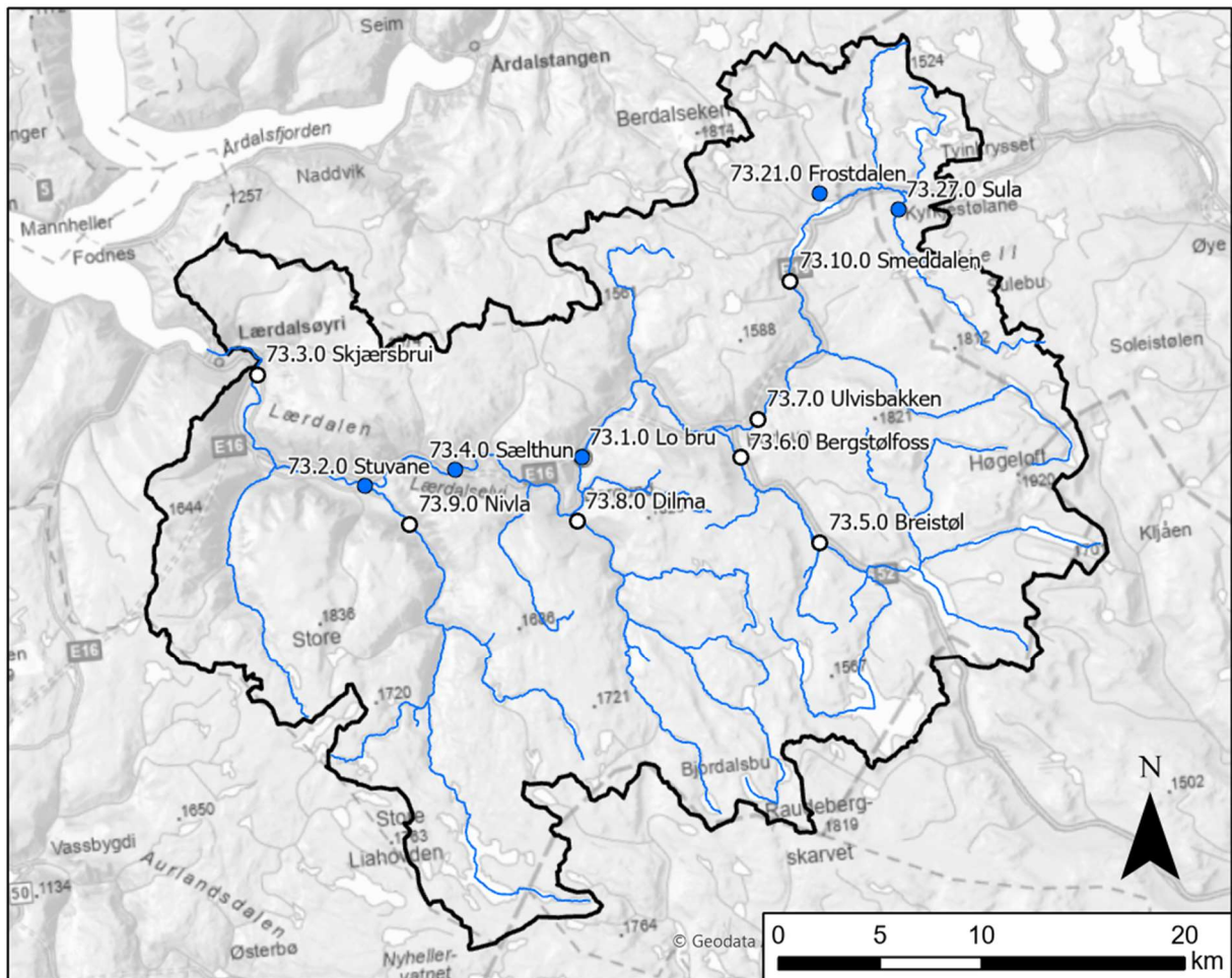
Figur 4-1: Kart over målestasjoner i Lærdalsvassdraget. Blå er aktive stasjoner og hvite er nedlagt.
