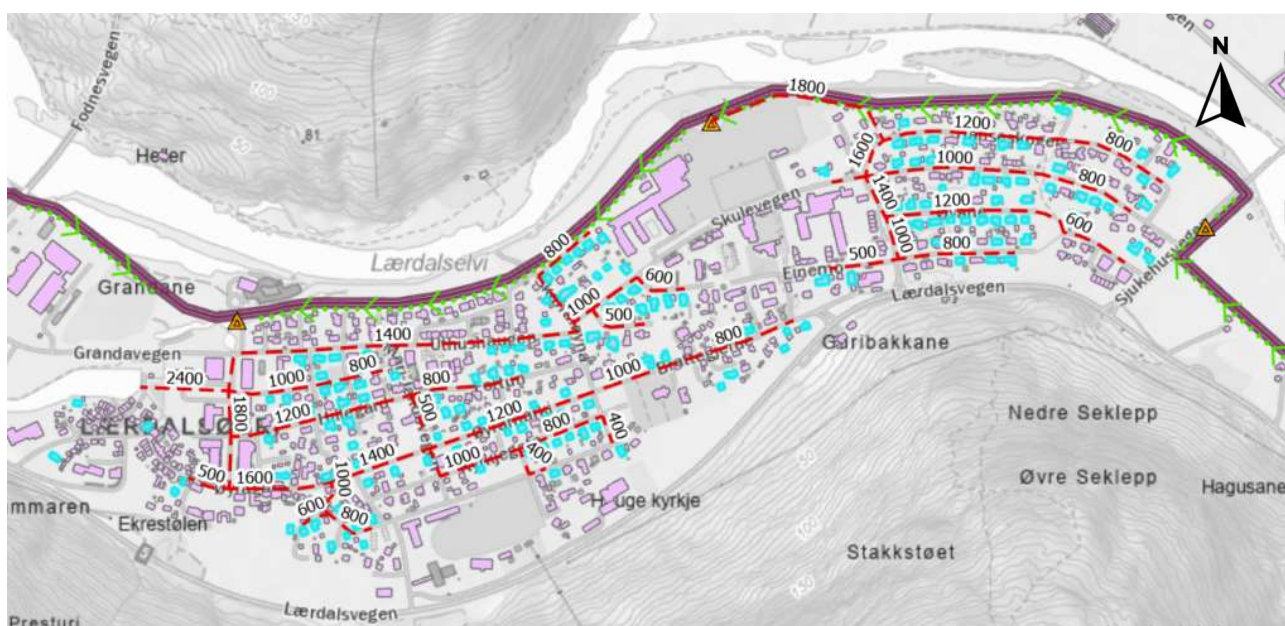
Figur 2-6: Vurdering av nytt dreneringssystem ved 1 meter grunnvannssenkning. Røde linjer viser plassering til de nye ledningene og tallene viser nødvendig diameter i mm. Med lyseblå vises bygninger med kjeller.
