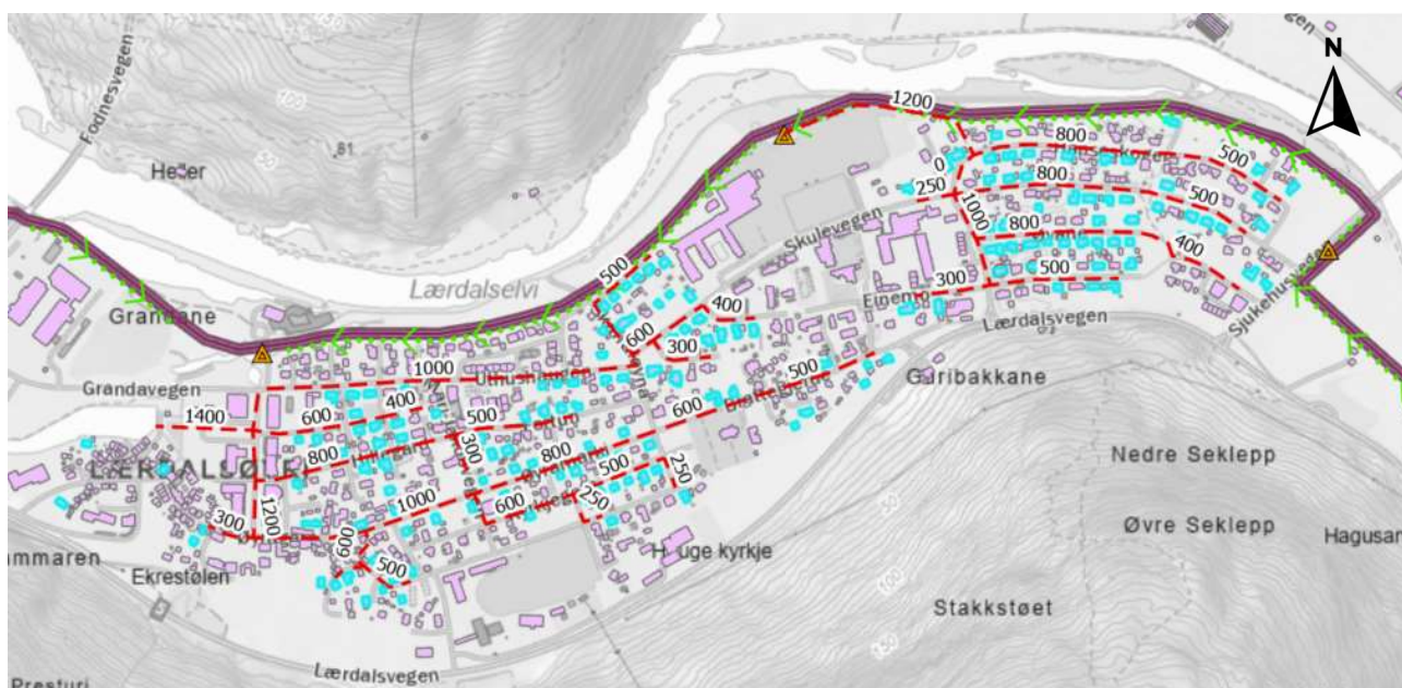
Figur 2-4: Vurdering av nytt dreneringssystem ved 1 meter grunnvannssenkning. Røde linjer viser plassering til de nye ledningene og tallene viser nødvendig diameter i mm. Med lyseblå vises bygninger med kjeller.
