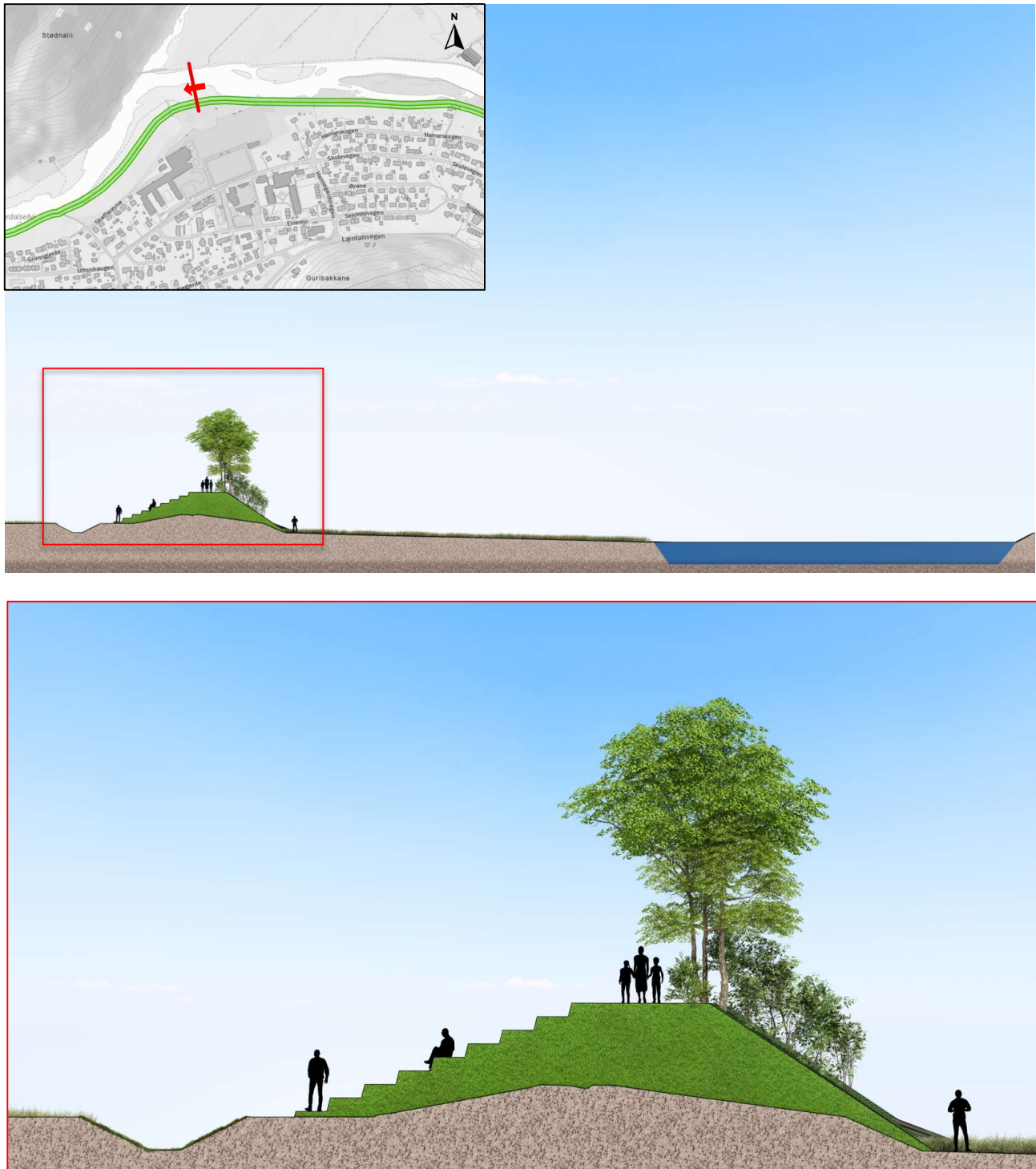
Figur 3-13: Snitt av planlagt flombarriere og grøft i tiltakskombinasjon 2B ved Lærdalshallen.
