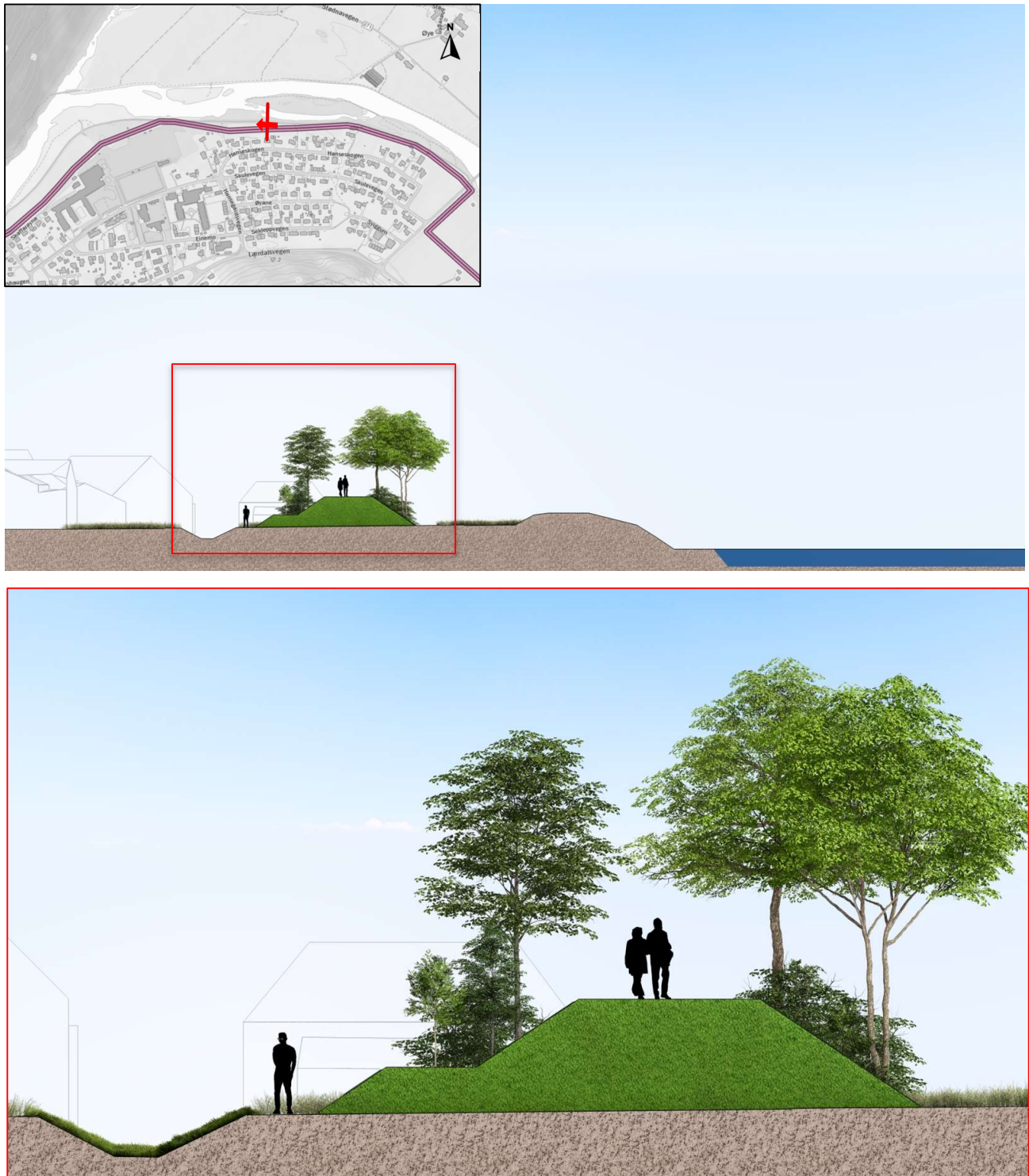
Figur 2-14: Snitt av planlagt flombarriere og grøft i tiltakskombinasjon 2A ved Hanseskogen.
