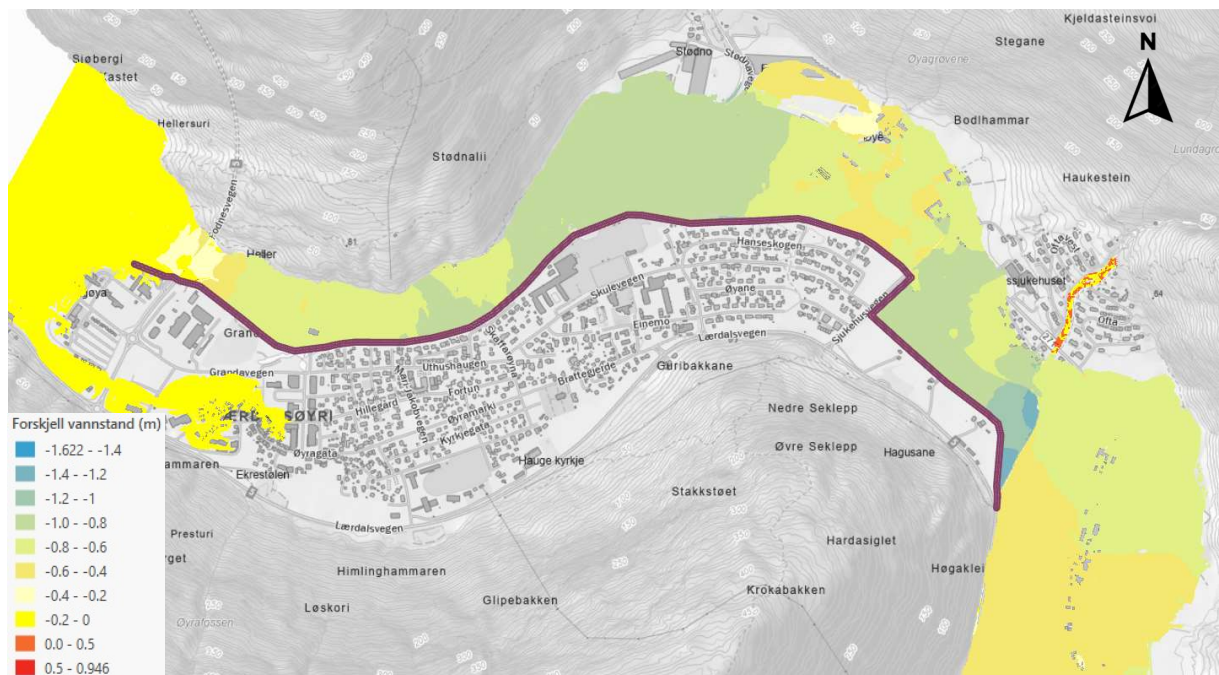
Figur 6-11: Sammenligning av flomvannstand ved en klimajustert 1000-årsflom: tiltakskombinasjon 4 minus tiltakskombinasjon 2A. Negative verdier indikerer en lavere flomvannstand i tiltakskombinasjon 4 sammenlignet med tiltakskombinasjon 2A.
