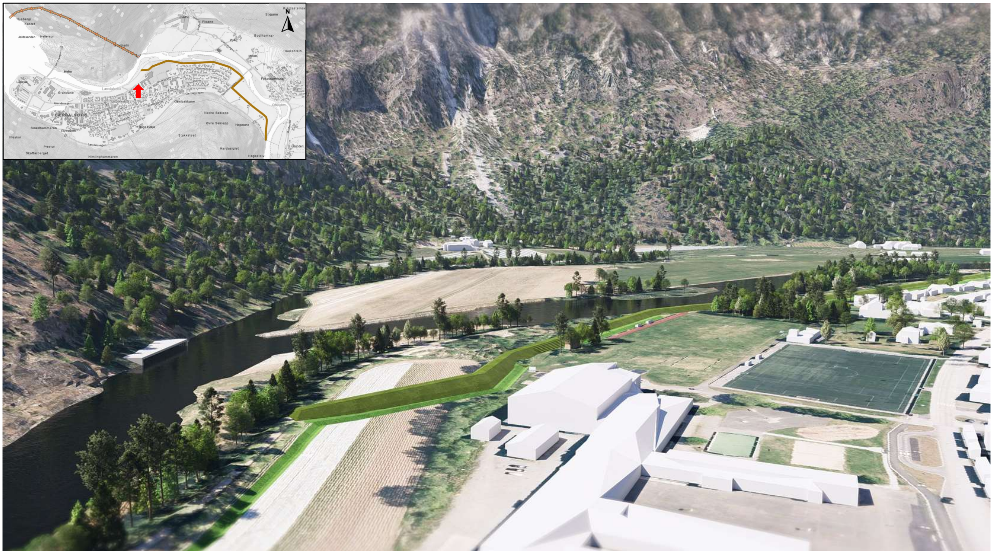
Figur 4-8: 3D-illustrasjon av planlagte flombarrierer, grøfter, pumpestasjoner og inntaksarrangement til flomtunnel ved Lærdalshallen i tiltakskombinasjon 5 sett fra sør.
