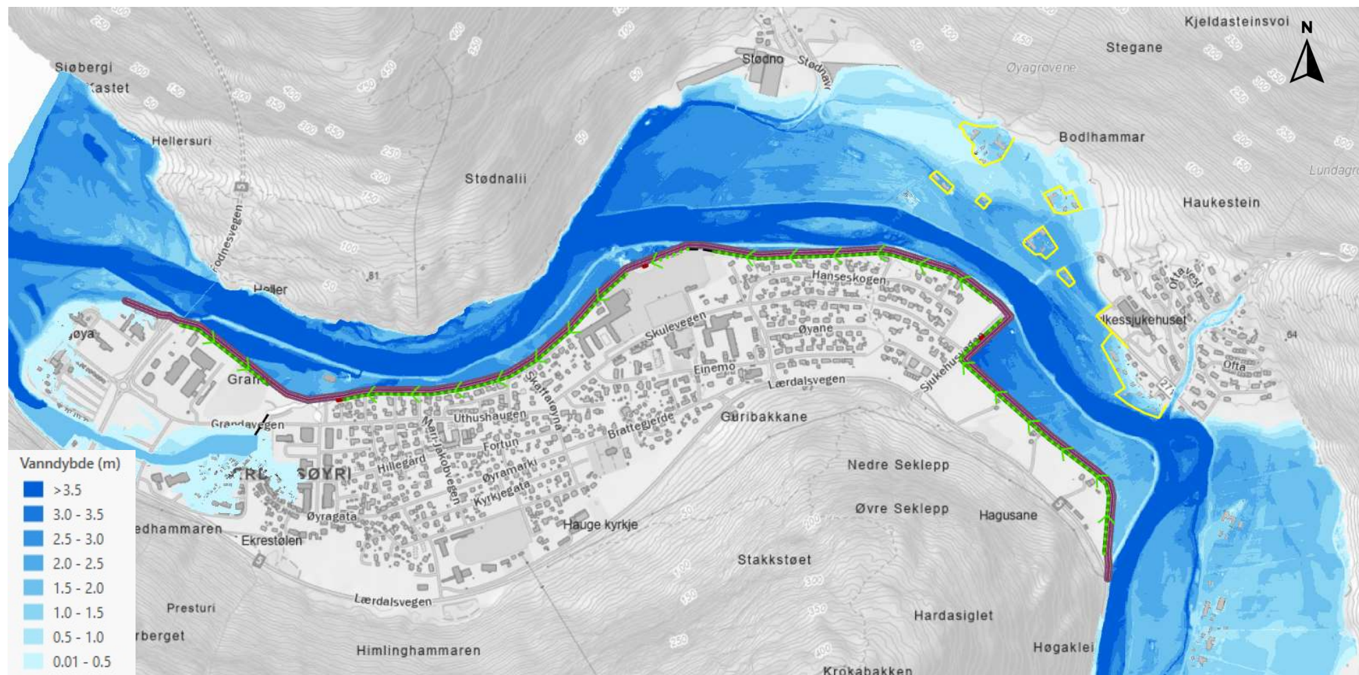
Figur 2-1: Oversiktskart over tiltakskombinasjon 2A. Se Figur 6-5 i hovedrapporten for flere detaljer om tiltakene.
