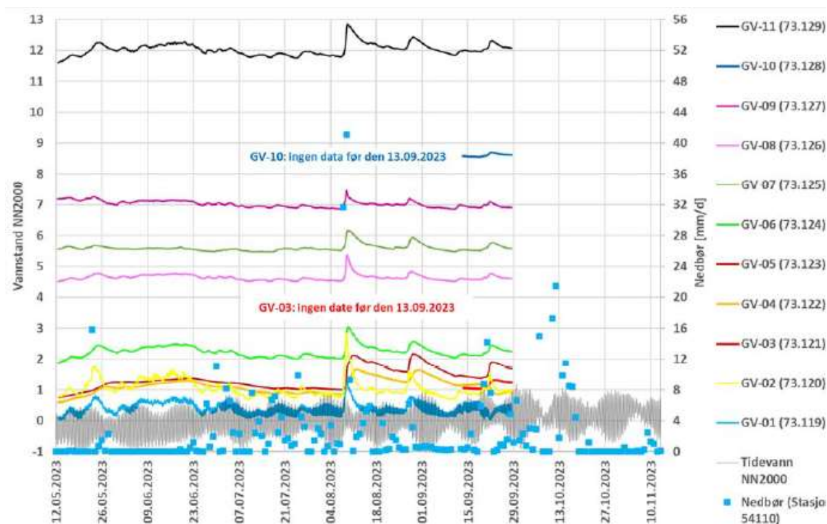
Figur 2-5: Tidsserier for grunnvannstand, tidevann og nedbør i perioden 12.05.2023 til 10.11.2023 (Dr. Blasy og Dr. Øverland, 2024).
