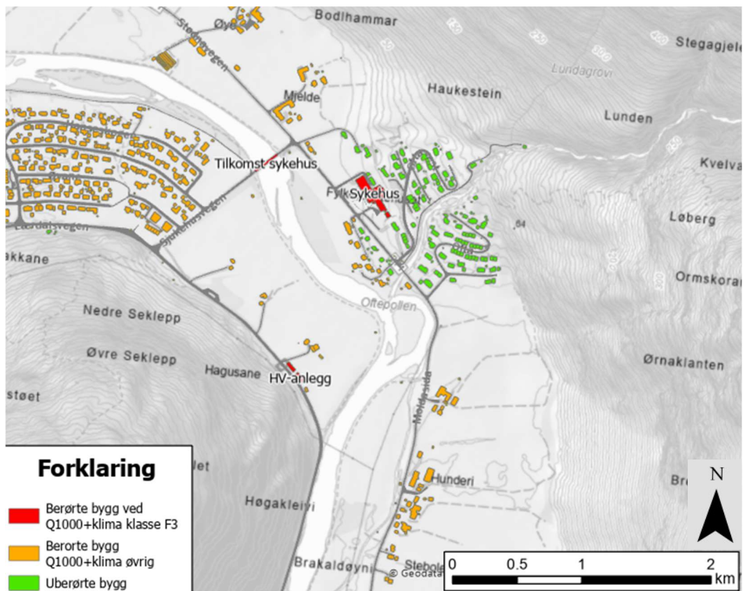
Figur 2-10: Kritiske objekt (sikkerhetsklasse F3) berørt ved 1000-årsflom inkl. klimapåslag i Lærdalsøyri (oppstrøms del).
