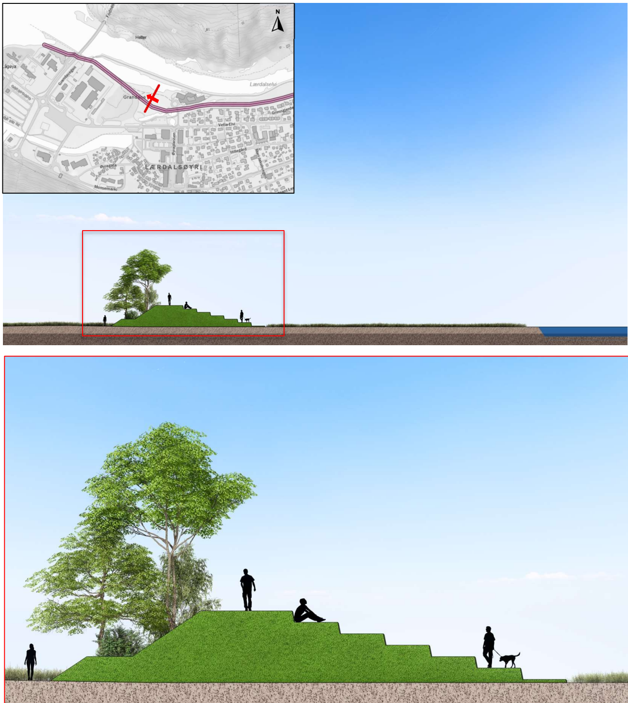
Figur 2-11: Snitt av planlagt flombarriere i tiltakskombinasjon 2A ved Grandane.
