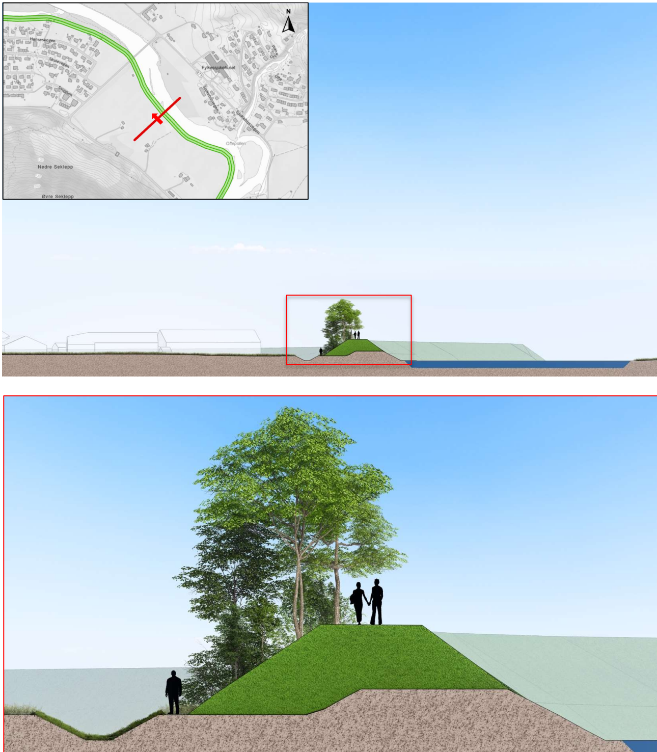
Figur 3-15: Snitt av planlagt flombarriere og grøft i tiltakskombinasjon 2B ved jordbruksarealet oppstrøms Sjukehusvegen.
