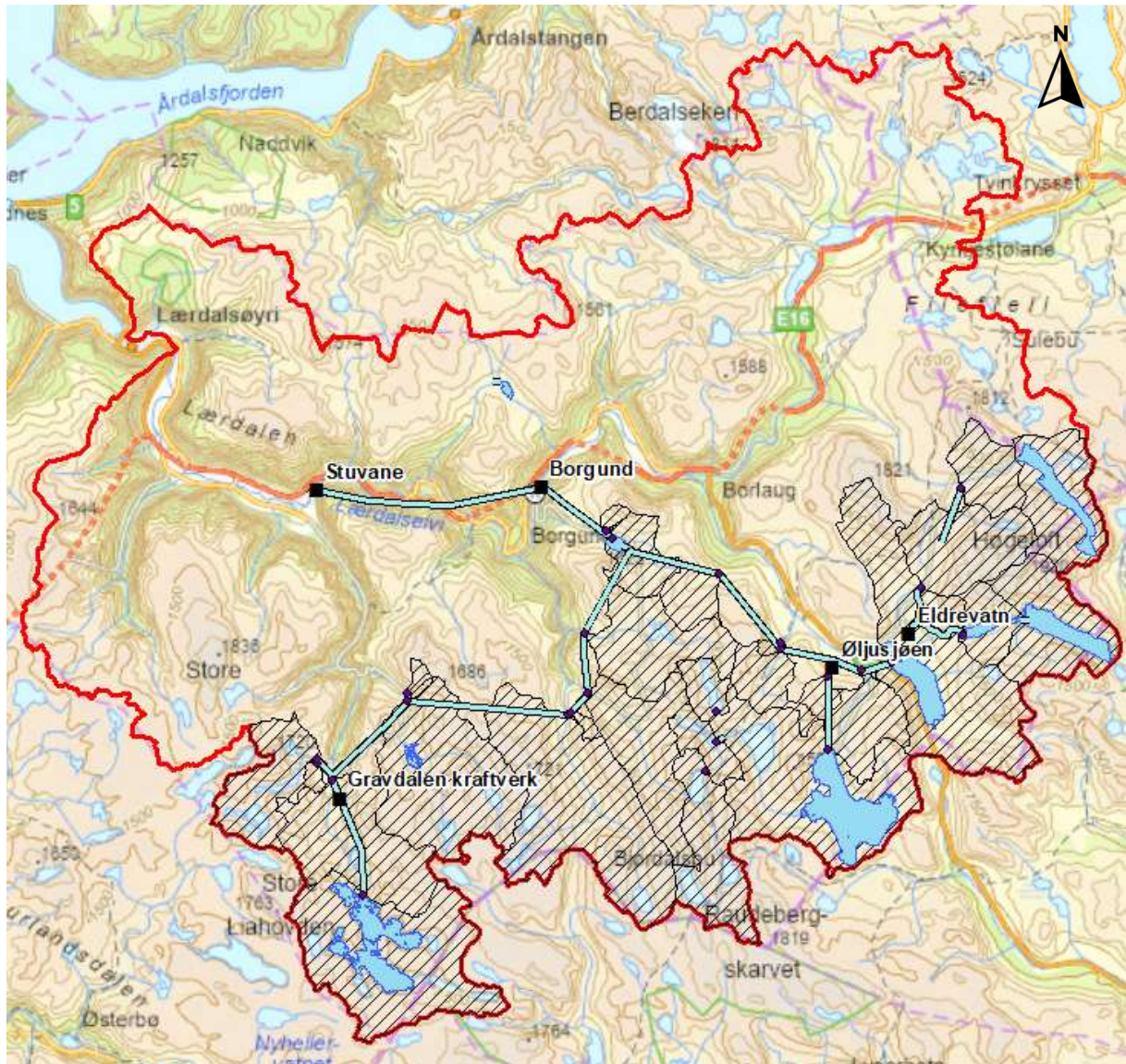
Figur 3-9: Regulerte felt (skravert) i feltet til Lærdalselva (rødt). Kartet viser kun felt som drenerer eller overføres til reguleringsmagasiner. Kraftverk som ikke påvirker flomforhold i Lærdalsøyri er ikke inkludert i kartet.
