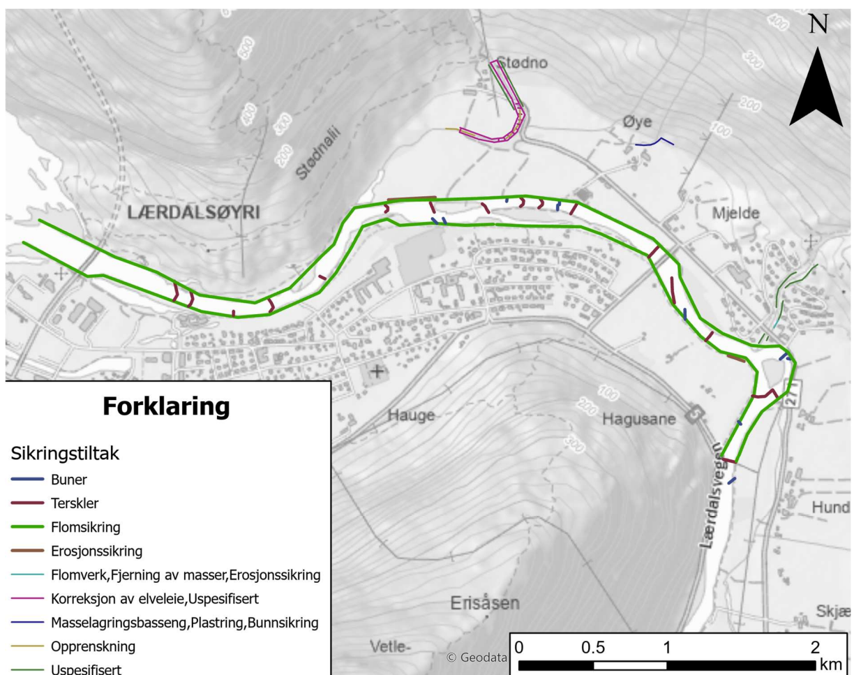
Figur 3-12: Eksisterende sikringstiltak registrert i NVE Atlas (NVE, 2024a).
