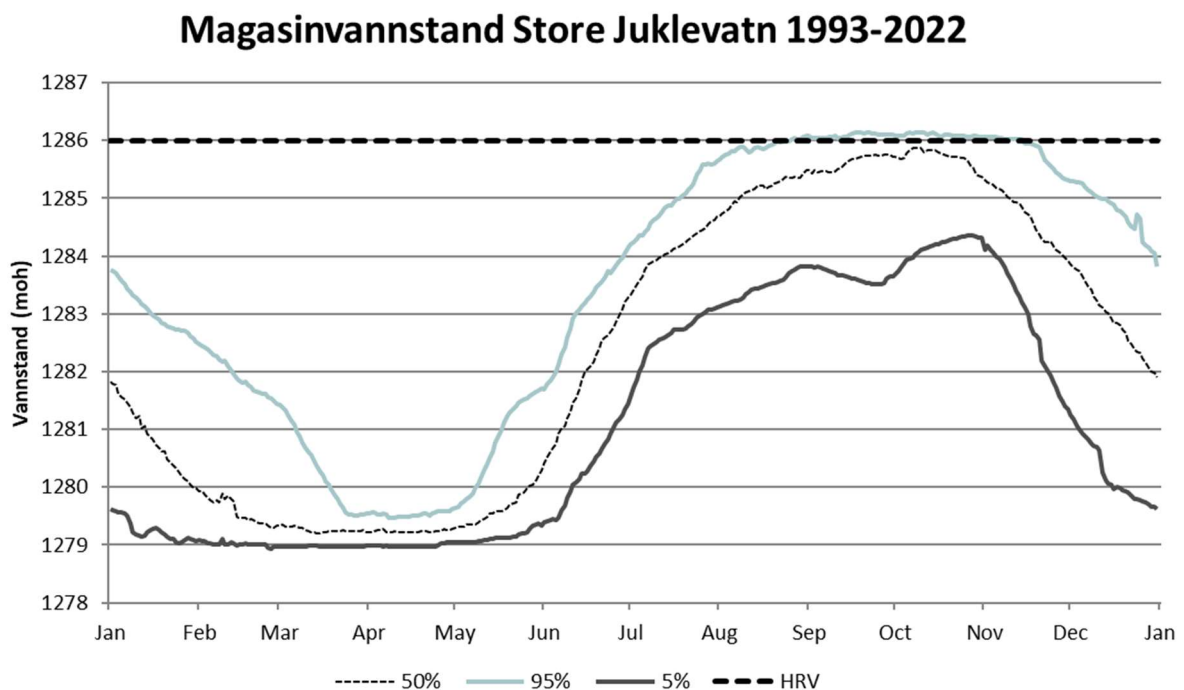
Figur 5-21: Historisk magasin vannstand ved Store Juklevatn.
