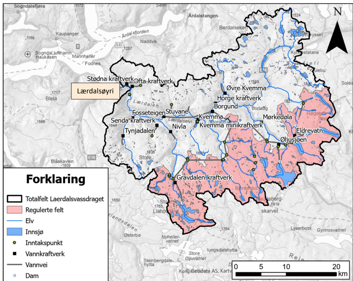
Figur 5-20: Oversiktskart som viser nedbørfeltet til Lærdalselva ved Lærdalsøyri samt regulerte felt.
