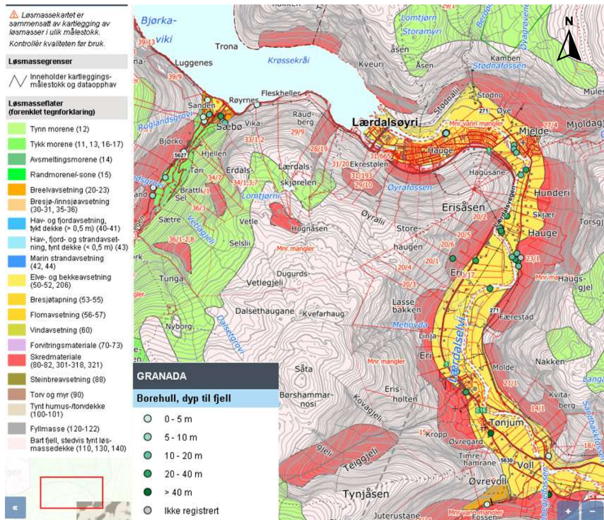
Figur 2-2: Løsmassegeologi for det aktuelle området med eksisterende borehull fargelagt etter dybde til fjell (NGU, 2023).
