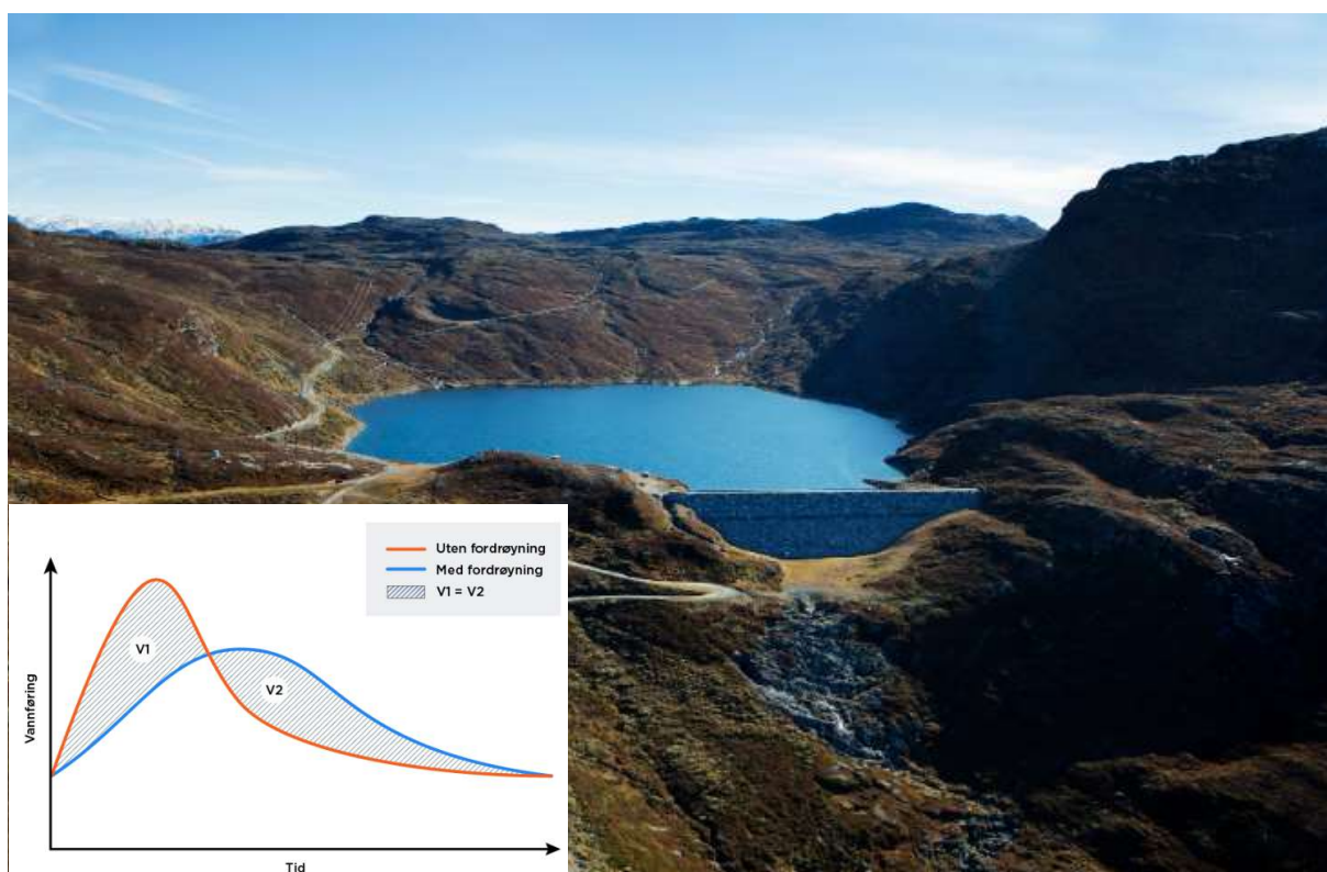
Figur 5-1: Eksempel på et eksisterende reguleringsmagasin i Lærdalsvassdraget: Dam Vassetvatn. Foto: Østfold Energi. Skissen, utarbeidet av NVE, illustrerer generelt hvordan fordrøynings tiltak påvirker flomstørrelsen ved forsinkelse og demping av flomtoppen.
