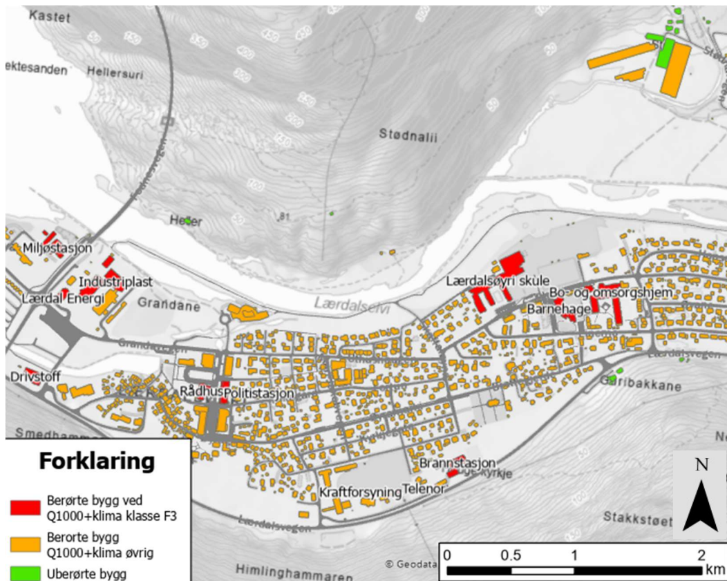
Figur 2-9: Kritiske objekt (sikkerhetsklasse F3) berørt ved 1000-årsflom inkl. klimapåslag i Lærdalsøyri (nedstrøms del).
