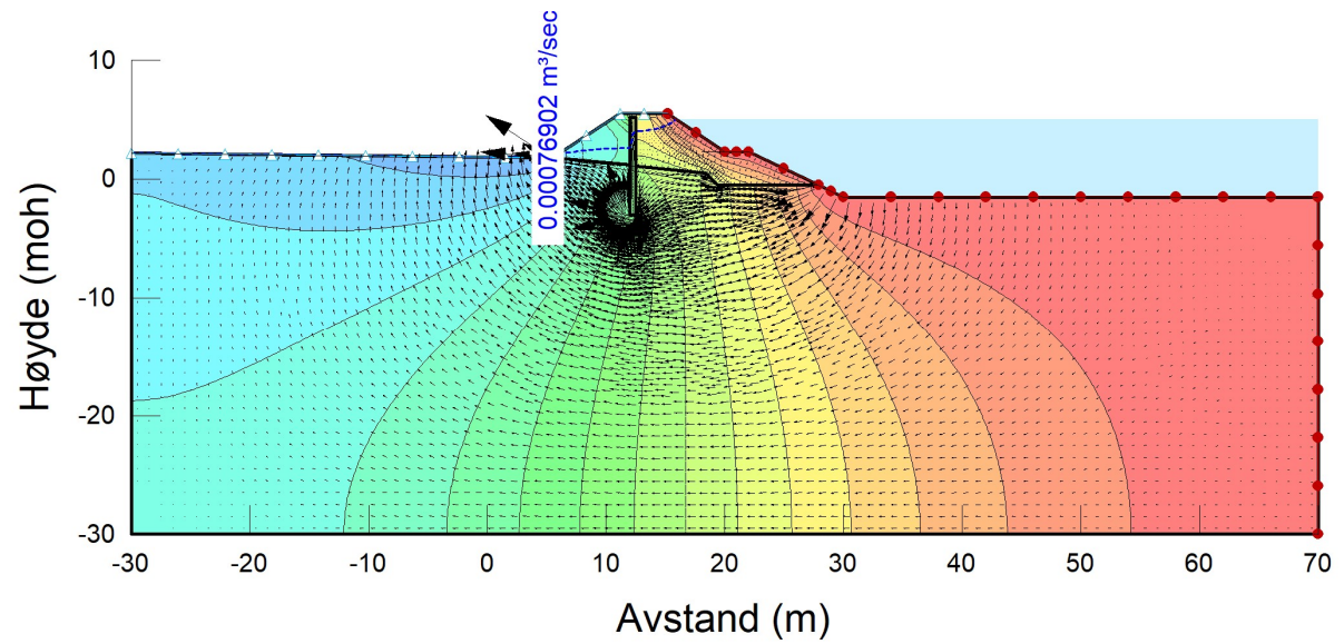
Figur 1-2: Eksempel på strømningsnett og resultatet fra modellforsøk med spunt.
