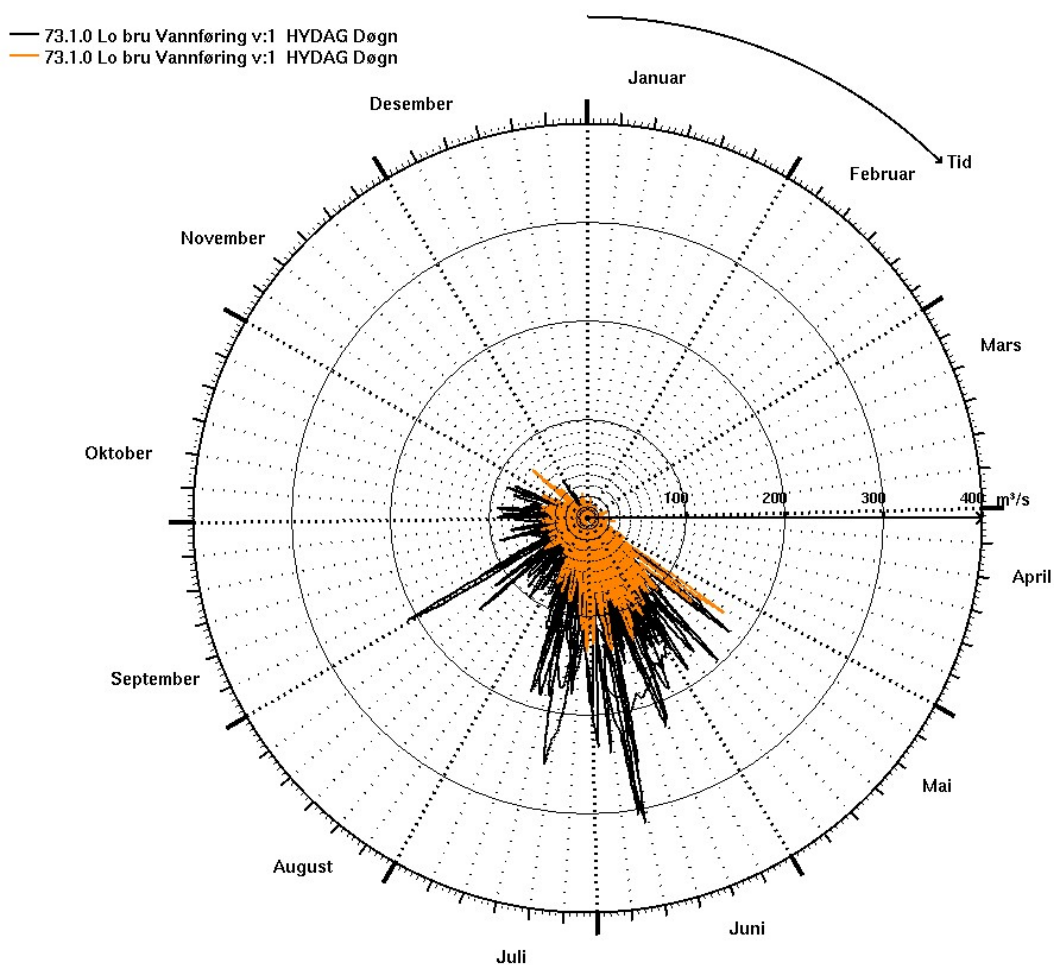
Figur 3-11: Årspolarplott for vannføring ved Lo bru før (svart) og etter (oransje) vassdraget ble regulert.
