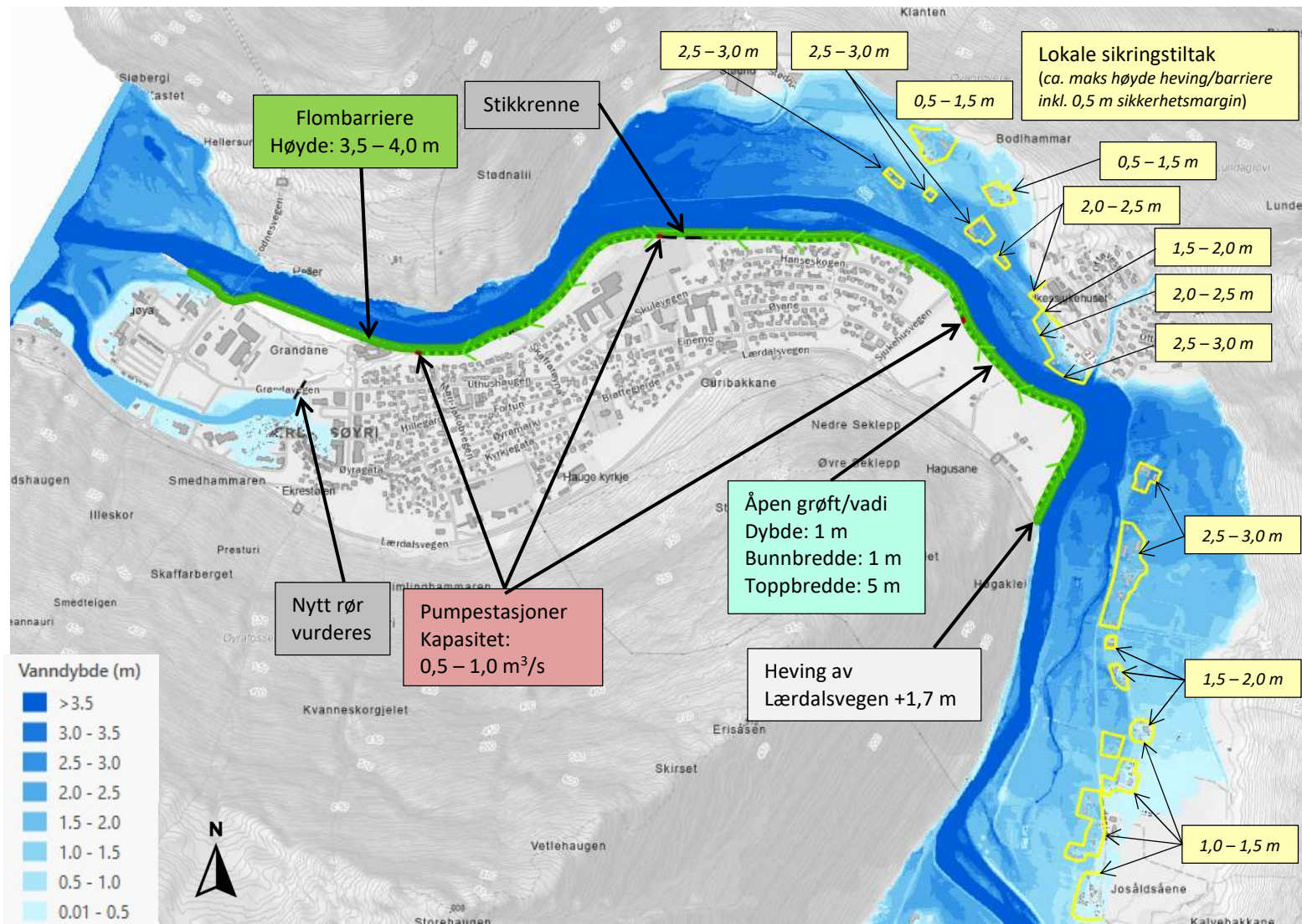
Figur 6-7: Oversiktskart over kombinerte tiltak for å sikre Lærdalsøyri ved en 1000-årsflom med 20% klimapåslag i tiltakskombinasjon 2B.
