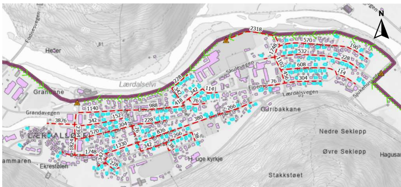
Figur 2-3: Vurdering av nytt dreneringssystem ved 1 meter grunnvannssenkning. Røde linjer viser plassering til de nye ledningene og tallene viser dimensjonerende vannmengde i l/s. Med lyseblå vises bygninger med kjeller.
