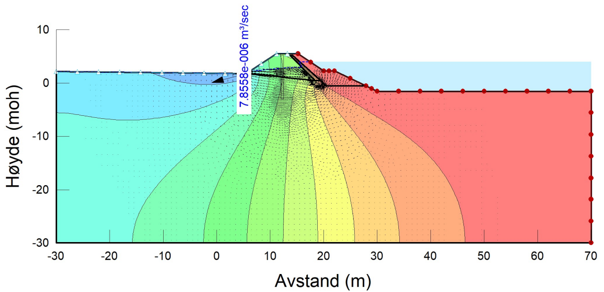
Figur 1-3: Eksempel strømningsnett og resultatet fra modellforsøk med morene-/leirtetning.
