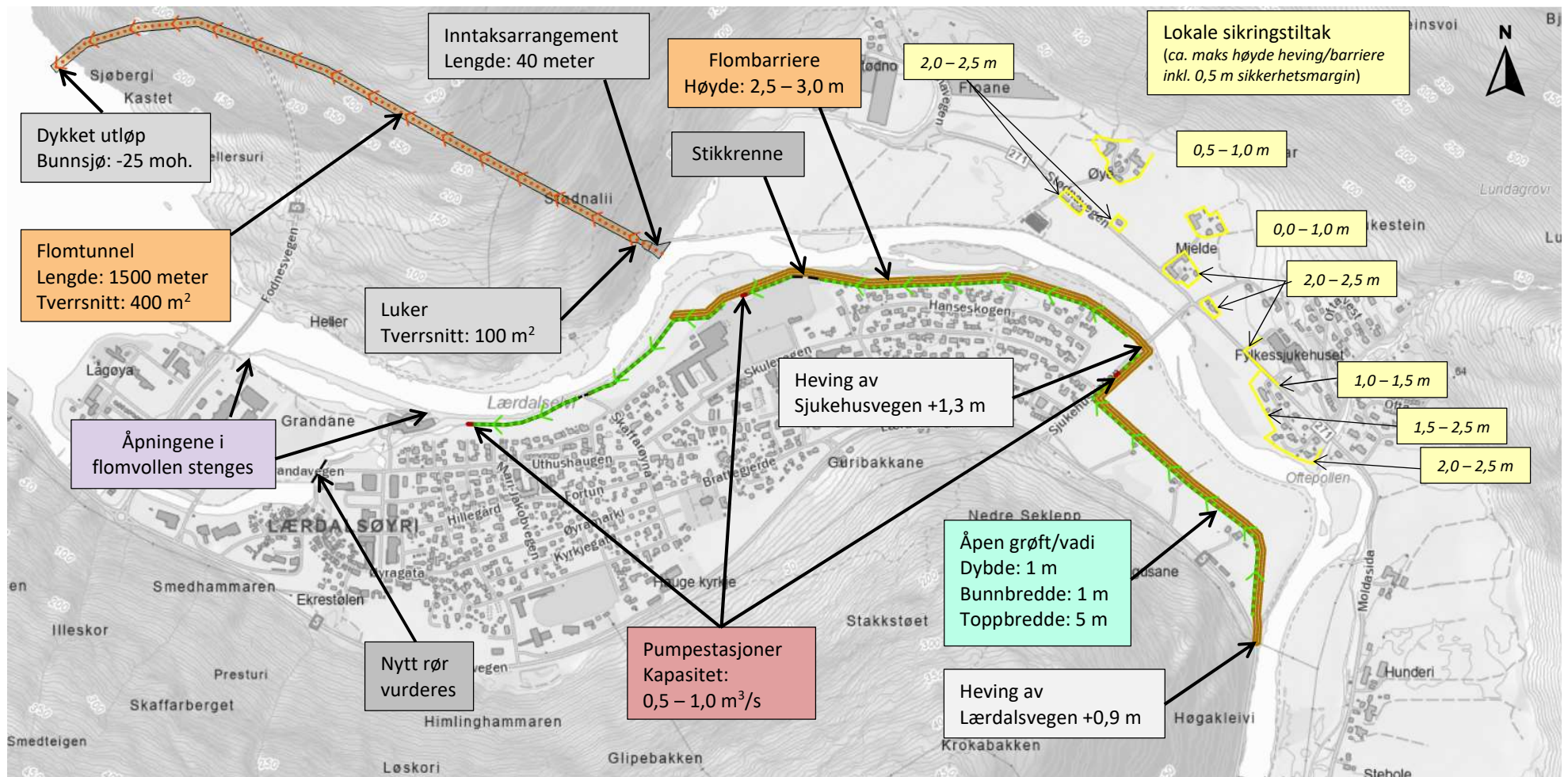
Figur 6-13: Oversiktskart over kombinerte tiltak for å sikre Lærdalsøyri ved en 1000-årsflom med 20% klimapåslag i tiltakskombinasjon 5.
