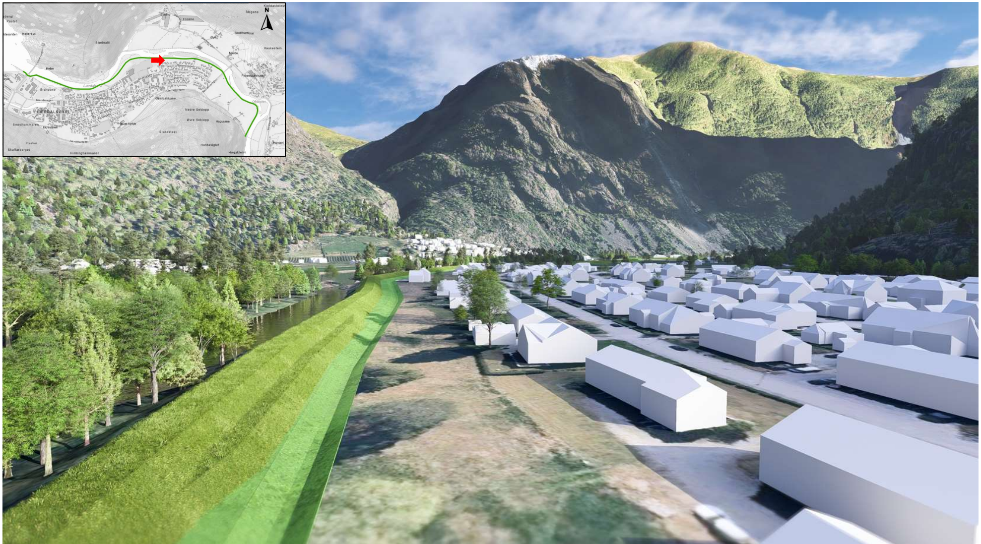
Figur 3-10: 3D-illustrasjon av planlagte flombarrierer og grøfter i tiltakskombinasjon 2B ved Hanseskogen sett fra vest.
