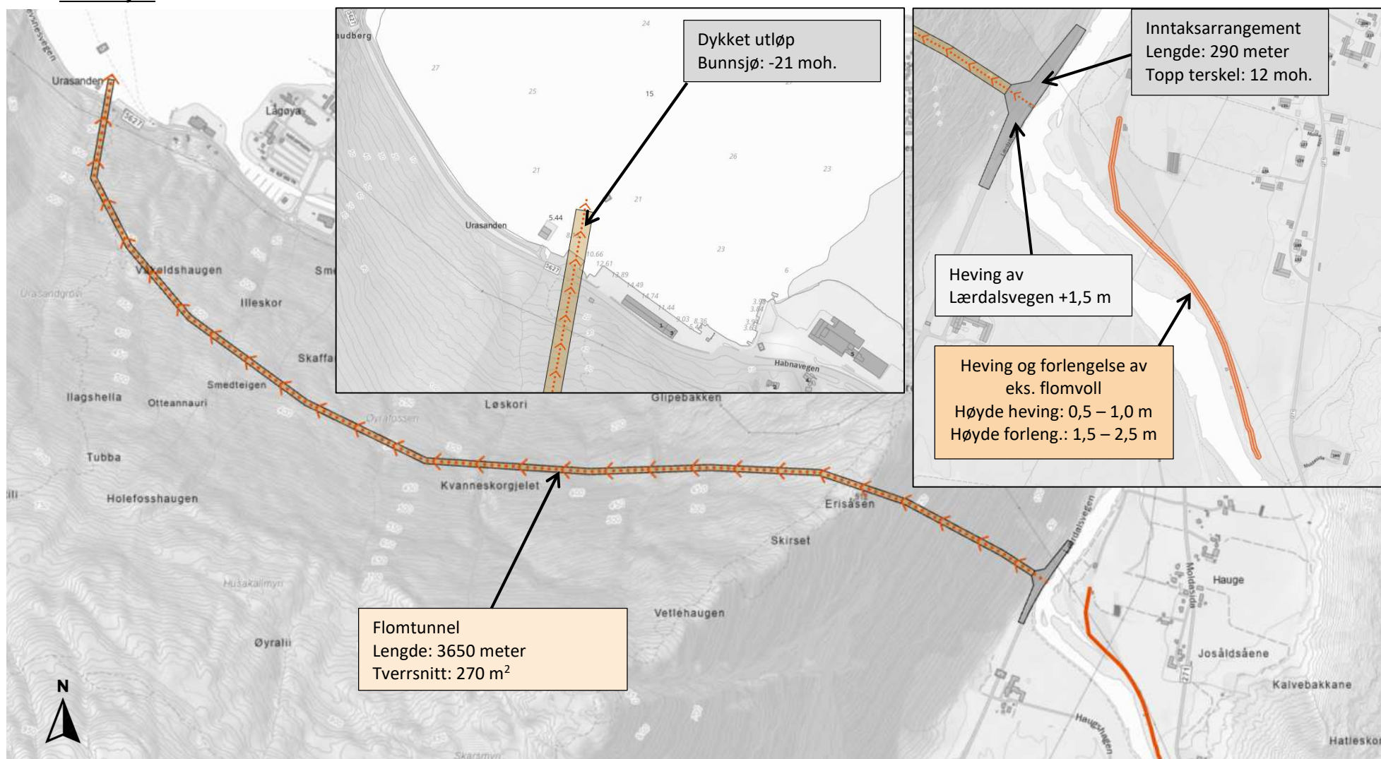
Figur 6-2: Oversiktskart over kombinerte tiltak for å sikre Lærdalsøyri ved en 1000-årsflom med 20% klimapåslag i tiltakskombinasjon 1.
