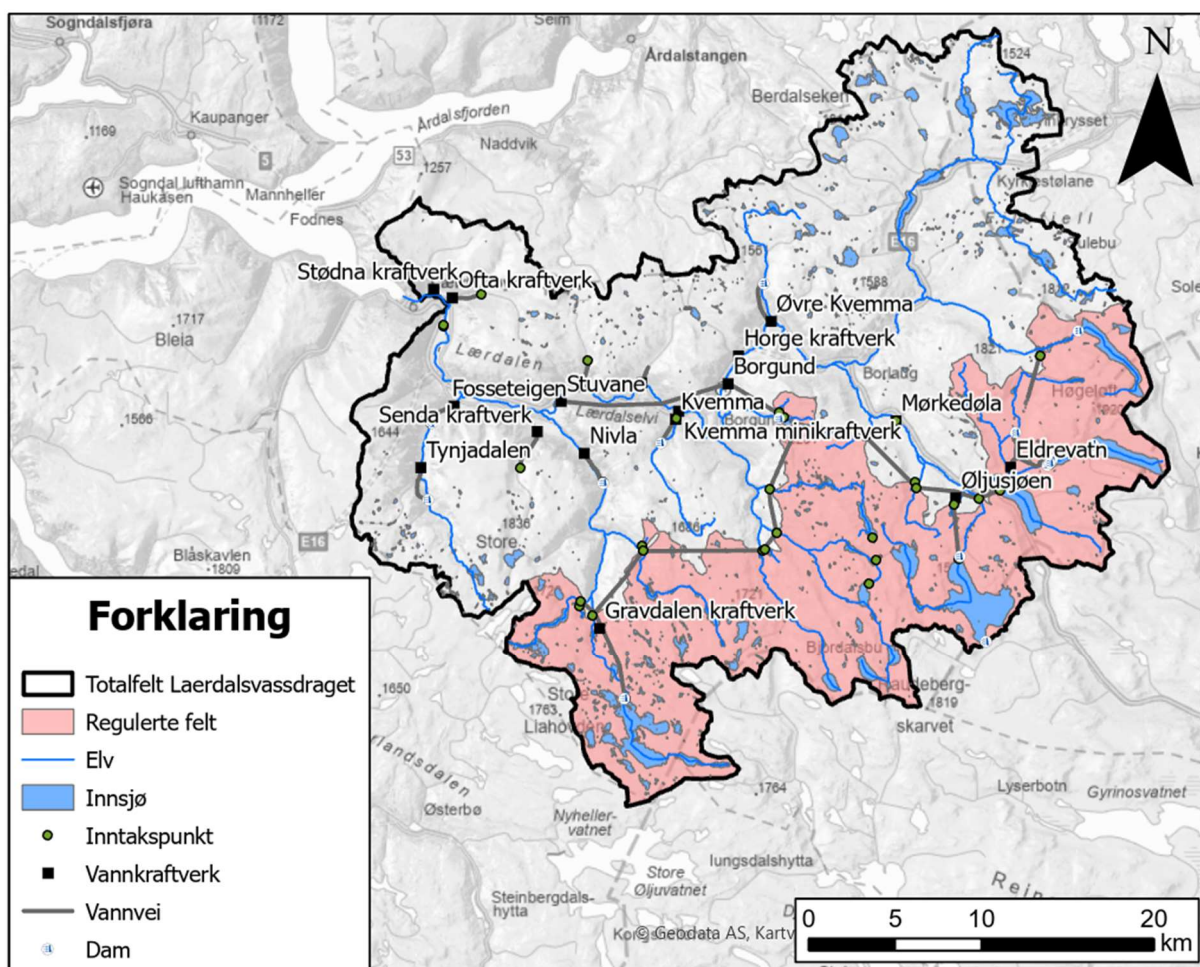
Figur 4-2: Vannkraftverk i nedbørfeltet.
