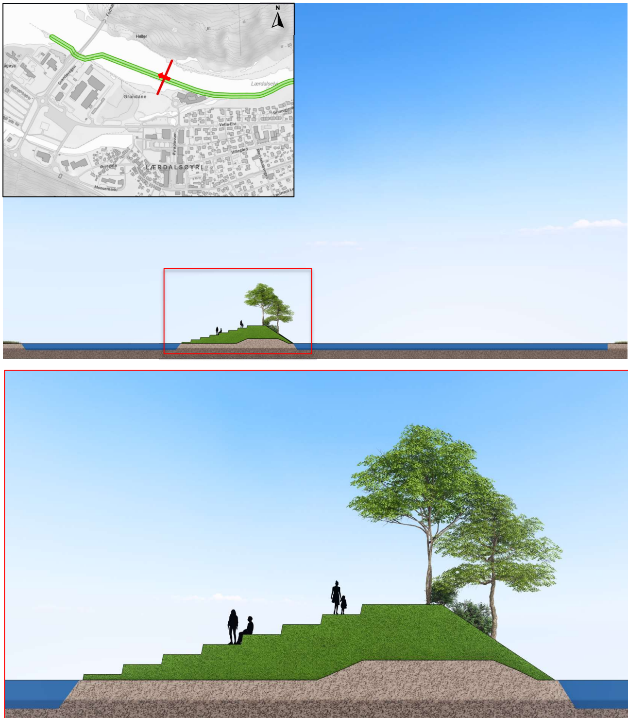
Figur 3-11: Snitt av planlagt flombarriere i tiltakskombinasjon 2B ved Grandane.
