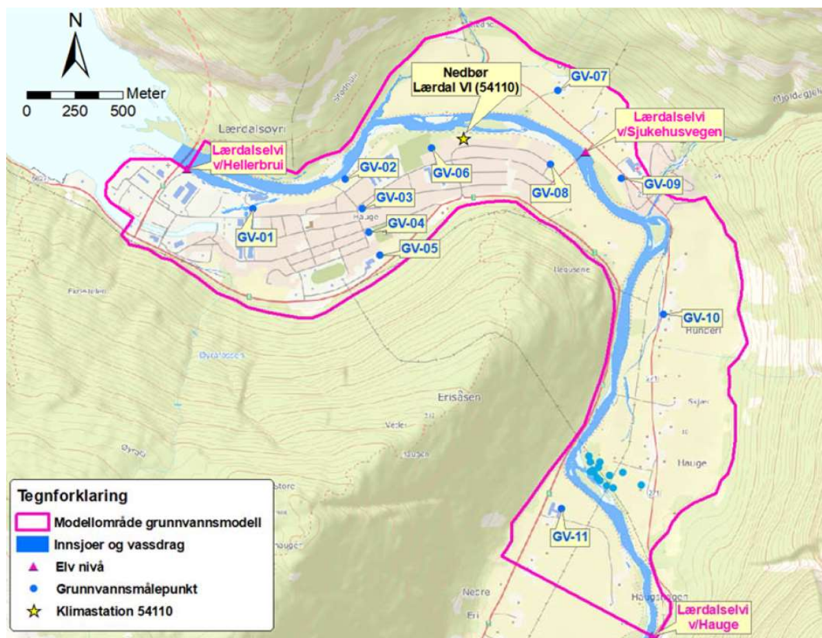
Figur 2-4: Kart med målepunkter for grunnvann og vannnivå i elv. Alle loggere er plassert innen modellområdet til grunnvannsmodellen (Dr. Blasy og Dr. Øverland, 2024).
