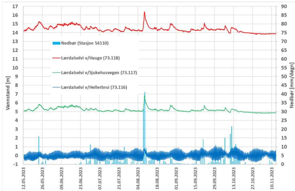
Figur 2-6: Tidsserier for vannstand i elven og nedbør (Dr. Blasy og Dr. Øverland, 2024).
