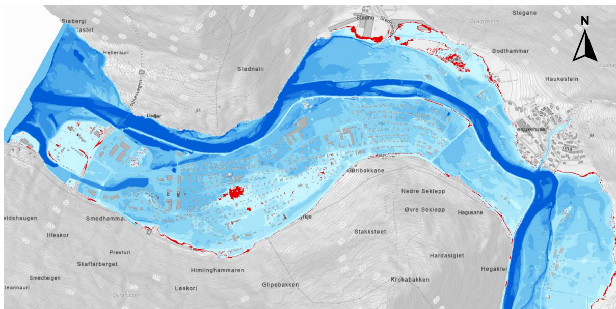
Figur 5-4: Flomsonekart ved en 200-årsflom med 20% klimapåslag. Røde områder viser ytterligere oversvømt areal ved en 1000-årsflom med 20% klimapåslag. Flere detaljer vises i Figur 6-1.
