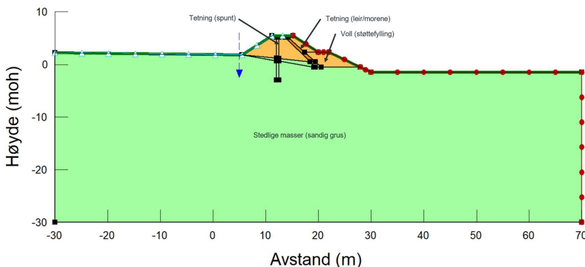
Figur 1-1: Flomvollgeometri og lagdeling brukt i analysen. Modellen er kjørt med to alternative tetningslag - spunt og morene, for å sammenligne effektene.
