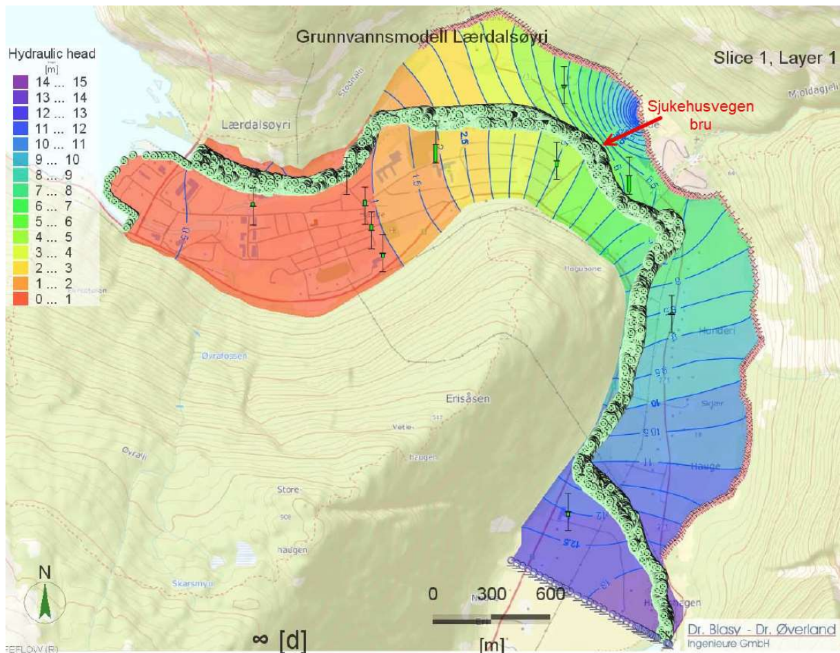
Figur 2-7: Modellresultat isolinjer grunnvannspotensial for stasjonær tilstand 05.08.2023 (Dr. Blasy og Dr. Øverland, 2024).
