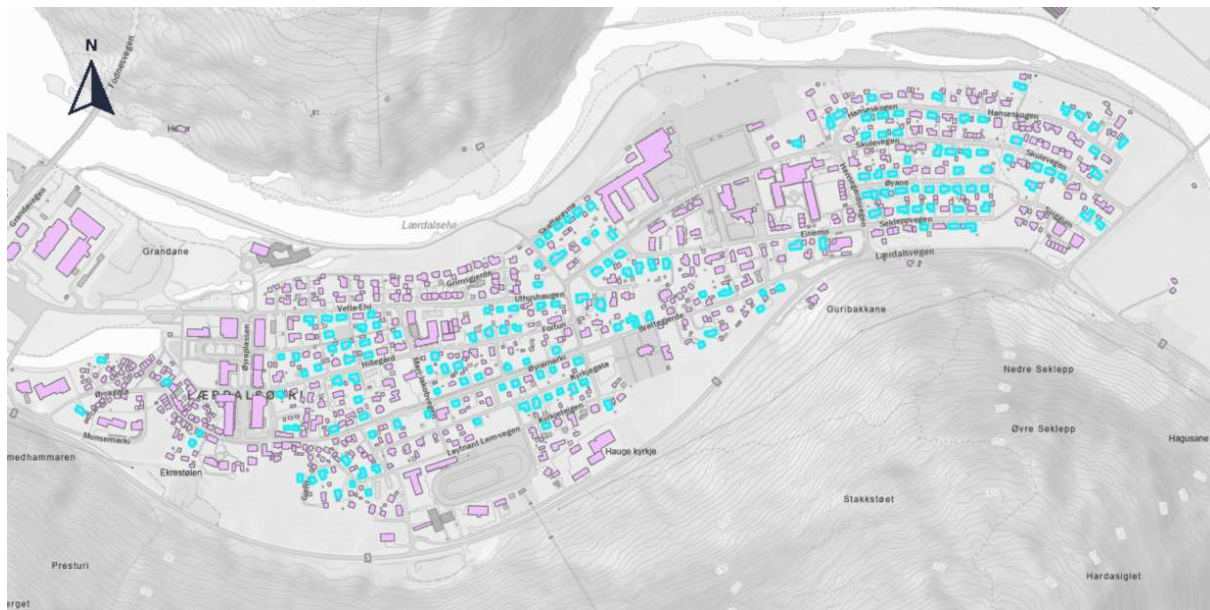
Figur 2-2: Plassering av bygninger med kjeller i Lærdalsøyri sentrum markert med blå farge.
