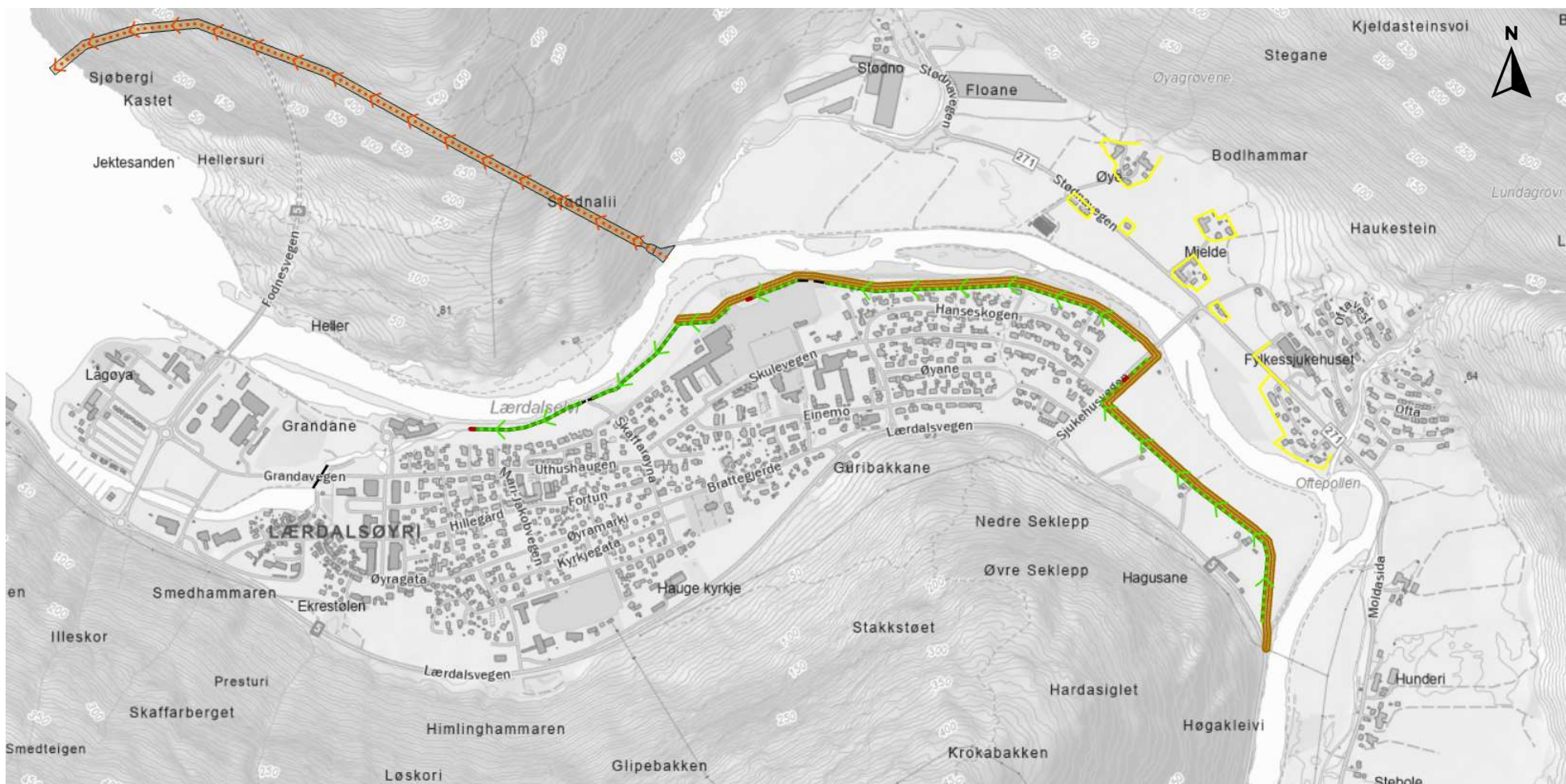
Figur 4-1: Oversiktskart over tiltakskombinasjon 5. Se Figur 6-13 i hovedrapporten for flere detaljer om tiltakene.
