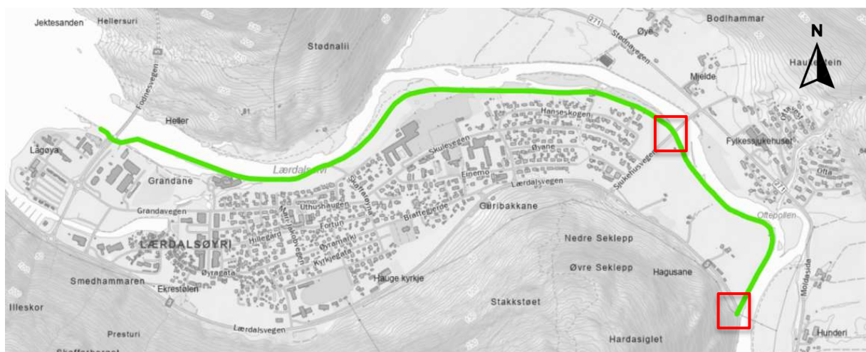
Figur 5-15: Oversikt over flombarrierens kryssinger ved kjøreveier: Sjukehusvegen (t.v.) og Lærdalsvegen (t.h.).
