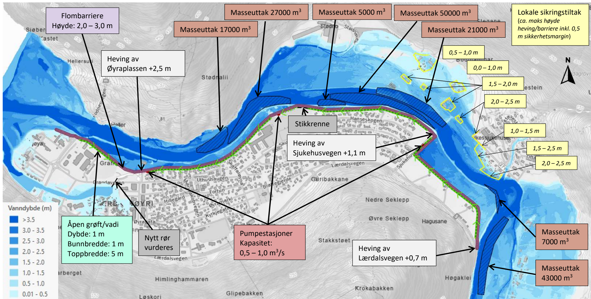
Figur 6-16: Oversiktskart over kombinerte tiltak for å sikre Lærdalsøyri ved en 1000-årsflom med 20% klimapåslag i tiltakskombinasjon 6.
