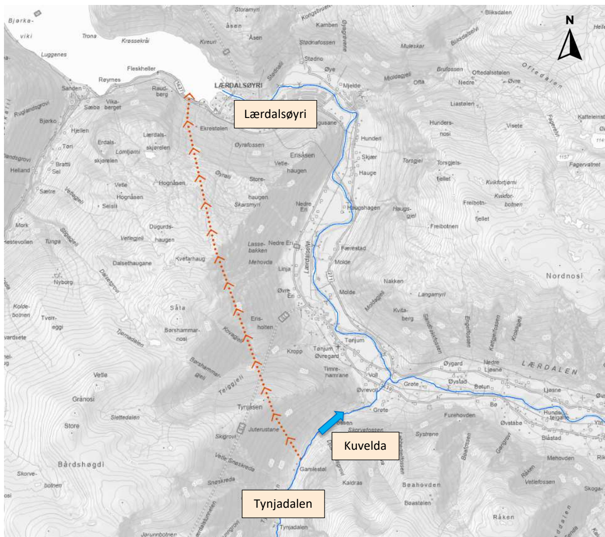
Figur 5-29: Oversiktskart som viser foreslått trase for flomtunnelen ved Tynjadalen.
