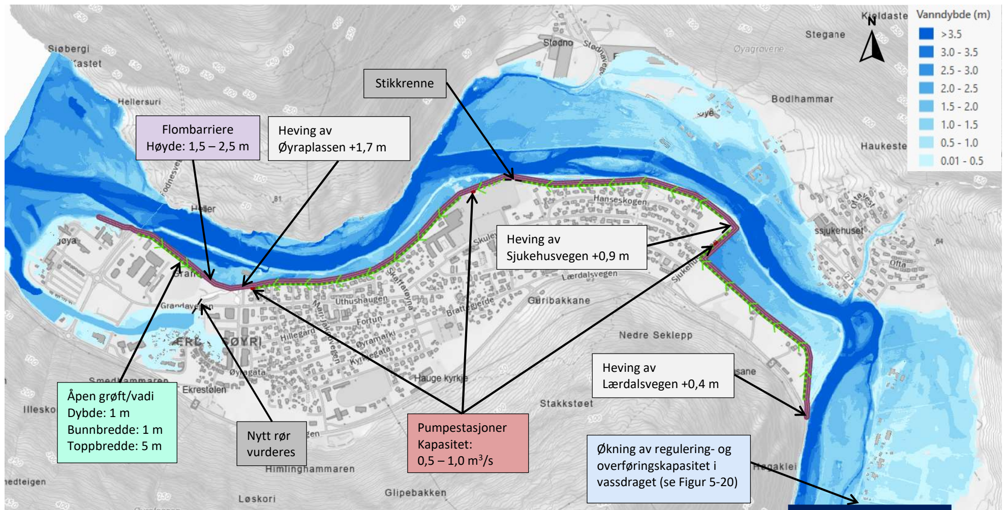
Figur 6-12: Oversiktskart over kombinerte tiltak for å sikre Lærdalsøyri ved en 1000-årsflom med 20% klimapåslag i tiltakskombinasjon 4.
