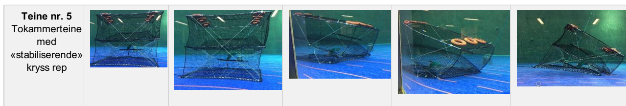
Figur 4. Bilder og beskrivelse av de 5 ulike riggingene av tokammerteinen som ble testet ut i strømtanken under økende strømforhold fra 0 til 1 knop.
