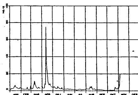
OPPSAL 1989
