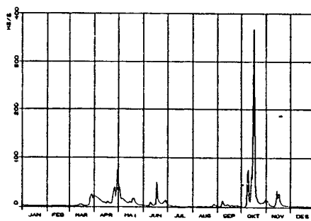
OPPSAL 1987
