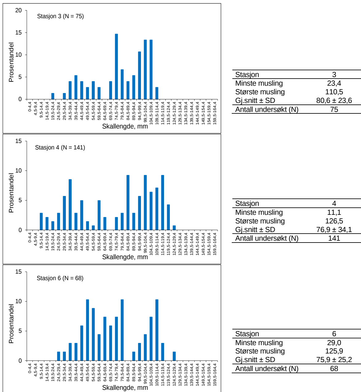
Figur 99. Lengdefordeling av levende elvemusling på stasjon 3, 4 og 6 i Vardneselva, basert på graving i substratet i slutten av juli 2023.
