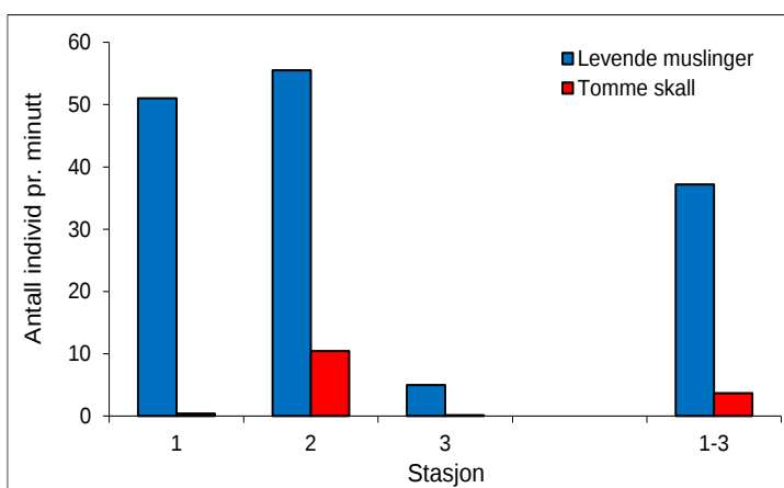
Figur 45. Tettheten av levende elvemusling og tomme skall, basert på tidsbegrensede tellinger (oppgitt som antall individ pr. minutt) på tre stasjoner i Nytingneselva i 2023.
