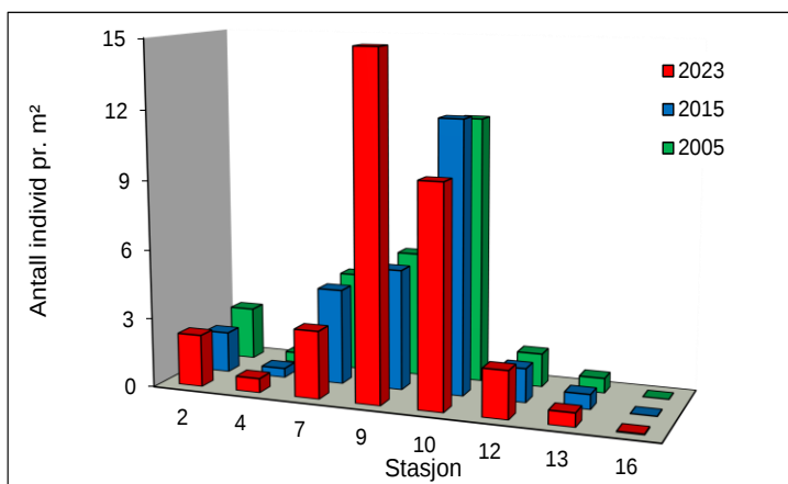
Figur 114. Tettheten av levende elvemusling, basert på tellinger i transekter på åtte stasjoner (oppgitt som antall individ pr. m²) i Karpelva i 2005, 2015 og 2023.
