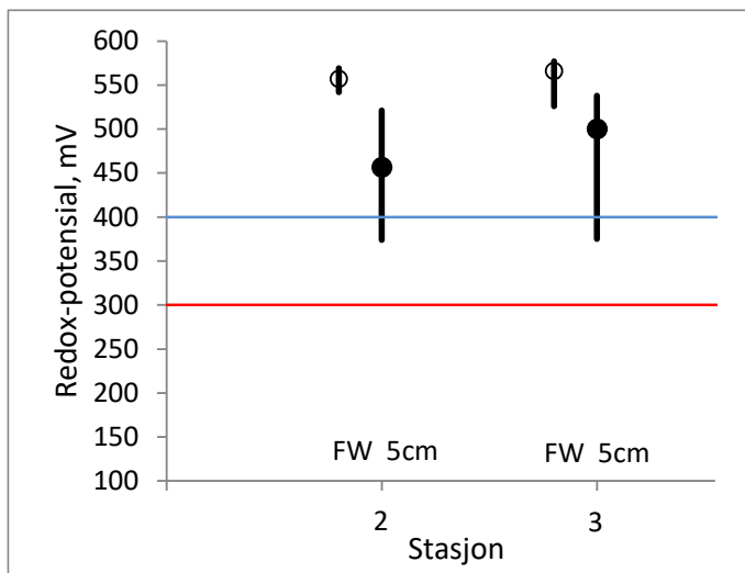
Figur 15. Redoksmålinger i Hopselva på to stasjoner (stasjon 2 og 3) i juni 2023. Median, minimums- og maksimumsverdi for målinger i de frie vannmasser (FW) og på 5–7 cm dyp i substratet (5 cm) er gitt for hver enkelt stasjon. Tabelloversikten angir antall målinger som ligger til grunn og andel av måleresultatene fordelt på redokspotensial >400 mV (ovenfor blå heltrukken linje), 300–400 mV (mellom blå og rød heltrukken linje) og <300 mV (nedenfor rød heltrukken linje).
