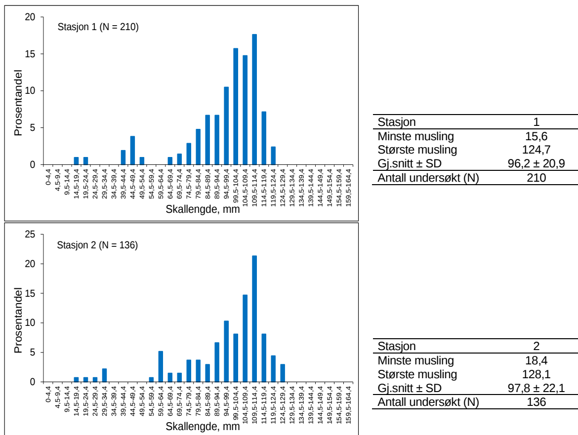
Figur 47. Lengdefordeling av levende elvemusling på stasjon 1 og 2 i Nytingneselva, basert på graving i substratet i slutten av juni 2023.
