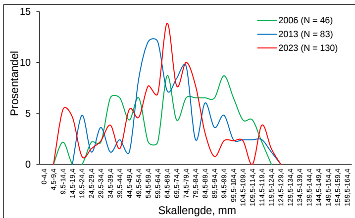
Figur 92. Lengdefordeling av levende elvemusling i Bødalselva i 2023 sammenlignet med 2006 og 2013. Det ble ikke gravd i substratet i 2006 og 2013.
