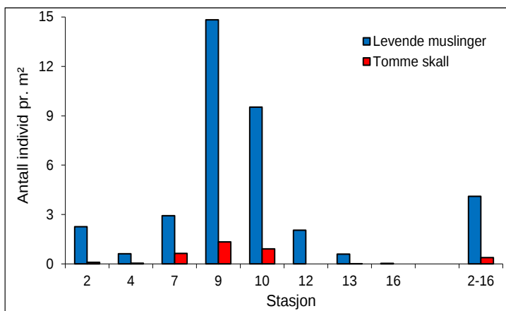
Figur 107. Tettheten av levende elvemusling og tomme skall, basert på tellinger i transekter (oppgitt som antall individ pr. m²) på åtte stasjoner i Karpelva i 2023.
