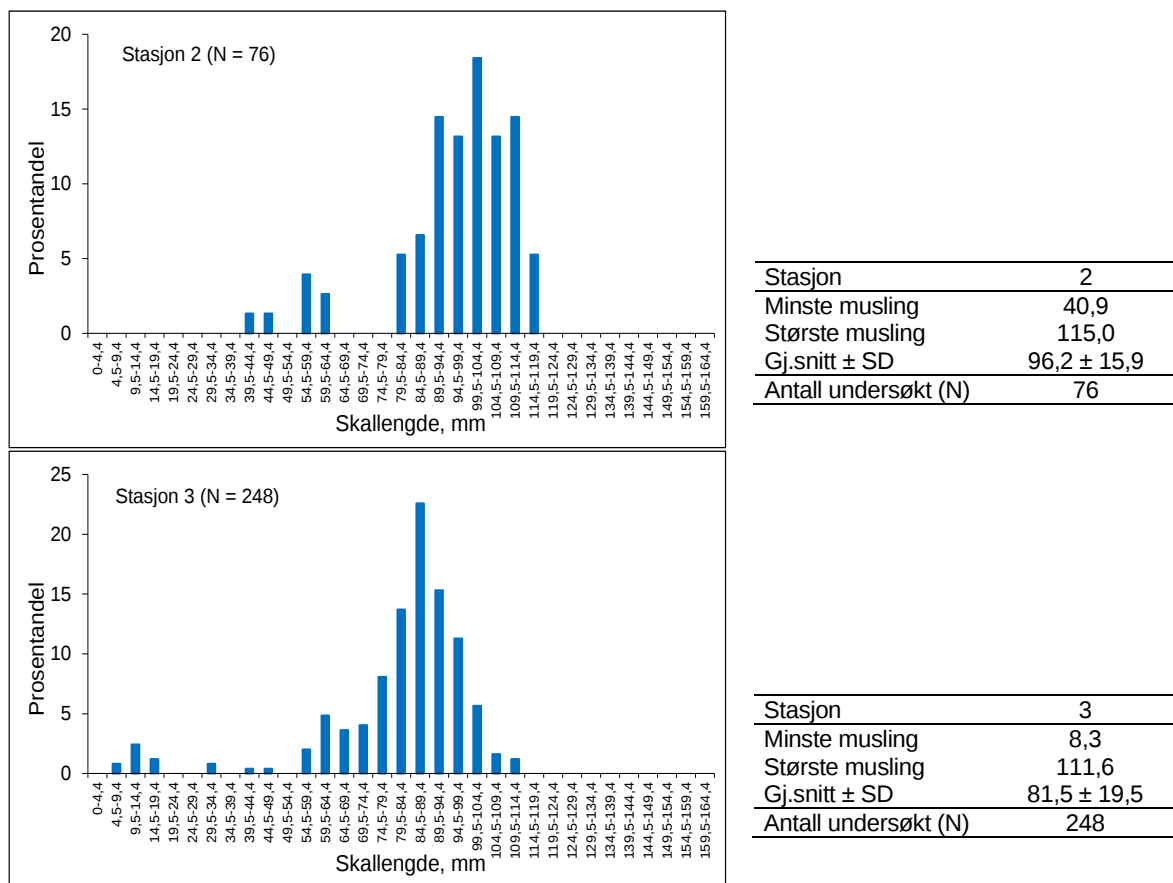
Figur 58. Lengdefordeling av levende elvemusling på stasjon 2 og 3 i Borgelva, basert på graving i substratet i slutten av juli 2023.
