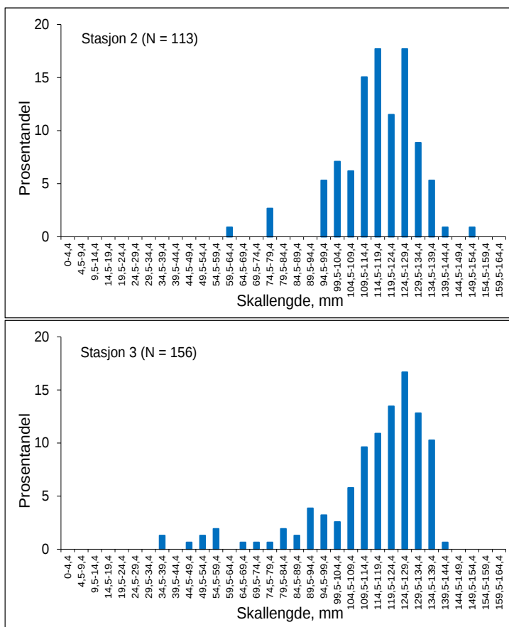
Figur 19. Lengdefordeling av levende elvemusling på stasjon 2 og 3 i Hopselva basert på graving i substratet i slutten av juni 2023.
