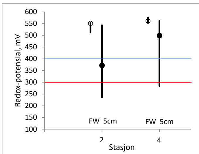
Figur 63. Redoksmålinger i Gryttingselva på to stasjoner (stasjon 2 og 4) i juli 2023. Median, minimums- og maksimumsverdi for målinger i de frie vannmasser (FW) og på 5–7 cm dyp i substratet (5 cm) er gitt for hver enkelt stasjon. Tabelloversikten angir antall målinger som ligger til grunn og andel av måleresultatene fordelt på redokspotensial >400 mV (ovenfor blå heltrukken linje), 300–400 mV (mellom blå og rød heltrukken linje) og <300 mV (nedenfor rød heltrukken linje).
