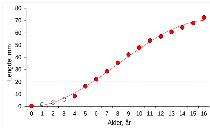
Figur 21. Vekstkurve basert på lengde av gjennomsnittlig årringsdiameter hos aldersbestemte elvemusling i Hopselva fram til 16-årsalder (N = 11). Skallene var erodert ved umbo, slik at de første vintersonene ikke lenger kunne bestemmes med sikkerhet, og vekstkurven er stipulert for de tre første leveårene (åpne sirkler).
