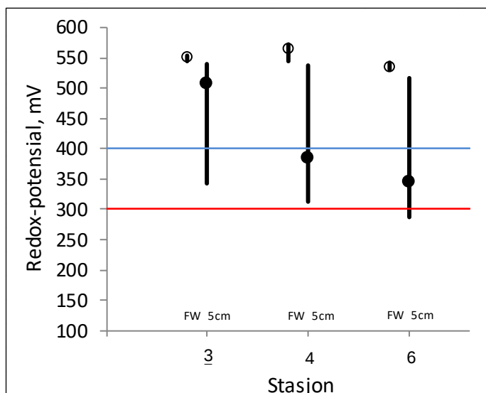
Figur 93. Redoksmålinger i Vardneselva på tre stasjoner (stasjon 3, 4 og 6) i juli 2023. Median, minimums- og maksimumsverdi for målinger i de frie vannmasser (FW) og på 5–7 cm dyp i substratet (5 cm) er gitt for hver enkelt stasjon. Tabelloversikten angir antall målinger som ligger til grunn og andel av måleresultatene fordelt på redokspotensial >400 mV (ovenfor blå stiplede linje), 300–400 mV (mellom blå og rød stiplede linje) og <300 mV (nedenfor rød stiplede linje).
