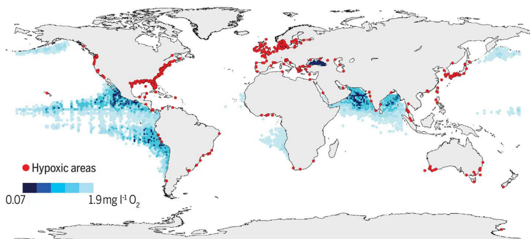
Figur 1: Lavt og synkende oksygenivå i åpent hav og kystvann påvirker alt fra biogeokjemi prosesser til matsikkerhet. Det globale kartet viser kystområder oksygenkonsentrasjonen er redusert til lavere enn 2 \text{ mg/L} . Dette tilsvarer det som ville blitt klassifisert som svært dårlige forhold i henhold til Tabell 1 ( <1.5 \text{ mL/L} ). De røde prikkene markerer områder hvor det er hypoksiske forhold, mens fargesskalen viser minimumssoner i 300 m dyp (blå skyggelagte områder). [Kart laget av data levert av R. Diaz, oppdatert av medlemmer av GO2NE-nettverket, og lastet ned fra World Ocean Atlas 2009].
