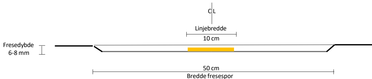
Figur 1: Fresespor ved plan nedfresing av midtlinje
