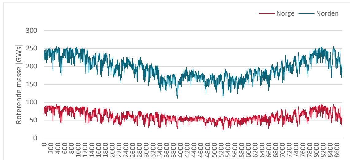
Figur 21: Timesverdier for mengde roterende masse i Norge og Norden for 2021.
