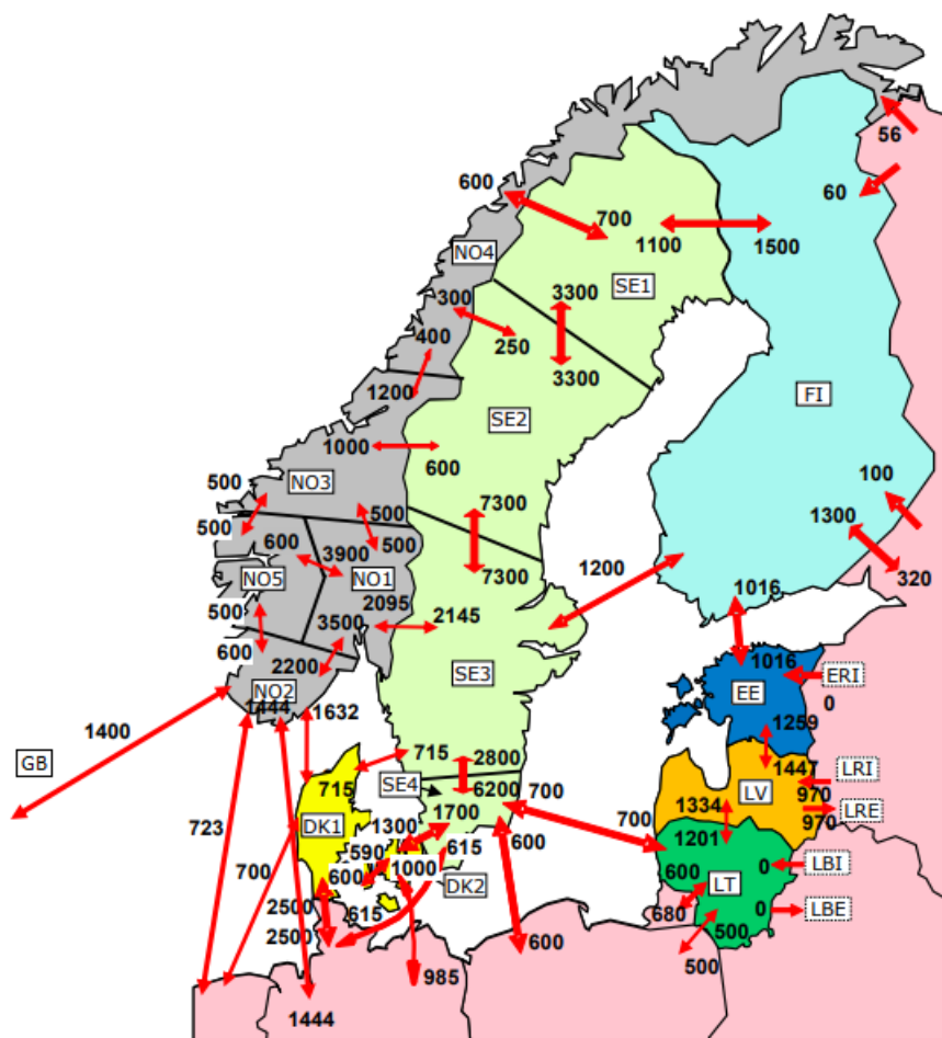
Figur 35: Maksimal handelskapasitet (NTC) i Norden (oppdatert 12. januar 2022) [15]
