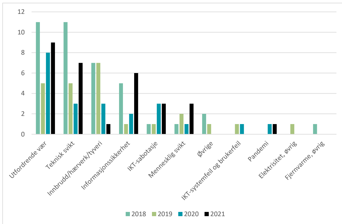
Figur 19: Grov kategorisering av uønskede hendelser som NVE er gjort kjent med i perioden 2018-2021. Antall hendelser for hver kategori er vist eksplisitt for 2021 [12].
