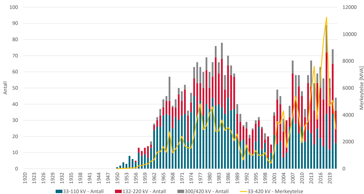
Figur 10 Oversikt over aldersfordelingen og total merkeytelse for transformatorer i regional- og transmisjonsnettet
