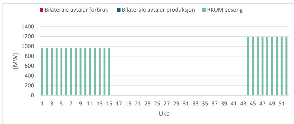
Figur 28: Kjøpte RK-opsjoner for sesongmarked og bilaterale avtaler fordelt ukesvis for 2021. Det har for 2021 ikke vært bilaterale avtaler på forbruk og produksjon.
