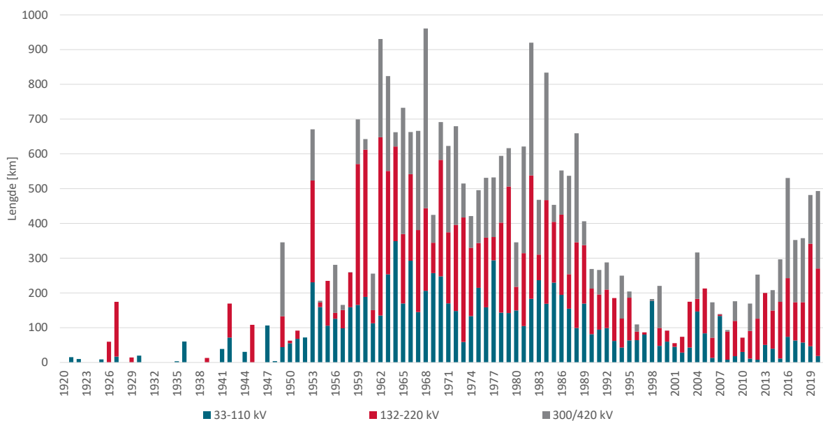
Figur 7 Oversikt over aldersfordelingen av luftledninger i regional- og transmisjonsnett
