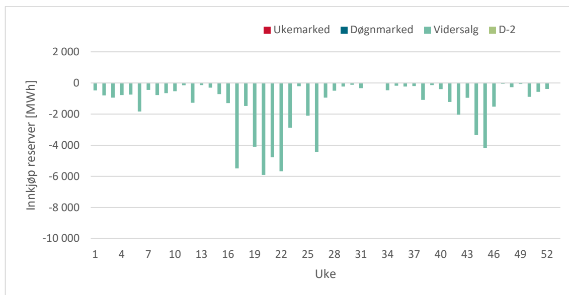
Figur 25 Innkjøp og videresalg driftsforstyrrelsesreserve (FCR-D) i MWh per uke i 2021.
