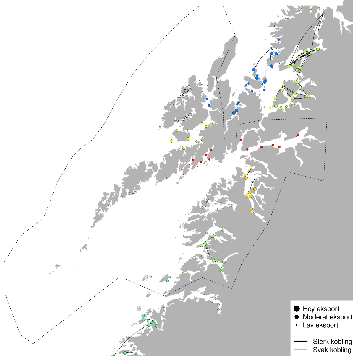
Figur 60: Sterkaste smittevegar for lakselus gjennom året 2024
