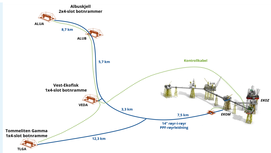
Figur 9: Innfasing av felt som tidlegare har vore i produksjon. Illustrasjon: ConocoPhillips.
