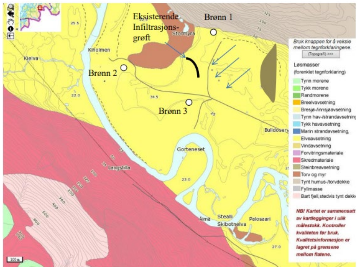
Figur 3 Lokalisering av gammel infiltrasjonsgrøft og miljøbrønner. Grunnvannets strømningsretning fra anlegget mot elven er angitt med blå piler.
