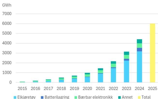
Figur 1. Utvikling i total installert litium-ion batterilagringskapasitet globalt, fordelt på formål, 2015-2025. Kilde: IEA 2026. [1] *
