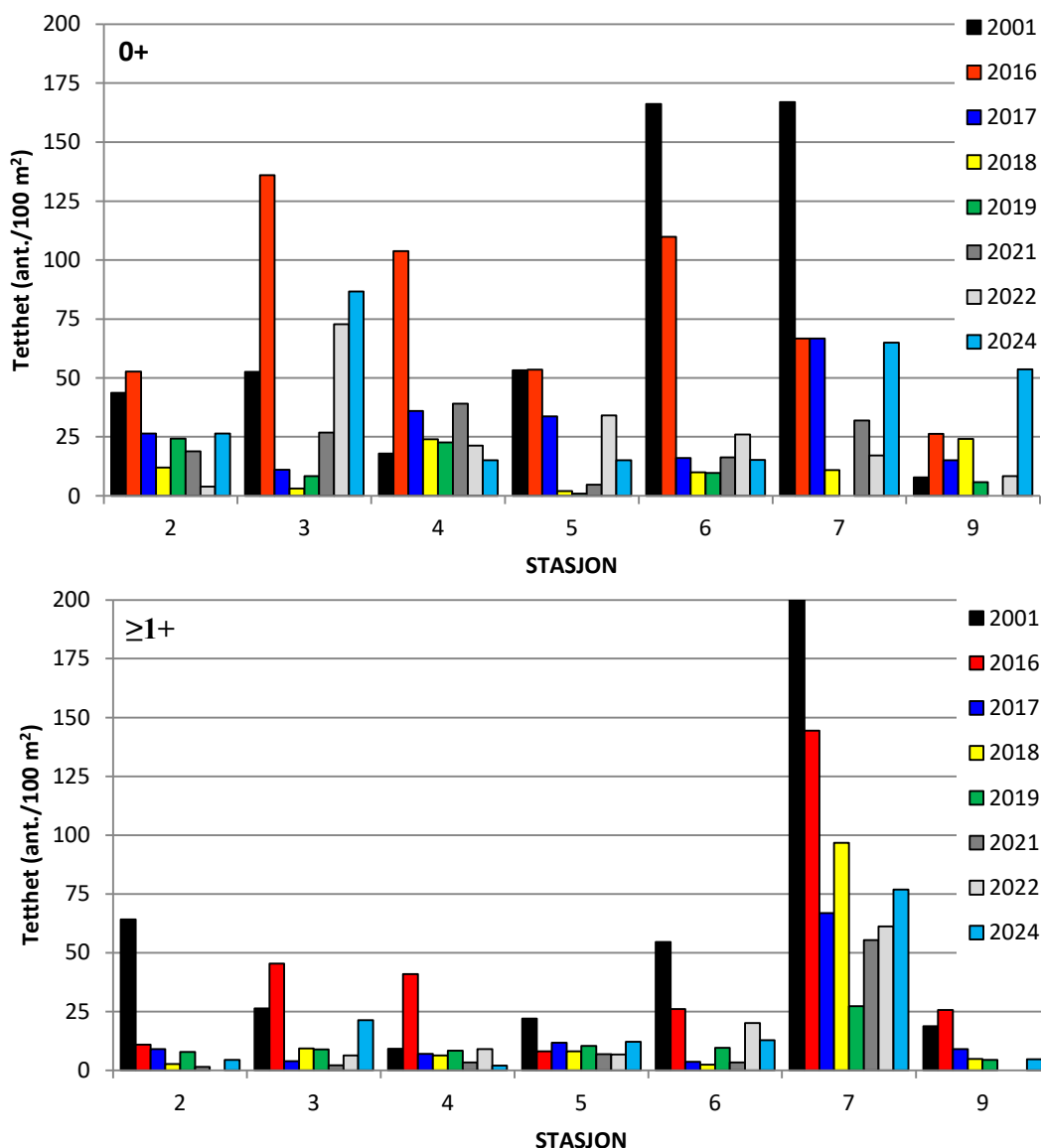
Figur 3.5. Beregnet tetthet (antall pr. 100 m 2 ) av 0+ og ørret \geq 1+ på de ulike stasjoner i Hemsil ovenfor Eikredammen som er undersøkt i hele perioden fra 2001.
