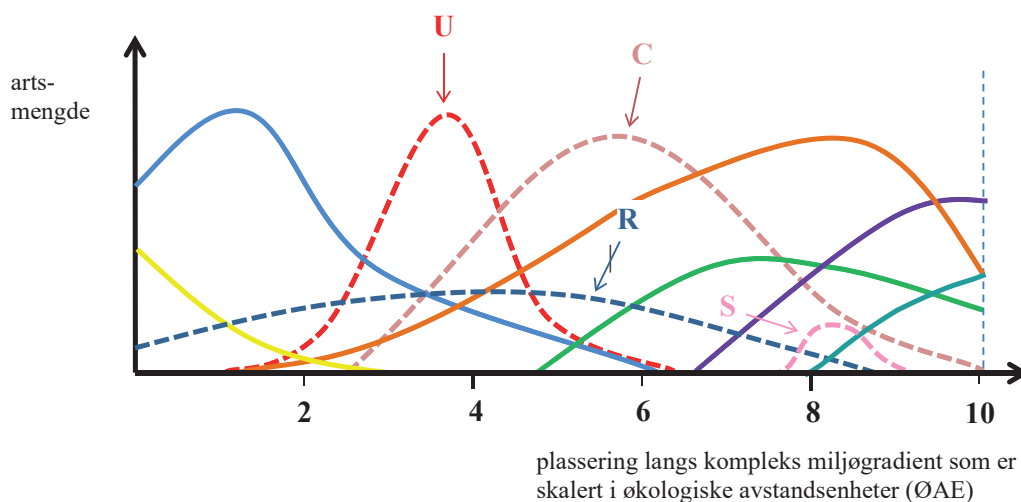
Fig. A1-5. Den unimodale artsresponsmodellen. Figuren viser artsresponskurver for 10 arter langs én kompleks miljøgradient, det vil si i et økologisk rom med bare én dimensjon. De fire kategoriene av artsresponsmønstre som blir definert ifølge CURS-modellen (se teksten for nærmere forklaring), er eksemplifisert ved arter hvis mengde er angitt med stipla linjer: C = kjerneart ( core species ), U = urban art ( urban species ), R = rural art ( rural species ), S = satelittart ( satellite species ). Den komplekse miljøgradienten (x-aksen) er skalert i økologiske avstandsenheter (ØAE), et nøkkelbegrep i NiN-sammenheng som er definert og drøftet i kapittel B2).
