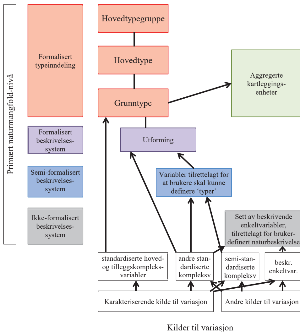
Fig. A2–3. Prinsippkisse for oppbygning av typeinndeling og beskrivelsessystem på et gitt primært naturmangfoldnivå i NiN versjon 2.
