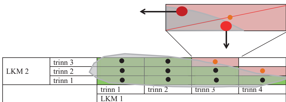
Fig. B4-2. Virkningen av tilleggskriterium 6 for inndeling av natursystem-hovedtyper i grunntyper, vist i grunntypediagrammet for en tenkt hovedtype som omfatter variasjon langs to LKM, LKM 1 med fire realisererte trinn og LKM2 med tre realisererte trinn innenfor hovedtypen. Grunntypediagrammet viser hovedtypens kompleksvariabelrom, men med ulik skala på x- og y-aksene i det todimensjonale koordinatsystemet (en celle i grammet svarer til ca. 1 ØAE langs begge akser). Den tykke grå streken i den nederste delfiguren omslutter kombinasjoner av miljøforhold som er, eller under normale omstendigheter (jf. tilleggskriterium 5) antas å være, realisert. Kriterium 6 medfører at de 9 cellene med midtpunkt i det økologiske rommet markert med svart prikk blir grunntyper, mens de to hvor midtpunktet er markert med oransje prikk ikke blir det. Den øverste delfiguren viser hvordan to konkrete arealenheter med plassering i det økologiske rommet gitt av den store mørkerøde og den store røde prikken blir tilordne nabo-grunntypene, henholdsvis for LKM1 trinn 2 & LKM2 trinn 3 og LKM1 trinn 3 & LKM2 trinn 2.
