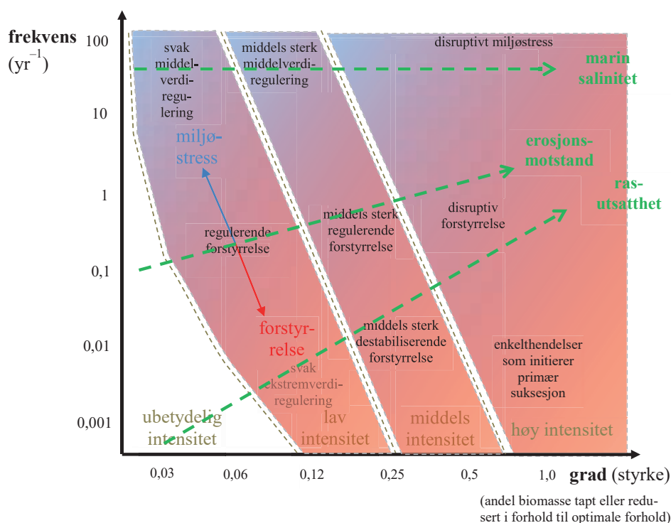
Fig. B3–3. Plassering av tre utvalgte lokale komplekse miljøgradienter i forhold til grad (styrke) av hver enkelt påvirkning utenfra som artene har begrenset toleranse overfor, påvirkningenes frekvens og den samlete intensiteten av slike påvirkninger. Graden (styrken) av påvirkninger utenfra er angitt som andelen av biomassen tapt i en forstyrrelsesbegivenhet eller reduksjonen i produktivitet som skyldes miljøstress i forhold til produktiviteten under optimale forhold, når alle andre miljøforhold enn den aktuelle påvirkningen holdes konstante. Brutte linjer skiller mellom fire nivåer av total påvirkningsintensitet: ubetydelig, lav, moderat og høy intensitet. Gradienten i dominerende prosess fra forstyrrelse (ekstremverdiregulering) til miljøstress (middelverdiregulering) er angitt som en gradient fra rød til blå bakgrunnsfarge. Begreper som beskriver ulike intensiteter av forstyrrelse og miljøstress er også vist i figuren (jf. Fig. B3–2). Pilene for alle gradientene peker i retning økende intensitet av påvirkninger. Marin salinitet (SA) representerer gradient-avhengig miljøstress, hvor påvirkningens intensitet er relatert til saltholdigheten. Erosjonsmotstand (EM) er en gradient i intensiteten av regulerende forstyrrelse, slik at påvirkning med lav og middels intensitet bare gir seg utslag i redusert mengde gjennom tap av biomasse (forstyrrelse) for et begrenset antall arter mens de øvrige artene opplever påvirkningen som en kilde til redusert produksjon (miljøstress). Rasutsatthet (RU) er en typisk destabiliserende forstyrrelsesgradient som, når intensiteten øker, ender i disruptiv forstyrrelse.
