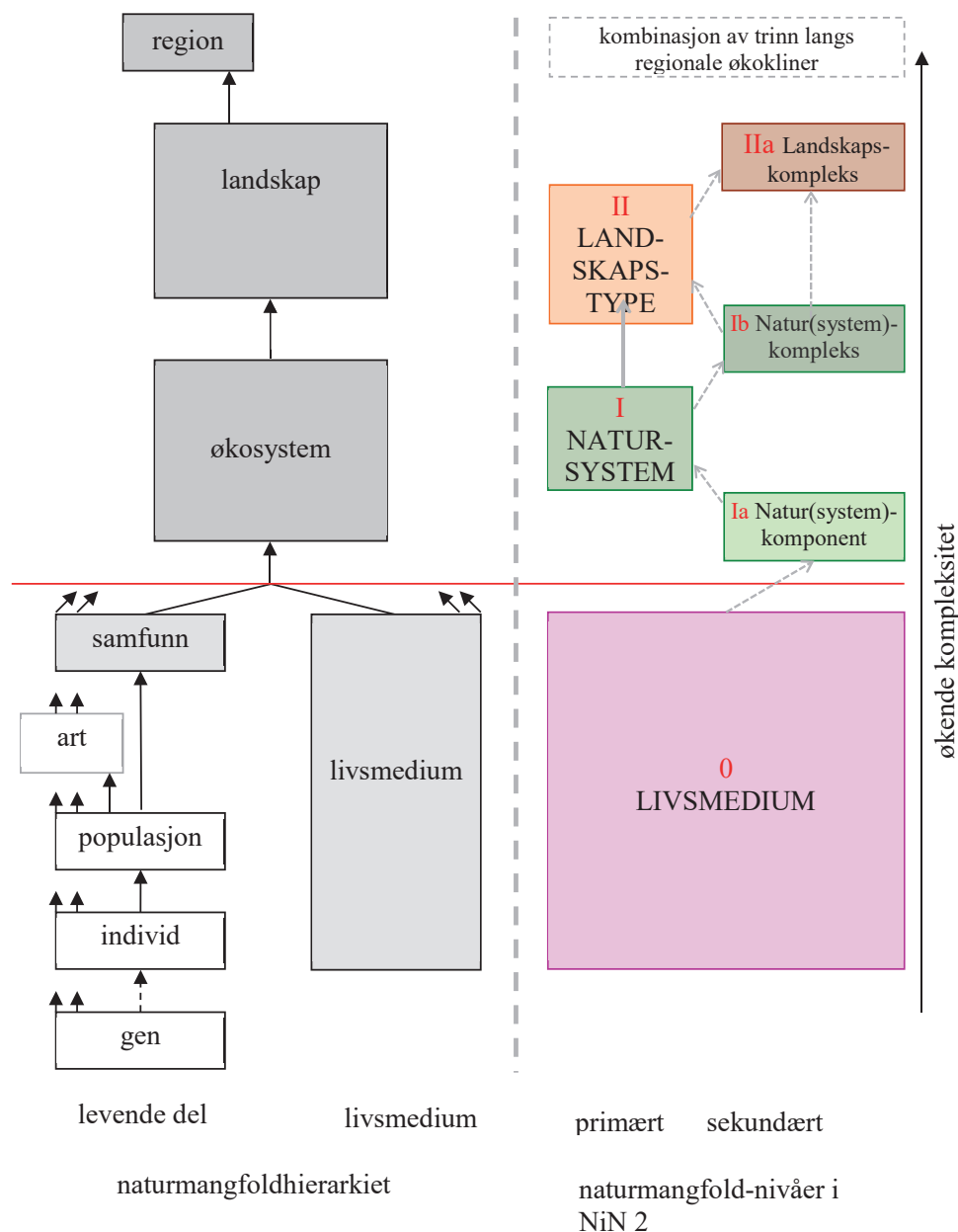
Fig. A2-2. Naturmangfoldhierarkiet, hierarkiet av nivåer for naturmangfold med ulik kompleksitet (venstre del av figuren), og sammenhenger mellom naturmangfoldhierarkiet og naturmangfold-nivåer som det utarbeides typeinndeling og beskrivelsessystem for i NiN 2 (høyre del av figuren). Naturmangfold-nivåene er fordelt på primære og sekundære naturmangfold-nivåer, mens livsmedium-nivået står i en særstilling. Den røde, horisontale streken skiller nivåer der artssammensetningen og miljøfaktorene typeinndeles samlet (over streken) og lavere naturmangfold-nivåer. Naturmangfold-nivåene økosystem og landskap er vist som bokser med stor vertikal utstrekning fordi det trengs flere nivåer enn to for å beskrive all variasjonen innenfor de skalaintervallene disse to nivåene omfatter. Streker mellom naturtypenivåene indikerer relasjoner, dvs. at flere natursystemkomponenter kan inngå i én natursystem-arealenhet, at flere natursystemer kan inngå i én natursystem-kompleks-arealenhet, og at flere landskap kan inngå i én landskapskompleks-arealenhet.
