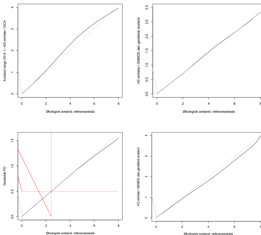
Fig. V3-4. Økologisk avstand, målt som avstand mellom par av OEer langs en ordinasjonsakse, som funksjon av kjent økologisk avstand for fire kombinasjoner av ordinasjonsmetode og simulert datasett. Enheter for økologisk avstand er S.D.-enheter som er resultatet av ikke-lineær reskalering av DCA-akser, og H.C.-enheter som opptrer i GNMDs, med eller uten step across. Referanseskalaen for avstand langs en underliggende gradient er en skalering i tilfeldige enheter som ikke er sammenliknbare mellom datasettene. Alle gradienter er regelmessig samlet med 41 observasjonseenheter (se Tabell V2-3 for datasettdetaljer). Røde, stiplede linjer angir PD50, punktet langs gradienten er PD mellom par av OEer = 0,5. (a) DCA-avstander skalert i S.D.-enheter, Datasett 0. (b) GNMDs-avstander skalert i H.C.-enheter, uten step across, Datasett 0. (c) GNMDs-avstander skalert i H.C.-enheter, med step across, Datasett 0. (d) GNMDs-avstander skalert i H.C.-enheter, uten step across, Datasett B.
