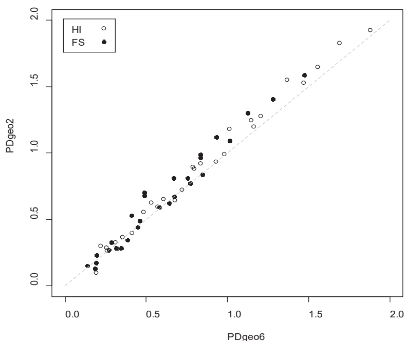
Fig. V4–6. Sammenheng mellom PDgeo, beregnet på grunnlag av mengdeangivelse henholdsvis på den standard 6-trinnskalaen (horisontal akse) og på den forenklete 2-trinnskalaen (vertikal akse), for 28 par av observasjonseenheter (alle kombinasjoner av 8 enkeltobservasjonseenheter) i hvert av de to datasettene HI og FS.
