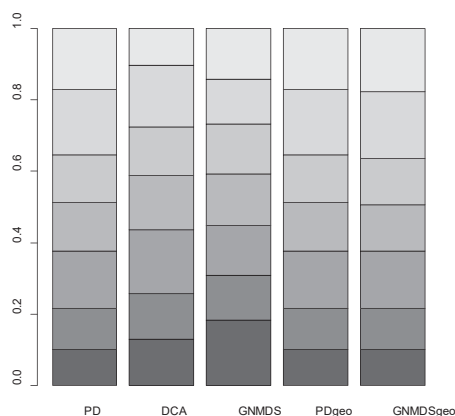
Fig. V4-3. Sammenlikning mellom fem mål på relativ økologisk avstand (ØA) mellom nabotrinn langs LKM hevdintensitet (HI). Relativ ØA er ØA-verdien mellom ett par av nabotrinn uttrykt som andel av summen av ØA-verdier for alle de sju nabotrinnene. Trinnparene fra 1–2 til 7–8 opptrer fra nederst til øverst i hver søyle.
