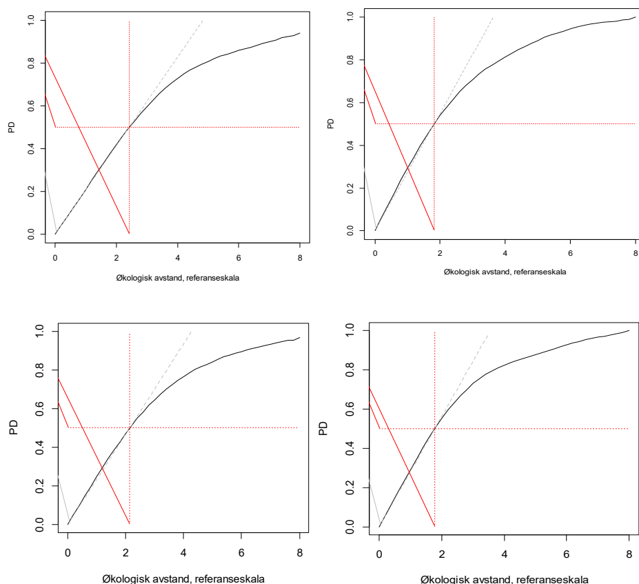
Fig. V3-1. PD som funksjon av økologisk avstand for fire simulerte datasett. Økologisk avstand er angitt som avstand langs en underliggende gradient, skalert i tilfeldige enheter som ikke er sammenliknbare mellom datasettene. Alle gradienter er regelmessig samlet med 41 observasjonseenheter (se Tabell V2-3 for datasettdetaljer). Røde, stiplede linjer angir PD50, punktet langs gradienten der PD mellom par av OEer = 0,5. (a) Datasett 0. (b) Datasett B. (c) Datasett C. (d) Datasett D.
