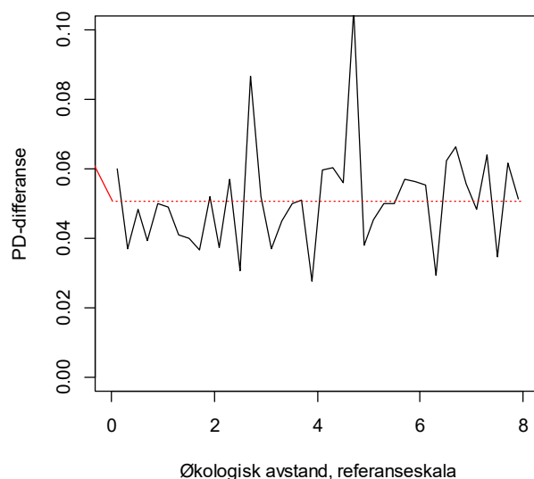
Fig. V3-2. PD-differanse mellom nabotrinns (økologisk avstand = 0,2 XD-enheter) som funksjon av plassering langs den 'underliggende' gradienten. Simulert datasett D. Artstettheten avtar fra 39 ved X = 0 til 17 ved X = 8
