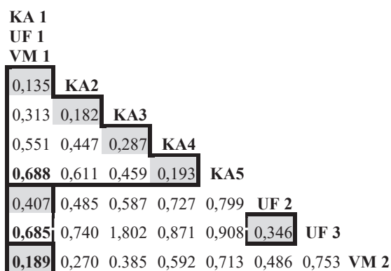
Fig. V4-4. Ulikhetsmatrise mellom de åtte observasjonsenhetene i Datasett FS som representerer variasjon langs de tre LKM kalkinnhold (KA) med fem trinn, uttørkingsfare (UF) med tre trinn og vannmetning (VM) med to trinn. Ulikhetsmatriser for hver av de tre gradientene er markert med svart, tjukk strek. PD (proportional dissimilarity) er benyttet som ulikhetsmål. PD-verdier mellom nabo-observasjonsenheter langs gradienten er markert med grå celler.
