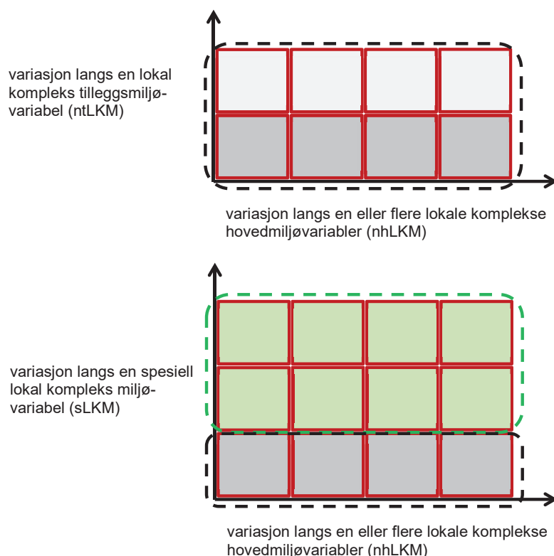
Fig. B4–1. Begrepene som brukes til å beskrive variasjon langs lokale komplekse miljøvariabler og deres relevans for inndeling av en natursystem-hovedtypegruppe i hovedtyper. Den øverste figuren illustrerer begrepet normal variasjonsbredde, som først og fremst beskrives av en hovedkompleksmiljøvariabelgruppe bestående av normale lokale komplekse hovedmiljøvariabler (nhLKM), det vil si LKM som 'forklarer' mer variasjon i artssammensetning enn 2 ØAE mellom tyngdepunkter for naturtyper innenfor en hovedtypegruppe. I den øverste figuren består hovedkompleksmiljøvariabelgruppa av én nhLKM med fire standardtrinn, hvert trinn illustrert som én 'boks' med grå bunnfarge, plassert langs den horisontale akse. Dersom hovedkompleksmiljøvariabelgruppa inneholder flere enn én nhLKM, trengs flere dimensjoner (et flerdimensjonalt rom) for å beskrive denne variasjonen. Den øverste figuren illustrerer situasjonen der det innenfor én eller flere 'bokser' langs nhLKM finnes variasjon langs en LKM som i utgangspunktet ikke behøver tilhøre normal variasjonsbredde, men som bare 'forklarer' mellom 1 og 2 ØAE mellom typiske naturtype-utforminger (illustrert som 'bokser' på lys grå bunn). Denne LKM er da en normal lokal kompleks tilleggsmiljøvariabel (ntLKM), og gir ikke grunnlag for å opprette ny hovedtype som skal skilles fra hovedtyper for den normale variasjonsbredden (svart stiplet linje omfatter den normale variasjonsbredden). Den nederste figuren illustrerer situasjonen der det finnes variasjon langs en LKM som ikke ligger innenfor normal variasjonsbredde, men hvor denne variasjonen 'forklarer' over 2 ØAE. Da blir denne LKM en spesiell lokal kompleks miljøvariabel (sLKM), som blir en definerende lokal kompleks miljøvariabel som gir grunnlag for å skille ut en spesiell hovedtype fra normal variasjon innenfor ei hovedtypegruppe (variasjonsbredden som omfattes av hovedtypen for spesiell variasjon er illustrert med grønn stiplet linje).
