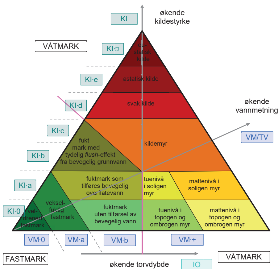
Fig. B3-12. Vanntilgangstrekanter, en begrepsmodell som viser de komplekse relasjonene mellom de tre vannrelaterte lokale miljøgradientene (LKM'ene) i NiN versjon 2: vannmetning (VM), som adresserer den generelle vanntilførselsstyrken og som i våtmarkssystemer erstattes av tørleggingsvarighet (TV), som angir avstanden til grunnvannsspeilet (fra tuenivå til mykmatte), samt kildevannspåvirkning (KI), som angir i hvilken grad tilført vann er grunnvann med kildevannsegenskaper. Miljøgradienten innhold av organisk materiale (IO) angir tendensen til torvdannelse og overgangen mot myr og kilde, og mellom disse. LKM er indikert med tykke, grå piler i figuren. Lilla linjer markerer grensa mellom fastmarkssystemer og våtmarkssystemer. Basistrinninndelingen av VM og KI er vist langs kanten av trekanten. Den spisse vinkelen mellom VM- og KI-vektorene viser at de to variablene er sterkt korrelert med hverandre. Merk: Lengden på trekantens sidekanter gjenspeiler ikke graden av endring i artssammensetning eller andre aspekter av naturvariasjon langs økoklinene.
