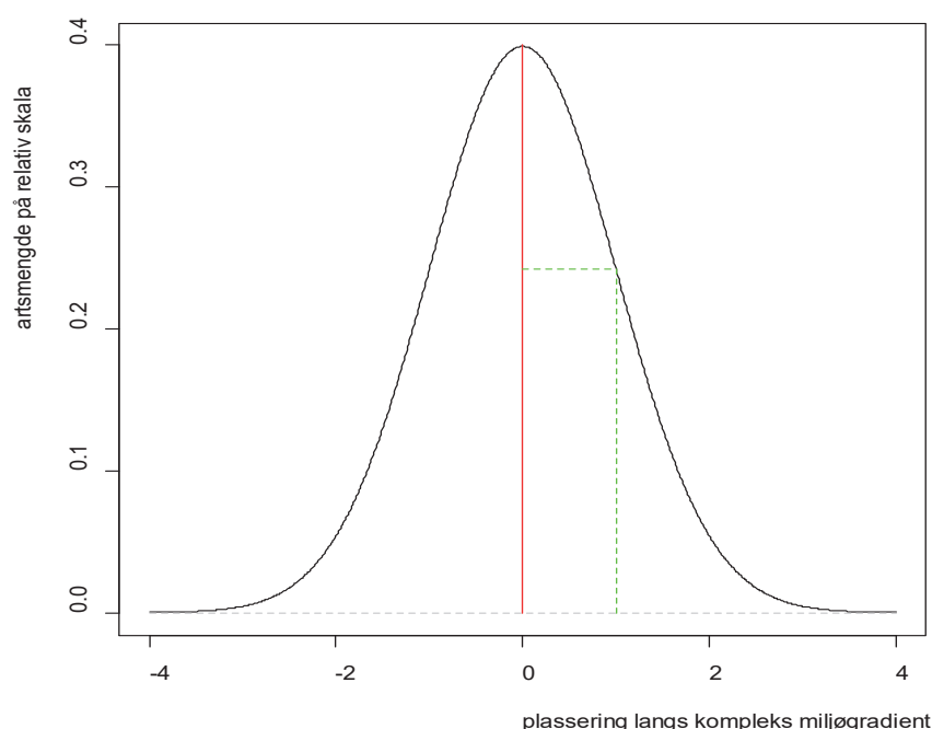
Fig. V2-2. Punktsannsynligheten i normalfordelingen med middelvei = 0 og standardavvik = 1, tolket som artsresponskurve på en underliggende kompleks miljøgradient, skalert i S.D.-enheter. Den røde linja markerer en gjennomsnittsarts optimum, den grønne stiplete linja markerer standardavviket i fordelingen.
