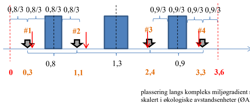
Fig. B2-4. Eksempel som illustrerer beregning av gradientlengde på grunnlag av estimerte økologiske avstander. Typiske utforminger av de fire naturtypekandidatene (#1, #2, #3 og #4, markert med oransje numre), som hver er representert med ei generalisert artsliste, plasserte seg langs den aktuelle komplekse miljøgradienten der pilene som peker ned mot tallinja viser. Parvise økologiske avstander ble beregnet ved bruk av PDgeo. Grenser mellom nabo-typekandidater, trukket midt mellom plasseringen av de typiske utformingene, er vist med tynne, brutte vertikale streker. Overgangsintervallet mellom nabo-naturtypekandidater, som har en utstrekning på 1/3 av den økologiske avstanden mellom naturtypekandidatene – 1/6 på hver side av grensa – defineres ikke å inngå i den ‘typiske utformingen’ av naturtypekandidaten (det vil si ikke å være ‘representativ for naturtypens miljøvariasjonsbredde’). Den typiske utformingen av endetrinnsnaturtypekandidatene plasseres midt i et intervall som ikke inneholder overgangsintervallet. Gradient-endepunktene plasseres seg dermed 0.8/3 \approx 0.3 ØAE utenfor den typiske utformingen av #1 og 0.9/3 = 0.3 ØAE utenfor den typiske utformingen av #4, og gradientlengden blir 3,6 ØAE. Plassering av gradientendepunkter og naturtypekandidatenes typiske utforminger langs en gradient etter re-skalerting til endepunkter 0 og 3,6 er vist med røde og oransje tall. Naturtypekandidatenes tyngdepunkt er angitt med røde piler.
