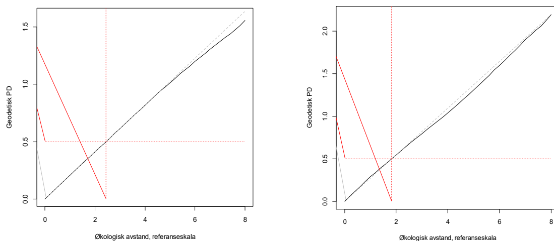
Fig. V3–3. PDgeo som funksjon av økologisk avstand for to simulerte datasett. Økologisk avstand er angitt som avstand langs en underliggende gradient, skalert i tilfeldige enheter som ikke er sammenliknbare mellom datasettene. Alle gradienter er regelmessig samlet med 41 observasjonseenheter (se Tabell V2–3 for datasettdetaljer). Røde, stiplede linjer angir PDgeo50, punktet langs gradienten er PDgeo mellom par av OEer = 0,5. (a) Datasett 0. (b) Datasett B.
