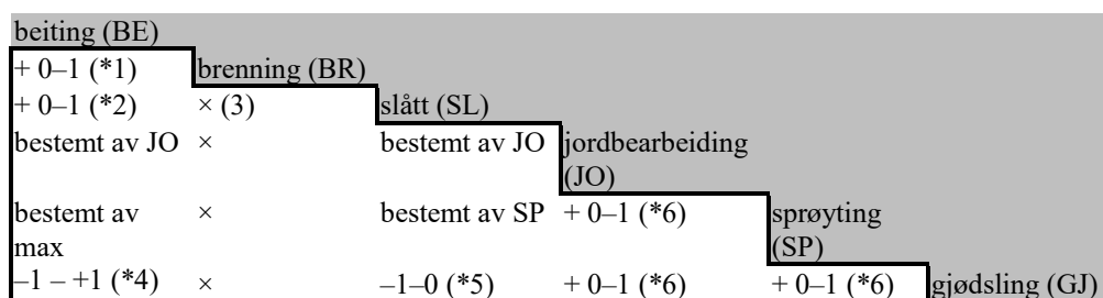
Fig. B3–5. Fordeling av hevdregimer bestående av en kombinasjon av to hevdformer på trinn langs den komplekse miljøgradienten hevdintensitet (HI), definert i henhold til Tabell B3–1. For hevdformer som ikke kan utgjøre et hevdregime alene, er hevdintensiteten angitt som potensiell effektendring (+ angir høyere og – angir lavere trinn) når hevdformen kombineres med andre hevdformer. (*n) er henvisninger til kommentarer.
