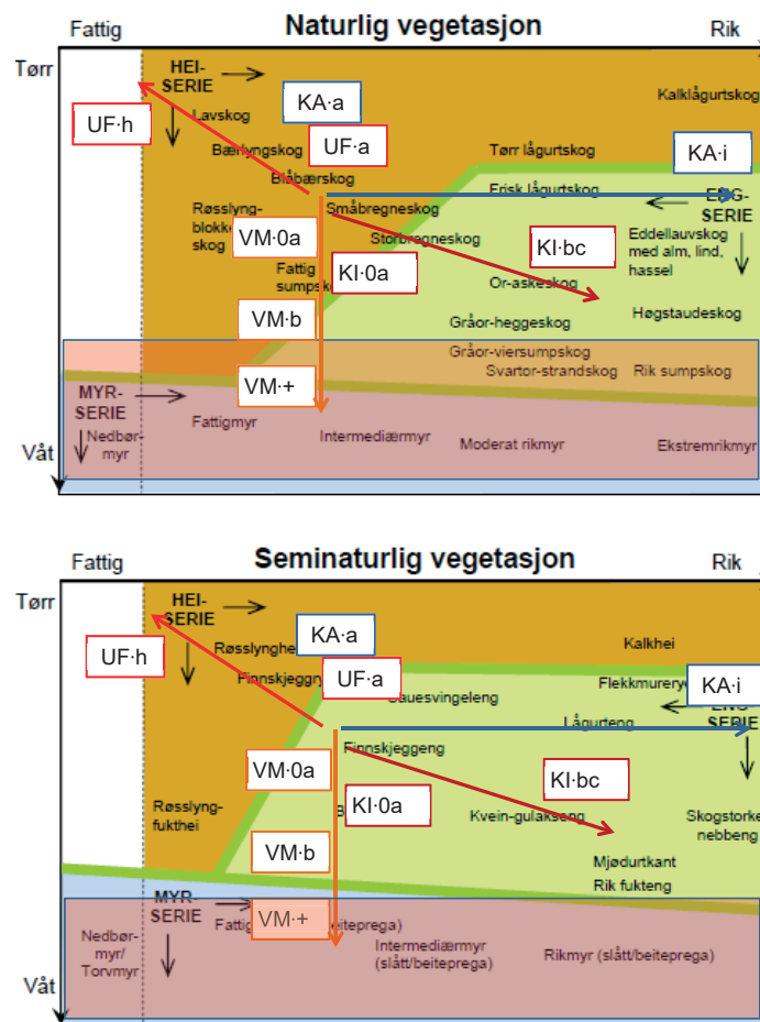
Fig. B3-14. Vektorer som for hver av de fire viktige LKM'ene kalkinnhold (KA), uttørkingsfare (UF), vannmetning (VM) og kildevannspåvirkning (KI) viser hvilken hovedretning de utspenner i figurer der naturlige og semi-naturlige vegetasjonstyper er fordelt på de tre seriene hei, myr og eng og plassert i forhold til forskjeller i fuktighet (tørr–våt) og tilgjengelig mineralnæring (fattig–rik) (Øien & Moen 2006; etter Moen 1998b). Brun farge viser heiserien, blå farge viser myrserien og grønn farge viser engserien.
