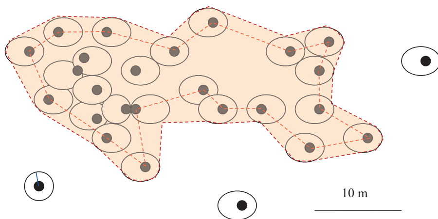
Fig. B3–10. Definisjonsmessig avgrensning av tresatt areal (stiplet mørk rød linje). Alternativt kunne tresatt areal vært definert ved å trekke linjer mellom stammesentrer. Trær er vist som svarte prikker, kroneperiferien som svart ellipse. Kroneradius er vist som blå linje for treet nederst til venstre i figuren.
