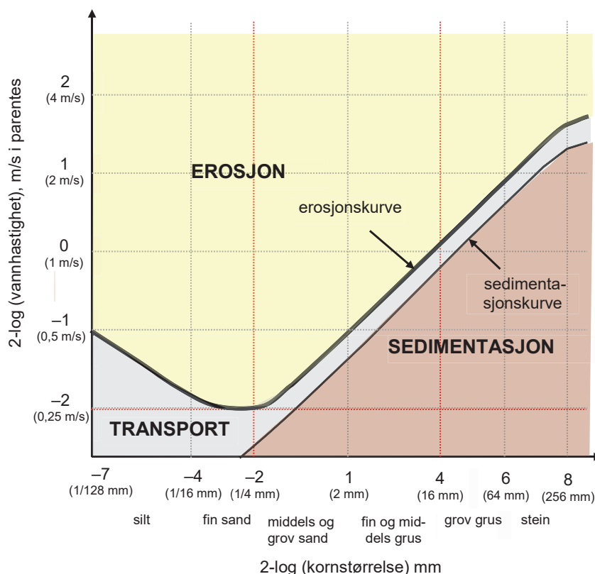
Fig. B3–8. Sammenhengen mellom vannhastighet og kornstørrelse, som bestemmer erosjon, transport og sedimentasjon av elvemateriale, basert på Hjulström (1935, 1939), Sundborg (1956), Sulebak (2007) og Dingman (2009). Gapet mellom sedimentasjons- og erosjonsfeltene i figuren illustrerer at større krefter må til for å sette partikler i bevegelse (erosjon) enn for å holde dem i bevegelse (transport). Formen på erosjonskurven er et resultat av at det er to ulike typer krefter som bidrar til å holde materiale fast på elvebunnen – kohesjon mellom små partikler (som avtar når partikkelstørrelsen øker) og press fra vann i bevegelse (som øker når partikkelstørrelsen øker). Sedimentets totale holdfasthet (dets kritiske skjærstyrke) er lavest for fin sand fordi kohesjonskreftene da er små samtidig som partiklene har lav vekt. Fin sand eroderes ved en vannhastighet omkring 0,2 m/s. Sedimentasjonskurven bøyer av (blir brattere) mot svært lave vannhastigheter fordi leire og fin silt bare sedimenteres når det er mer eller mindre strømsstille (< 0,01 m/s). Skalaen på y-aksen er basert på vannhastigheter for ei elv som er ca. 1 m dyp. Sedimenter med gitt kornstørrelse eroderes ved lavere vannhastigheter i grunnere elver, samtidig som grunnere (mindre) elver ikke frambringer vannhastigheter som er høye nok til å erodere grove sedimenter.
