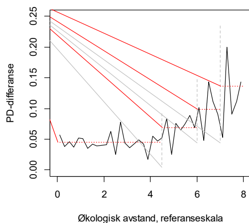
Fig. V3–6. Forskjell i PD mellom trinn langs en gradient simulert med et artsuttynningsintervall som starter ved posisjonen X = 4,5 og fortsetter mot høyere verdier av økologisk avstand. Røde stiplete linjer angir middelverdien for PD-forskjell i fire ulike intervaller langs gradienten, adskilt av grå, stiplete linjer.
