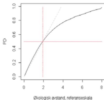
Fig. V3-5. PD som funksjon av økologisk avstand for Datasett U (artsuttynnings-situasjonen). Økologisk avstand er angitt som avstand langs en underliggende gradient, skalert i tilfeldige enheter som ikke er sammenliknbare mellom datasettene. Røde, stiplede linjer angir PD50, punktet langs gradienten der PD mellom par av OEer er lik 0,5.
