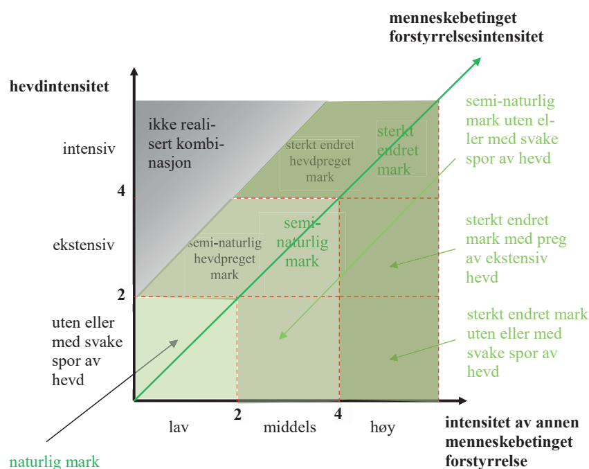
Fig. B3–4. Menneskeforstyrrelsesfirkanten. Begreper knyttet til variasjon i (total) menneskebetinget forstyrrelsesintensitet i grønt. Økende intensitet på den grønne bakgrunnsfargen angir økende (total) menneskebetinget forstyrrelsesintensitet. Figuren viser relasjoner mellom begrepene naturlig mark, semi-naturlig mark og sterkt endret mark og den lokale komplekse miljøgradienten hevdintensitet (HI). Aksene er tentativt skalert i økologiske avstandsenheter (ØAE).
