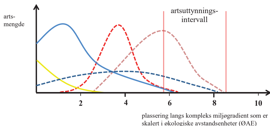
Fig. B2-2. Illustrasjon av en artsutryddingssituasjon, det vil si at det mot en gradient-ende finnes et artsutryddingsintervall; det vil si et punkt utenfor hvilket (det vil si mellom punktet og et gradientendepunkt) ingen arter øker i mengde, men gradvis når sin toleransegrense. Skalaen på y-aksen er en vilkårlig, relativ skala for artsmengde. Den komplekse miljøgradienten (x-aksen) er skalert i økologiske avstandsenheter (ØAE) som er foreslått brukt i NiN versjon 2 (se Fig. B2-1 og teksten). Standard lengde av et artsutryddingsintervall settes til 2.4 ØAE fra optimum for den mest tolerante arten til gradientendepunktet (der ingen arter lenger forekommer stabilt).
