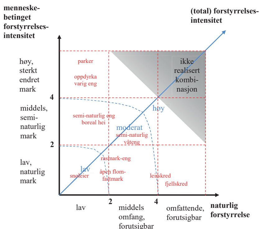
Fig. B3–1. Den generelle forstyrrelsesfirkanten. Omtrentlig plassering av naturtypebegreper (se NiN[2] artikkel 3) i rødt. Begreper knyttet til variasjon i total forstyrrelsesintensitet i blått. Aksene er tentativt skalert i økologiske avstandsenheter (ØAE).
