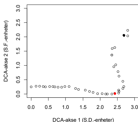
Fig. V3-8. DCA-ordinasjon av de 41 OEene i Datasett U (artsuttynnings-situasjonen). Det røde punktet angir OEen fra punktet X = 4,4 langs gradienten (der arts1uttynningsintervallet starter), det svarte punktet angir gradientendepunktet ( X = 8,0 ).
