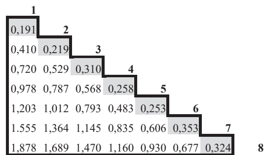
Fig. V4-2. Ulikhetsmatrise mellom de åtte observasjonsenhetene i Datasett HI som representerer trinn langs LKM hevdintensitet (HI). PDgeo ( proportional dissimilarity med step across basert på øvre grense for pålitelige ulikhetsverdier \varepsilon = 0,5 ) er benyttet som ulikhetsmål. PDgeo-verdier mellom naboobservasjonsenheter langs gradienten er markert med grå celler.
