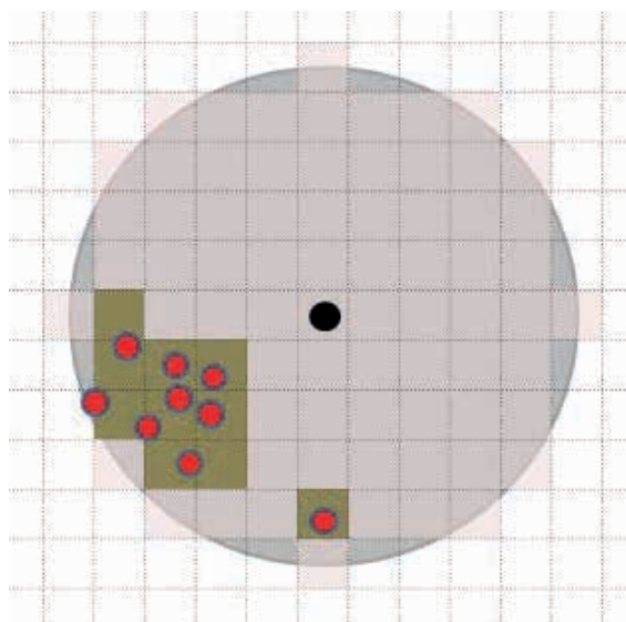
Fig. C2–1. Skisse som viser beregning av nøkkelvariabel av naboskapstypen som frekvens i 81 standardiserte ruter á 100 \times 100 m. De 81 rutene (markert med rosa skygge) ligger helt eller delvis innenfor en sirkel (naboskapssirkelen, markert med grå skygge) med radius 500 m omkring et fokuspunkt, som nøkkelvariabelen blir beregnet for (markert med en svart prikk som er plassert i midten av ei rute). I eksemplet er egenskapen nøkkelvariabelen er basert på (f.eks. forekomst av bygninger) indikert med rød prikk. I dette eksemplet har nøkkelvariabelen verdien 10, eller alternativt 0,123 hvis oppgitt som frekvens.
