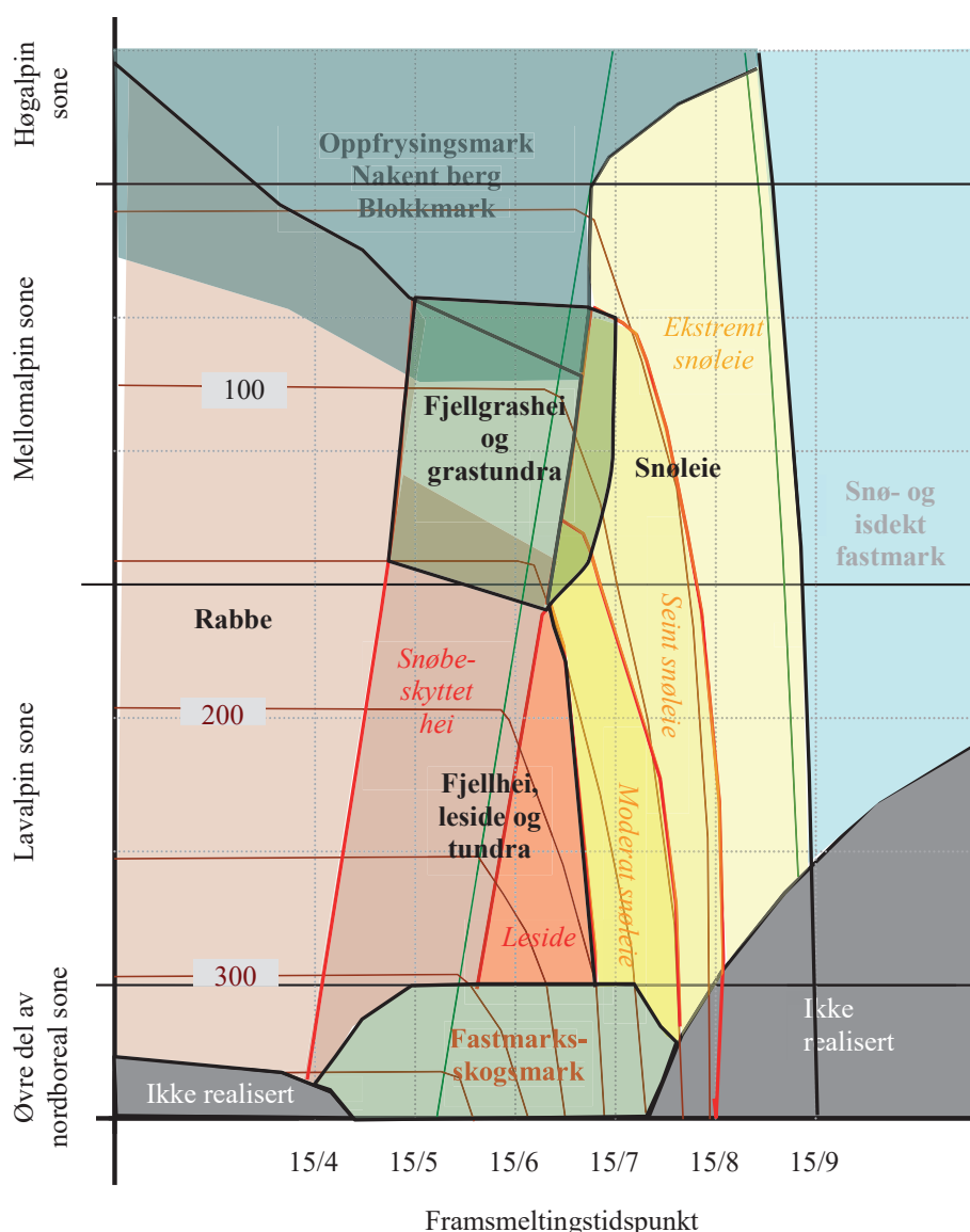
Fig. B3-16. Sonering på fastmark i fjellet på det norske fastlandet relatert til framsmeltingstidspunkt og høyde i forhold til skoggrensa og vedvekstgrensa (mellom mellom- og høg-alpin sone). Trinn langs uttørkingsfare (UF) (innen T3 Fjellhei, leside og tundra) og snødekkebettinget vekstsesongreduksjon (SV) (innen T7 Snøleie) er kursivert. Natursystem-hovedtyper er avgrenset med svarte linjer og navnsatt med fet skrift. Figuren viser hvordan først leside og moderat snøleie, deretter snøbeskyttet hei og seint snøleie fases ut mot høyden fordi kombinasjonene av lang nok vekstsesong og stabilt nok snø-dekke forsvinner. Grønne linjer angir begynnelsen og avslutningen på vekstsesongen. Brune isolinjer angir varmesum (rødbrune tall) i dag-grad-enheter (ddu) med basistemperatur 5 °C (T- 5, summert over alle dager med T, døgnmiddeltemperatur, over 5 °C). Klimadata fra Aune (1993) for Kongsvold (Oppdal, STr, 885 m.o.h.), basert på en vertikal temperaturgradient på -0.5 °C.
