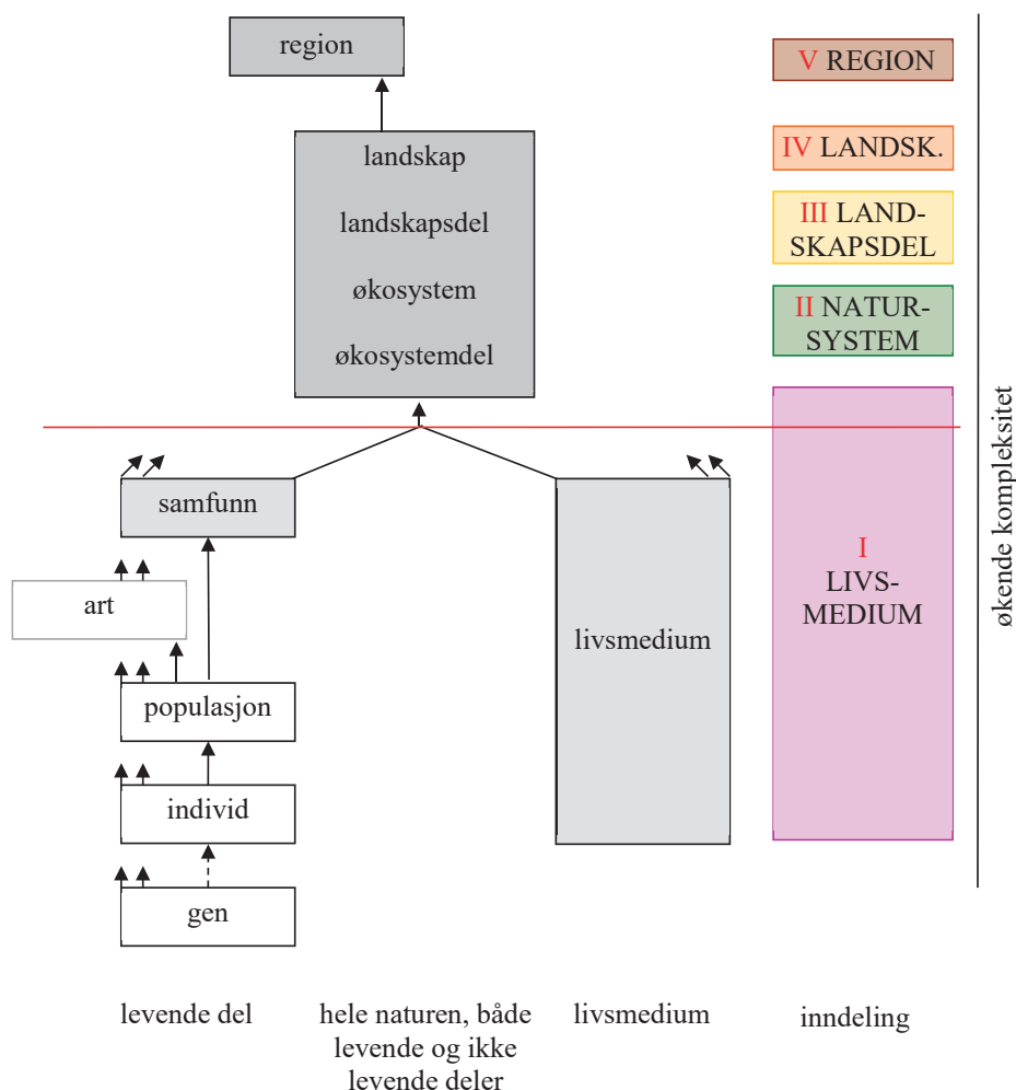
Fig. A1-1. Naturmangfoldhierarkiet, hierarkiet av nivåer for naturmangfold med ulik kompleksitet (venstre del av figuren), og sammenhenger mellom naturmangfoldhierarkiet og de fem naturmangfold-nivåene som var gjenstand for typeinndeling og utarbeidelse av beskrivelsessystem i NiN versjon 1.0 (I-V i høyre del av figuren). Den røde, horisontale streken skiller mellom øko-nivåene der artssammensetningen og miljøfaktorene typeinndeles samlet (over streken) og lavere naturmangfold-nivåer. Naturmangfold-nivåene økosystem og landskap er vist som bokser med stor vertikal utstrekning fordi det trengs flere nivåer enn to for å beskrive all variasjonen innenfor de skalaintervallene disse to nivåene omfatter. Nivåene samfunn og livsmedium, som sammen med øko-nivåene er aktuelle for naturtypeinndeling, er markert med lys grå farge. Den brutte streken i pila mellom gen og individ markerer at det kan skilles ut flere mellomnivåer.
