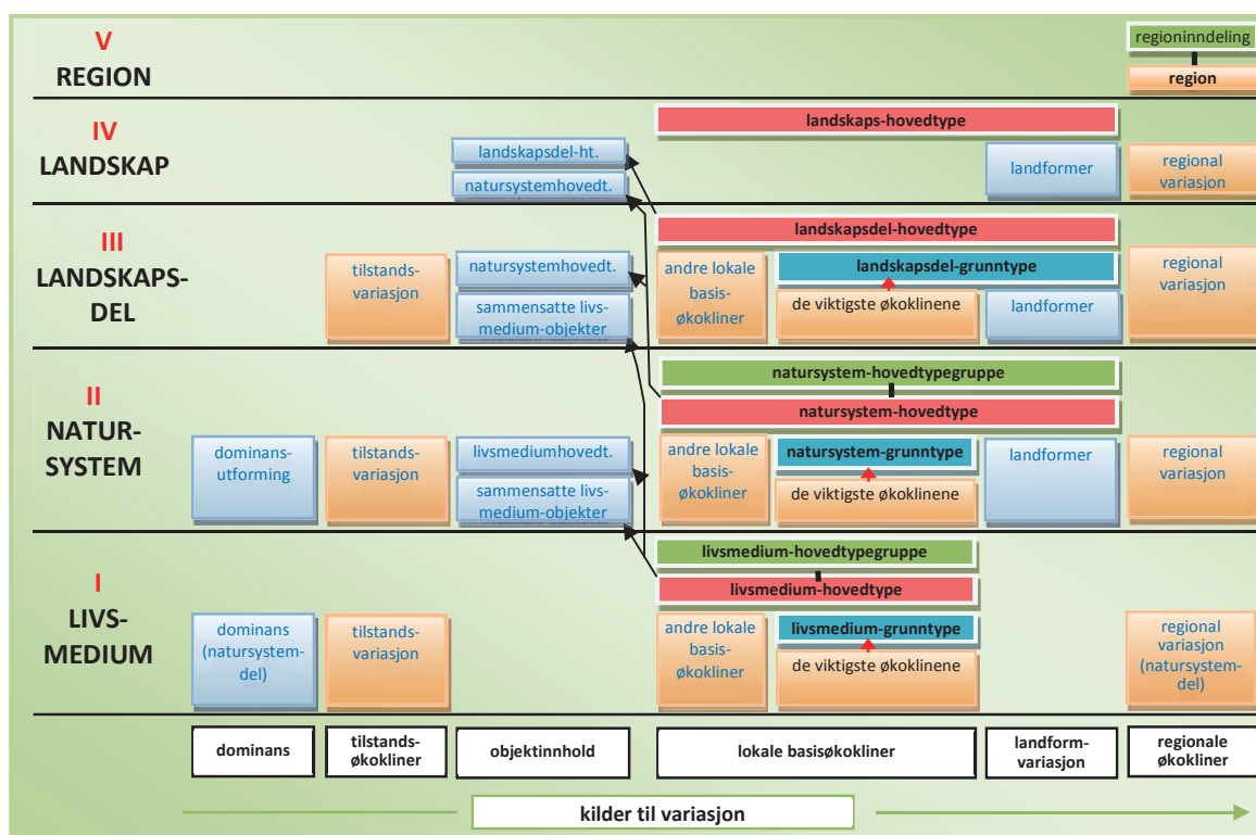
Fig. A2-1. 'Naturtypefiguren' i NiN versjon 1.0, som viser systemets arkitektur: De fem naturmangfold-nivåene NiN 1 inneholder typeinndelinger for er vist på den vertikale aksen (skilt av horisontale linjer). Inndelingen på hvert naturmangfold-nivå inneholder inntil tre generaliseringsnivåer (som er plassert over hverandre mellom de horisontale linjene som avgrenser hvert naturmangfold-nivå). Hovedtypegruppe-nivået er vist som grønne bokser og hovedtypenivået som røde bokser. Variasjon på generaliseringsnivået under hovedtype fanges opp av et beskrivelsessystem som er basert på et standardisert begrepsapparat for seks kilder til variasjon. Dette beskrivelsessystemet har (inntil) tre elementer: (1) inndeling i grunntyper (mørk blå bokser) basert på trinndeling av de viktigste lokale basisøkolinene (oransje bokser med svart skrift); (2) variasjon langs andre økolinier (oransje bokser); og (3) andre kilder til variasjon (lys blå bokser). Kategorien objektinnhold omfatter enheter som er definert ved forekomst av naturtyper på et lavere naturtypenivå (og/eller 'spesielle naturforekomster'), som vist med svarte piler. Bokser omgitt av stiplet linje blir ikke beskrevet eksplisitt i NiN versjon 1, men er i prinsippet relevant for å beskrive variasjon på det aktuelle naturtypenivået.
