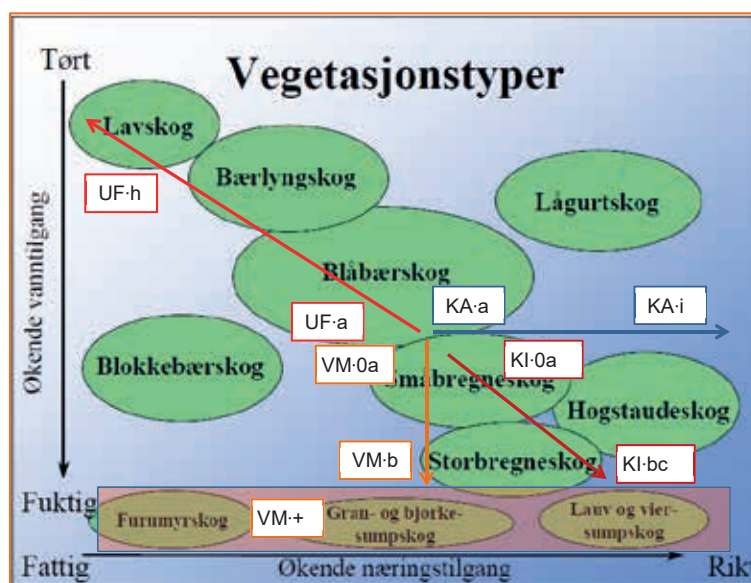
Fig. B3–13. Vektorer som for hver av de fire viktige LKM'ene i skogsmark viser retningen på største variasjon i 'boblediagrammet' der Larsson (2000) plasserer et utvalg av vegetasjonstypene i skog i forhold til tilgangen på vann og næring (gjengitt fra Larsson 2000: iii). KA = kalkinnhold; UF = uttørkingsfare; VM = vannmetning; KI = kildevannspåvirkning. Den spisse vinkelen mellom VM og KI, og mellom KI og KA, indikerer at disse miljøvariablene samvarierer
