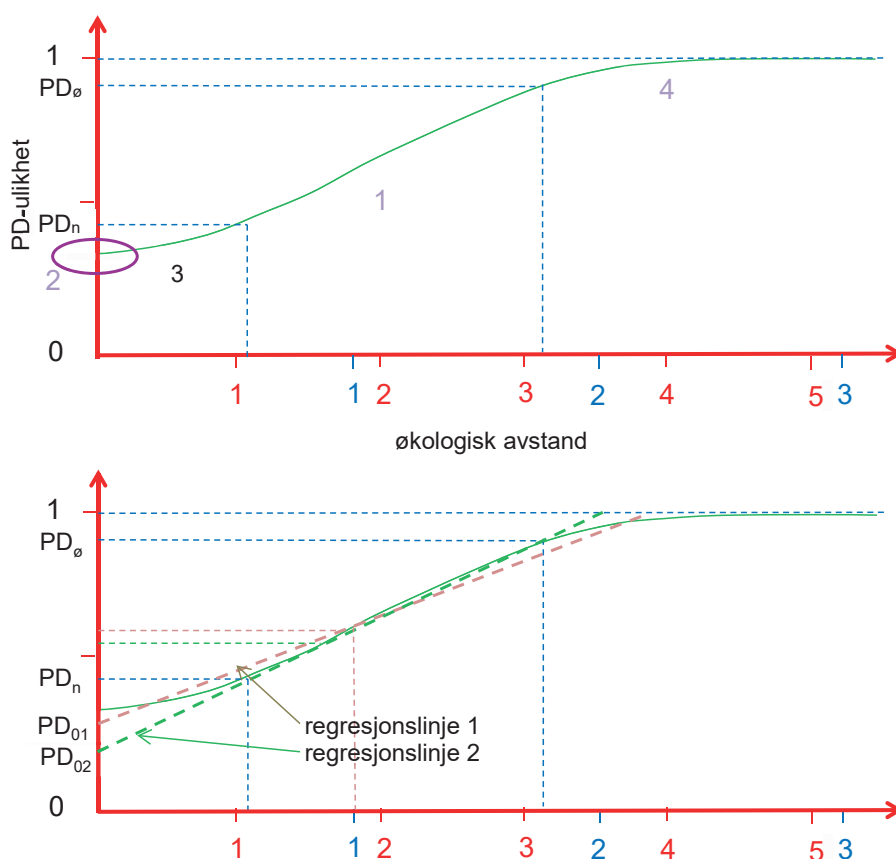
Fig. V2-1. Relasjoner mellom artssammensetningsulikhet (AU) og økologisk avstand (ØA) i konkrete observasjonsdata. Øverst: Illustrasjon av en typisk sammenheng mellom AU og ØA, med de fire utfordringene knyttet til bruk av artssammensetningsulikhet som mål på økologisk avstand indikert med fiolette tall: 1 – at sammenhengen er lineær bare i et begrenset intervall; 2 – at tilfeldig variasjon gjør at ØA = 0 ikke svarer til at AU = 0; 3 – ikke-linearitet mellom AU og ØA når AU er nær ulikheten mellom replikater (UMR); 4 – ikke-linearitet mellom AU og ØA når artssammensetnings-ulikheten er høy. AU er eksemplifisert med ulikhetsmålet proporsjonal dissimilaritet (proportional dissimilarity; PD), men i hovedtrekk vil alle AU-indeks følge samme mønster. To ulike skalerings av ØA-aksen er vist i figuren: skalering i S.D.-enheter (røde tall) og i H.C.-enheter (blå tall). PD n og PD 0 angir nedre og øvre grense for området der PD er lineært relatert til økologisk avstand. Nederst: Grafisk forklaring på H.C.-enheten som brukes til skalering av aksene i NMDS-ordinasjon med R-pakken vegan (Oksanen et al. 2012) (den lysebrune regresjonslinja 1). Den grønne regresjonslinja 2 representerer en alternativ definisjon av H.C.-enheten (se teksten). PD 01 og PD 02 er skjæringspunkter med y-aksen (se forklaring i teksten).
