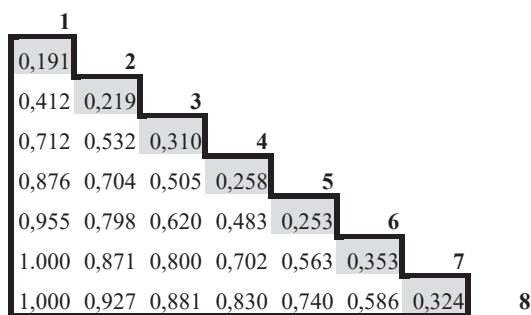
Fig. V4-1. Ulikhetsmatrise mellom de åtte observasjonsenhetene i Datasett HI som representerer trinn langs LKM hevdintensitet (HI). PD ( proportional dissimilarity ) er benyttet som ulikhetsmål. PD-verdier mellom naboobservasjonsenheter langs gradienten er markert med grå celler.
