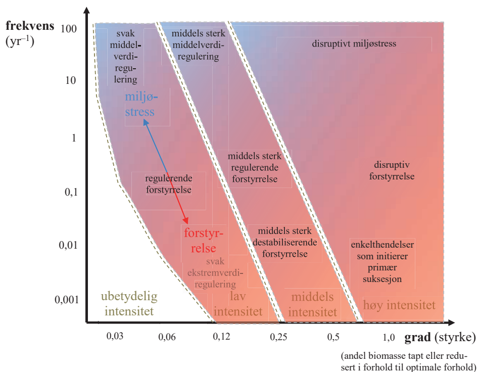
Fig. B3-2. Sammenheng mellom grad (styrke) av påvirkninger utenfra som artene har begrenset toleranse overfor, disse påvirkningenes frekvens og den samlede intensiteten av slike påvirkninger. Graden (styrken) av påvirkninger utenfra er angitt som andelen av den totale biomassen som går tapt i en forstyrrelsesbegivenhet eller reduksjonen i produktivitet som skyldes miljøstress i forhold til produktiviteten under optimale forhold, når alle andre miljøforhold enn den aktuelle påvirkningen holdes konstante. Brutte linjer skiller mellom fire nivåer av total påvirkningsintensitet: ubetydelig, lav, moderat og høy intensitet. Gradienten i dominerende prosess fra forstyrrelse (ekstremverdiregulering) til miljøstress (middelverdiregulering) er angitt som en gradient fra rød til blå bakgrunnsfarge. Begreper som beskriver ulike intensiteter av forstyrrelse og miljøstress er også vist i figuren.
