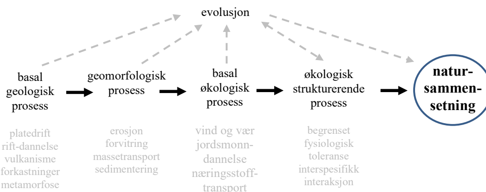
Fig. A1–2. Relasjon mellom ulike naturprosesser som gir opphav til variasjon i natursammensetning. Eksempler på hver av naturprosessene er angitt med grå skrift. Pilene mellom evolusjon og de andre prosessene angir hovedretningen for hvordan de påvirker hverandre.
