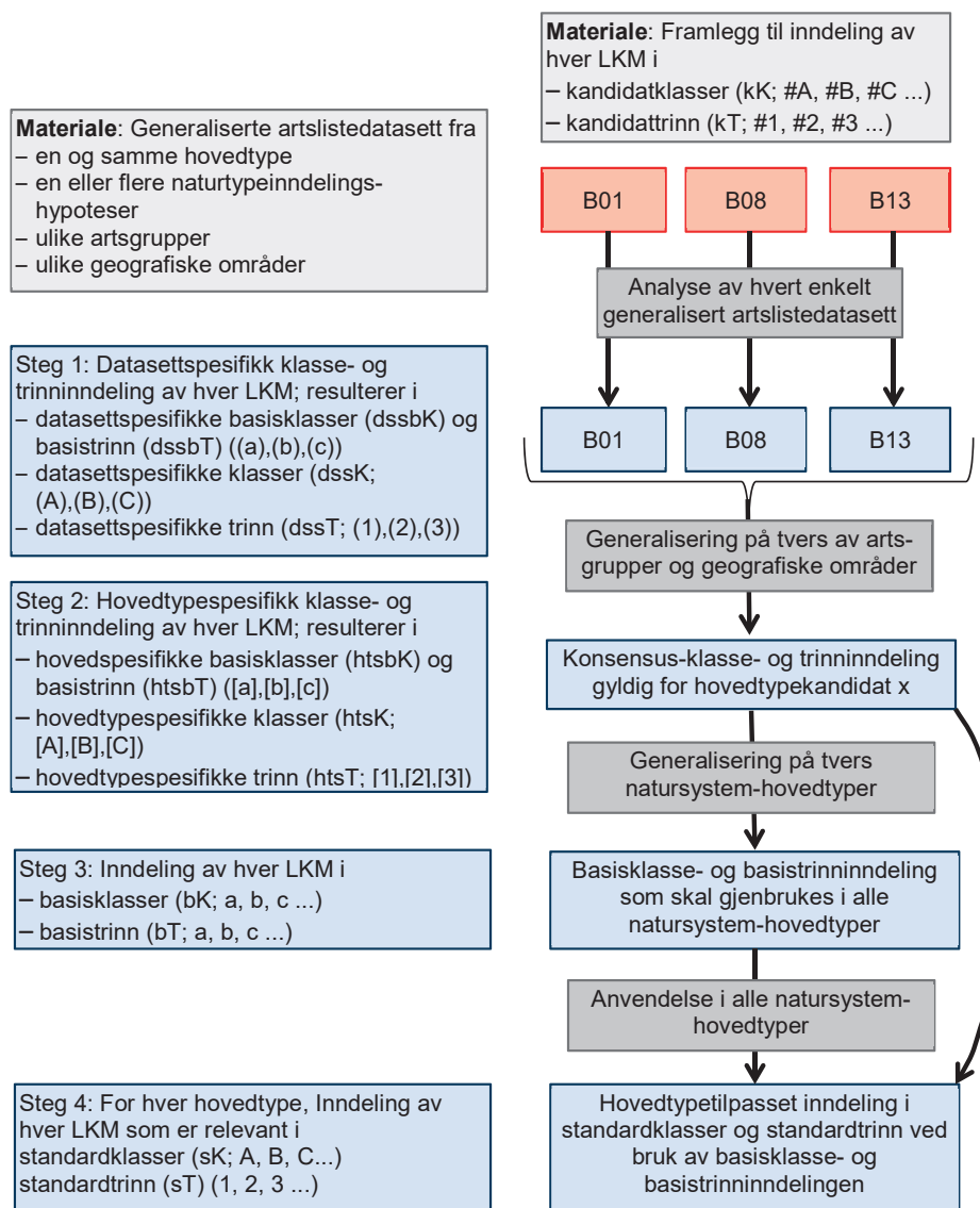
Fig. B2–3. Skjematisert oversikt over fire-stepsprosedyren fra analyse av generaliserte artslistedata til hovedtypetilpasset klasse- og trinndeling av komplekse miljøvariabler. Forkortelser av, og notasjon for, viktige begreper er også vist.
