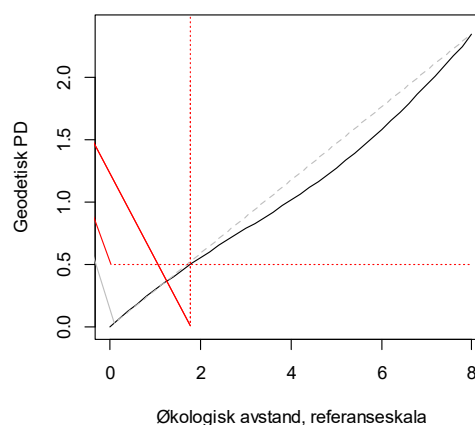
Fig. V3–7. PDgeo som funksjon av økologisk avstand for Datasett U (artsuttynnings-situasjonen). Økologisk avstand er angitt som avstand langs en underliggende gradient, skalert i tilfeldige enheter som ikke er sammenlignbare mellom datasettene. Røde, stiplete linjer angir PD50, punktet langs gradienten er PD mellom par av OEer er lik 0,5.
