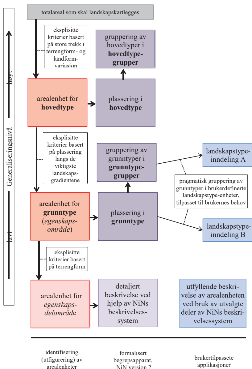
Fig. C1-1. Prinsippkisse for relasjoner mellom ulike faser i landskapskartleggings- og landskapstypifiseringsprosessen. Venstre søyle viser utfigurering av arealenheter, midtre søyle viser typifisering etter NiN versjon 2 (tilordning av arealenheterne til hovedtypegruppe, hovedtype og grunntype), og høyre søyle viser verktøy for brukertilpasset landskapsbeskrivelse.
