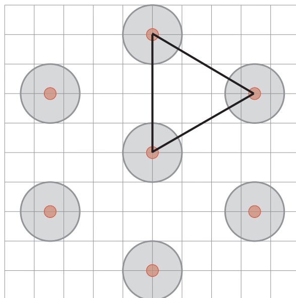
Fig. B3–9. Illustrasjon av hvordan tretetthet kan uttrykkes som arealandel innenfor kroneperiferi på grunnlag av målinger av gjennomsnittlig avstand mellom stammesentre for nabotrær målt i kroneradius-enheter ( g ). Skissen viser en skog med regelmessig plasserte trær, alle like store, og avstand mellom stammesentre lik 4 kroneradius-enheter ( g = 4 ). 22.7 % av arealet innenfor den avgrensede trekanten ligger innenfor kroneperiferien til de tre hjørnetrærne (se teksten). Rød prikk = trestamme, grå sirkel om rød prikk, idealisert kroneperiferi med radius lik gjennomsnittet av kroneradier målt i ulike himmelretninger.
