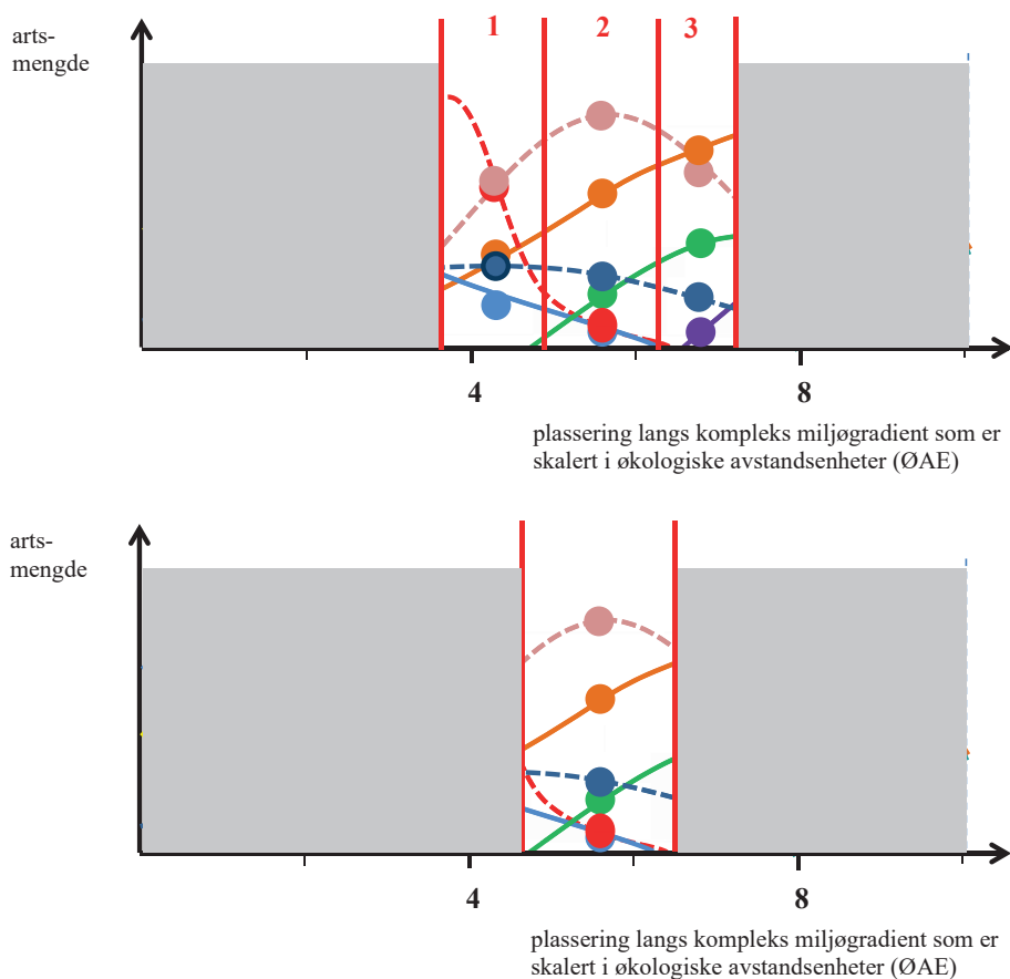
Fig. B2-6. Prinsipp for standardisert trinndeling av lokale kompleks miljøgradient uten behov for hovedtypespesifikk tilpasning. (A, øverst) Lokal kompleks miljøgradient med et omfang av variasjon i artssammensetning, f.eks. innen en hovedtype, på 3,4 ØAE og som derfor skal deles i tre standardtrinn 1–3. Standardtrinnene er skilt av røde vertikale linjer og nummerert med røde tall. Forventet mengde av hver art i typisk utforming for hvert trinn er angitt med prikk i samme farge som artenes responskurve. (B, nederst) Lokal kompleks miljøgradient med et omfang av variasjon i artssammensetning, f.eks. innen en hovedtype, på 1,8 ØAE og som derfor ikke skal trinndeles.
