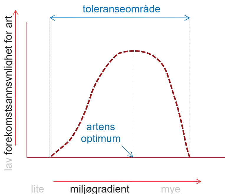
Fig. A1-4. Den unimodale (entoppete) artsresponsmodellen: Arters respons på viktige komplekse miljøgradienter følger vanligvis i store trekk en klokkeformet kurve
