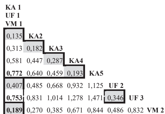
Fig. V4-5. Ulikhetsmatrise mellom de åtte observasjonsenhetene i Datasett FS som representerer variasjon langs de tre LKM kalkinnhold (KA) med fem trinn, uttørkingsfare (UF) med tre trinn og vannmetning (VM) med to trinn. Ulikhetsmatriser for hver av de tre gradientene er markert med svart, tjukk strek. PDgeo (proportional dissimilarity med step across basert på øvre grense for pålitelige ulikhetsverdier \varepsilon = 0,5 ) er benyttet som ulikhetsmål. PDgeo-verdier mellom naboobservasjonsenheter langs gradienten er markert med grå celler.
