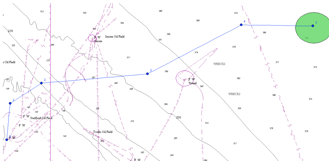
Figur 3. Sleperute fra Statfjord A, detaljer.
