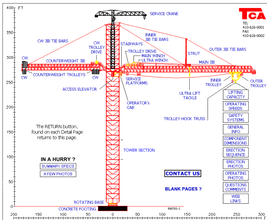
Figur 22. TCA tårnkran
