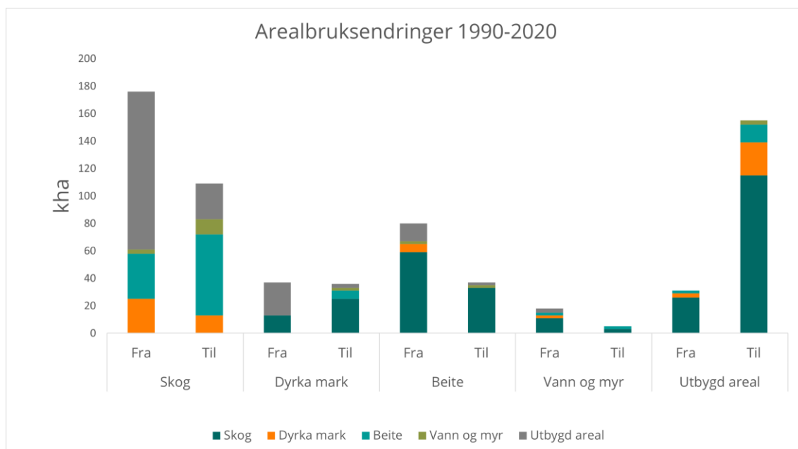
Figur 5: Arealbruksendringer i Norge fra 1990 til 2020 i kilohektar (kha). "Fra"-søylene viser arealer som er tapt fra kategorien, og fargene representerer hva arealene er gått til. For skog viser denne søylen avskogingen i perioden (se første søyle fra venstre). "Til"-søylene viser arealer som er kommet til kategorien, og her representerer fargene hvilken kategori arealene kommer fra. For skog viser denne søylen påskogingen i perioden. Kun arealbruksendringer er med i figuren. Arealer som ikke har endret bruk, er utelatt. Disse er vesentlig større enn endringene for den enkelte kategori. Kilde: Beregnet basert på Miljødirektoratet mfl. (2022).
