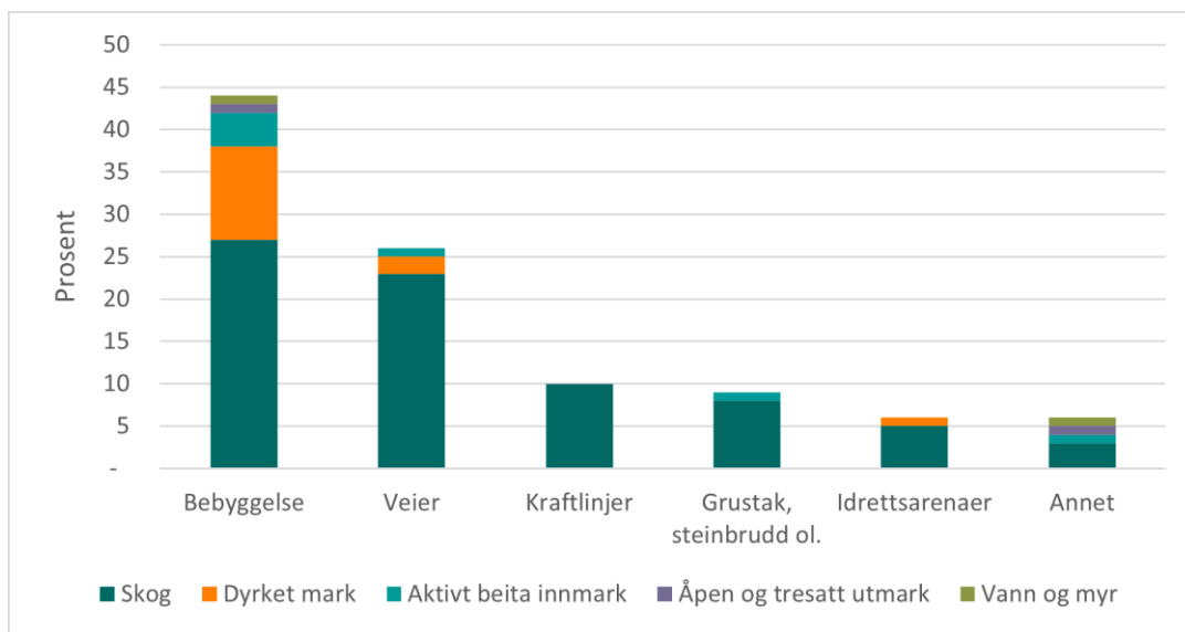
Figur 7. Nedbygget areal 1990-2019 fordelt på opprinnelig arealkategori og type nedbygging. Prosent. Kilde: Søgaard mfl. 2021.
