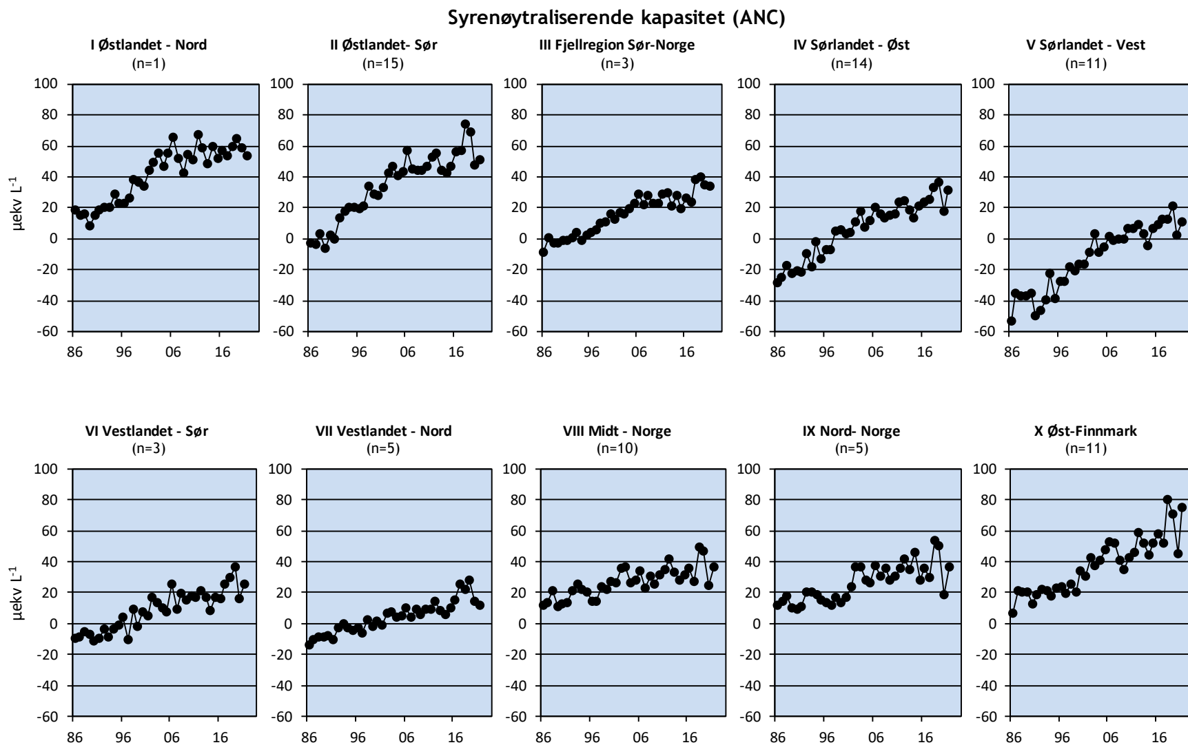
Figur 6. Årlige gjennomsnittsverdier av syrenøytraliserende kapasitet (ANC) i innsjøene for hver av de 10 regionene. Enhet: \mu\text{ekv L}^{-1} . n angir antall innsjøer i hver region.
