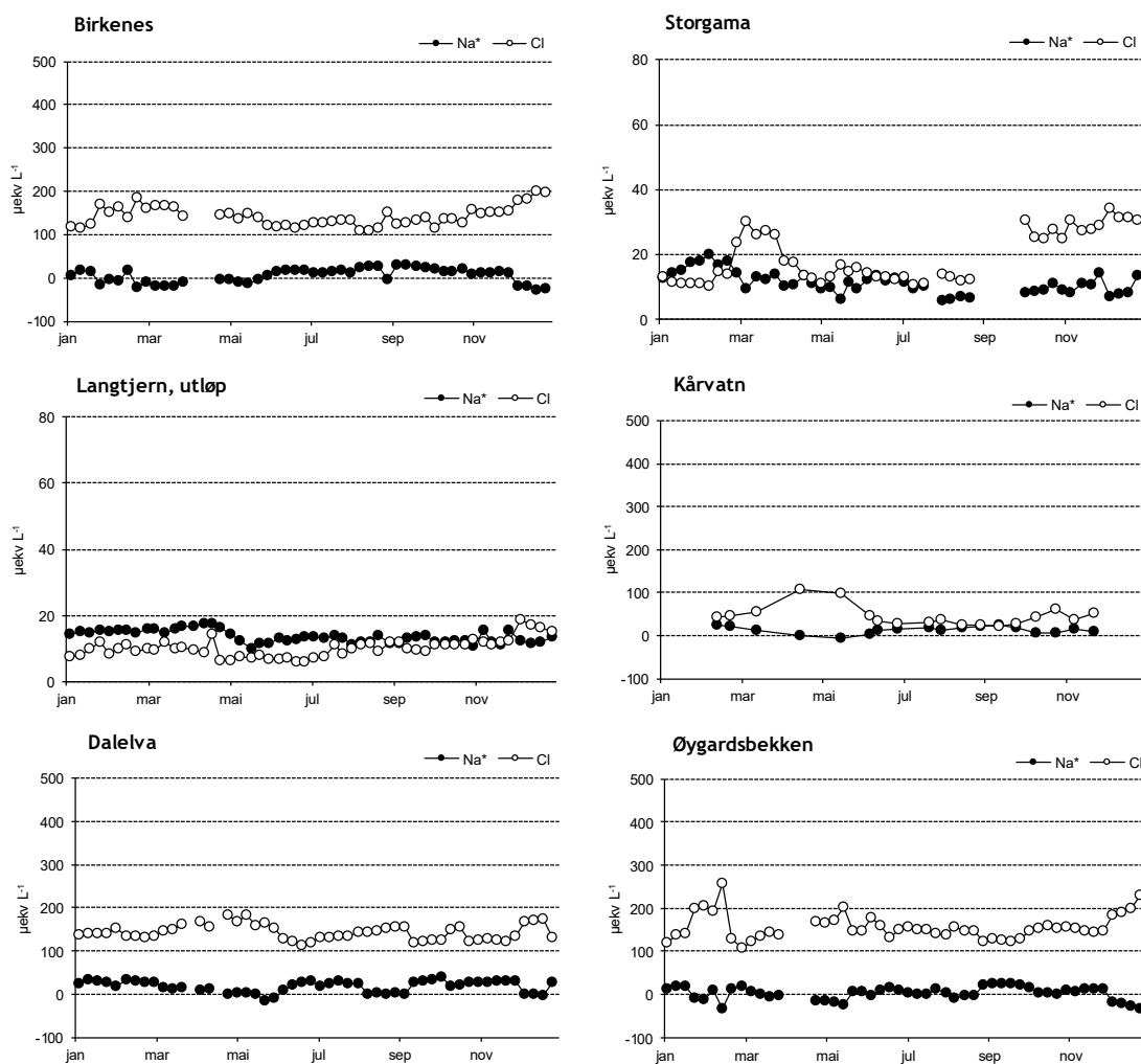
Figur 16. Sesongmessig fluktuasjoner i konsentrasjonene av ikke-marin natrium (Na + ) og klorid (Cl - ) på feltforskningsstasjonene i 2021. Na + ● og Cl - ○. NB! Ulik skala på y-aksene. Enhet: µekv L -1 . Negativ Na + tolkes som at natrium holdes tilbake i nedbørfeltet og erstattes av andre kationer i avrenningen.
