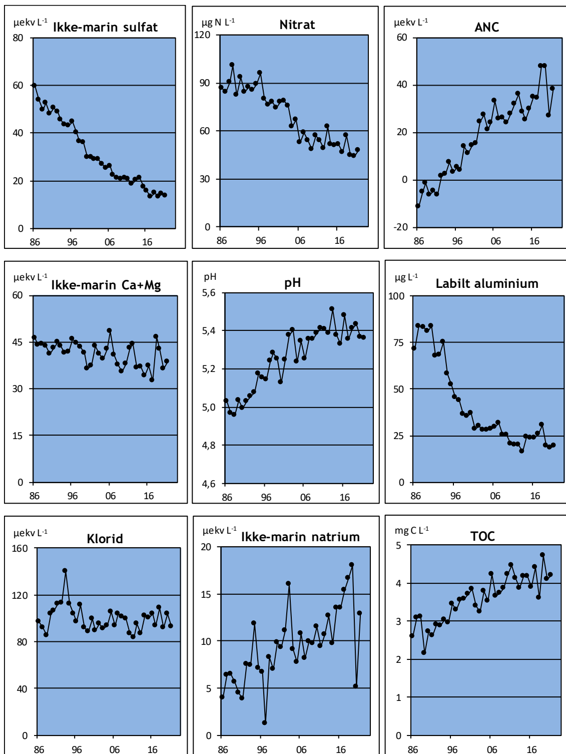
Figur 3. Årlige gjennomsnittskonsentrasjoner fra 1986 til 2021 av et utvalg av parametere i 78 forsursfølsomme innsjøer fordelt over hele landet.
