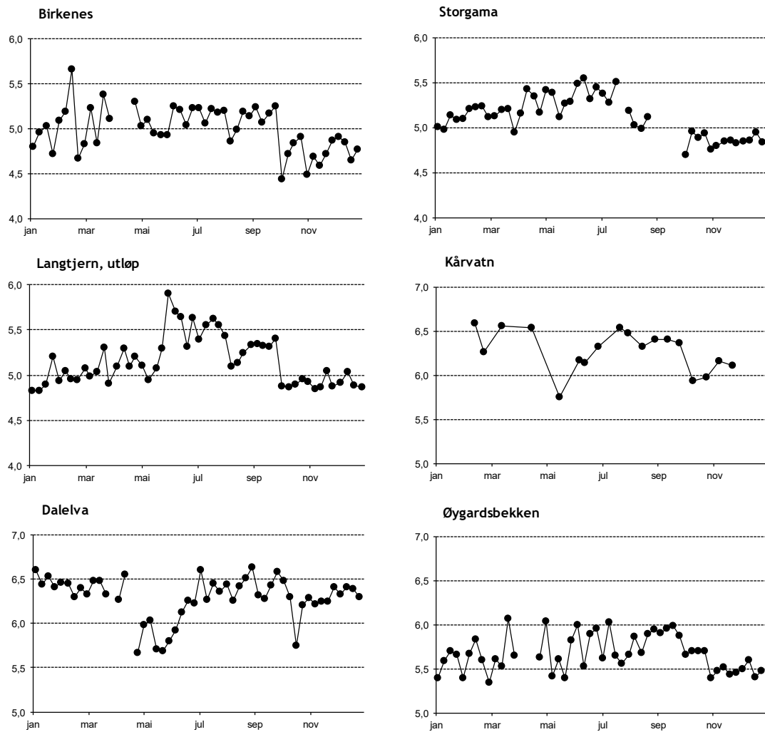
Figur 14. Sesongmessig fluktuasjoner i pH ved feltforskningsstasjonene i 2021. NB! Ulike skalaer på y-aksene.
