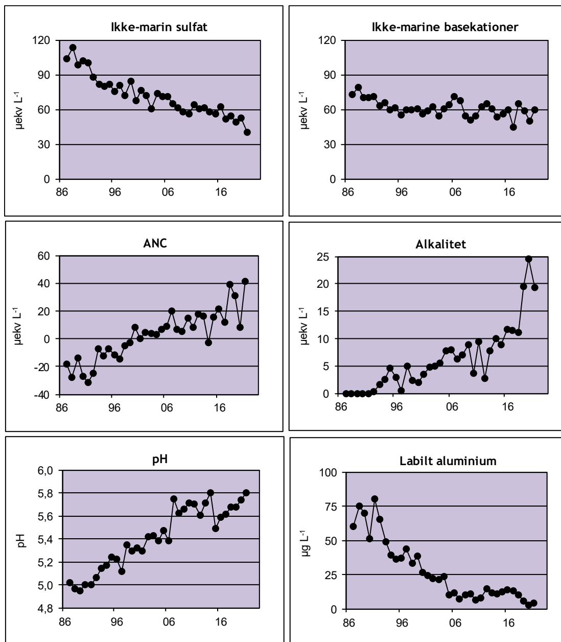
Figur 11. Forsuringsparametere for seks små innsjøer på Jarfjordfjellet for perioden 1987-2021. Middelverdier for ikke-marin sulfat ( \text{SO}_4^* ), ikke-marine divalente basekationer ( \text{Ca}+\text{Mg}^* ), syrenøytraliserende kapasitet (ANC), alkalitet, pH og labilt aluminium.
