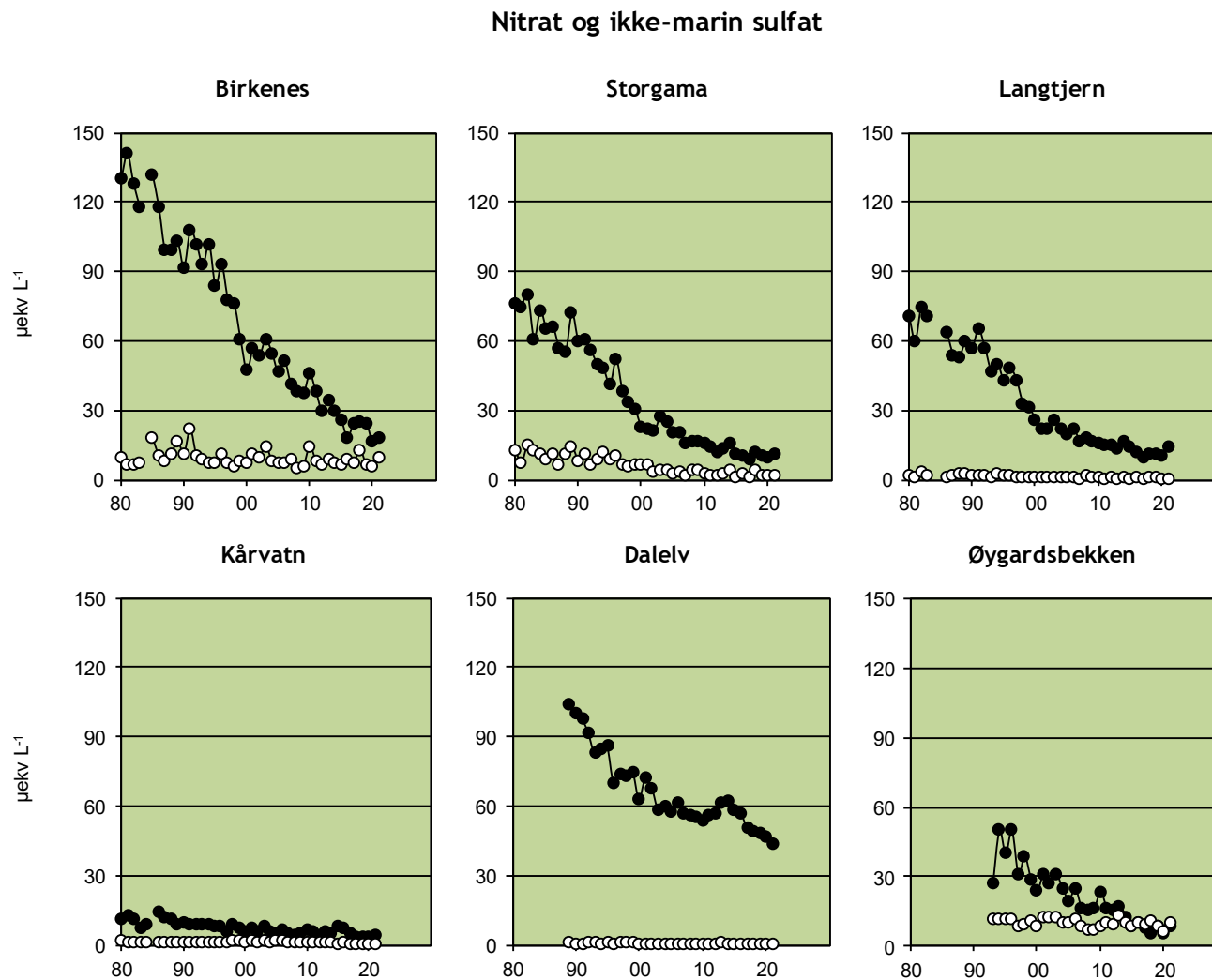
Figur 20. Volumveide konsentrasjoner av nitrat (NO 3 ) og ikke-marin sulfat (SO 4 * ) ved feltforskningsstasjonene for perioden 1980-2021. SO 4 * ● og NO 3 ○. Enhet: µekv L -1 .
