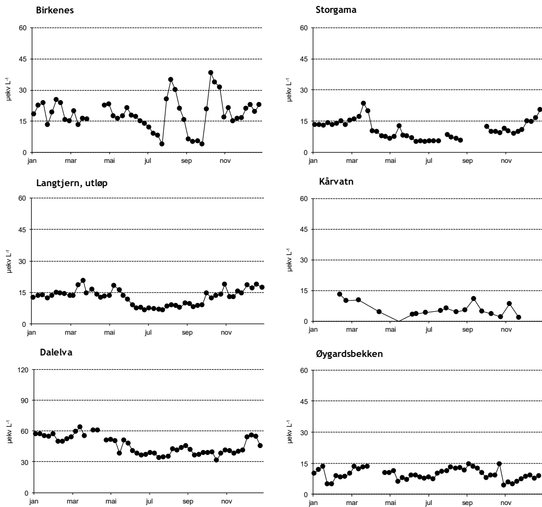
Figur 13. Sesongmessig fluktuasjoner i konsentrasjonene av ikke-marin sulfat ( \text{SO}_4^* ) ved feltforskningsstasjonene i 2021. NB! Ulik skala på y-aksene. Enhet: \mu\text{ekv L}^{-1} .
