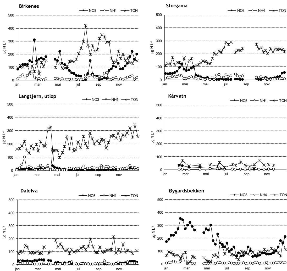
Figur 19. Sesongmessig fluktuasjoner i konsentrasjonene av nitrat (NO 3 ), ammonium (NH 4 ) og totalt organisk nitrogen (TON) ved feltforskningsstasjonene i 2021. TON = totalt nitrogen – NO 3 – NH 4 . NO 3 ●, NH 4 ○ og TON ✕. Enhet: µg N L -1 .
