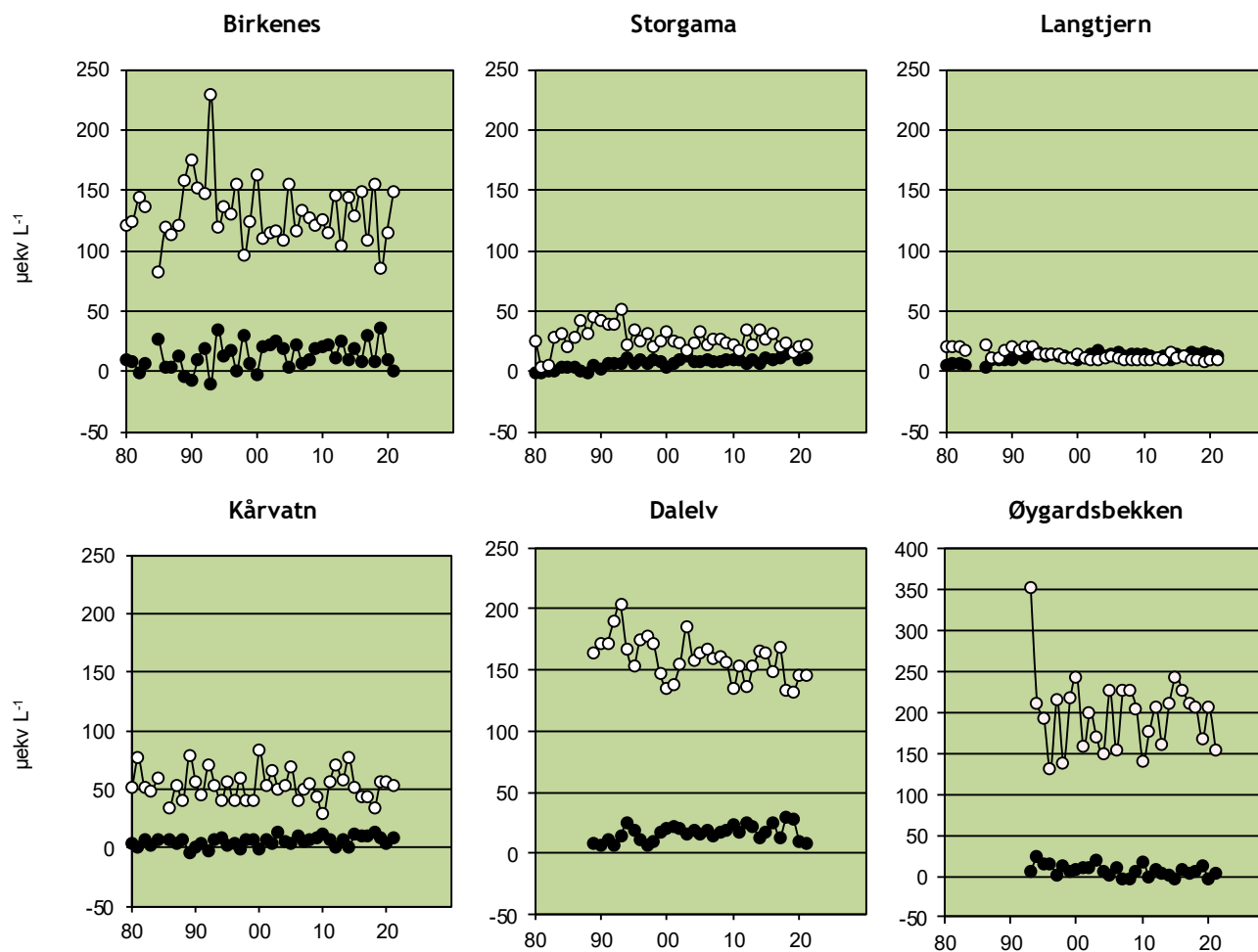
Figur 23. Volumveid konsentrasjoner av klorid (Cl - ) og ikke-marin natrium (Na + ) ved feltforskningsstasjonene for perioden 1980-2021. Na + ● og Cl - ○. Enhet: µekv L -1 . NB! Ulik skala på y-aksen til Øygardsbekken
