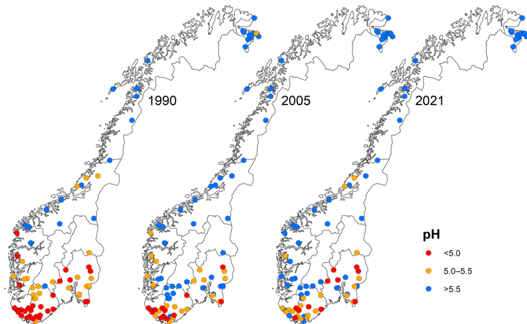
Figur 2. pH i tidstrendsjøene i 1990, 2005 og 2021. Figuren illustrerer tydelig forbedringen i forsureningssituasjonen, ved at sjøene blir mindre sure (får høyere pH). pH i enkelte sjøer på Østlandet er imidlertid fortsatt lavere enn 5. Dette kommer av høyt og økende humusinnhold som gir naturlig lav pH.
