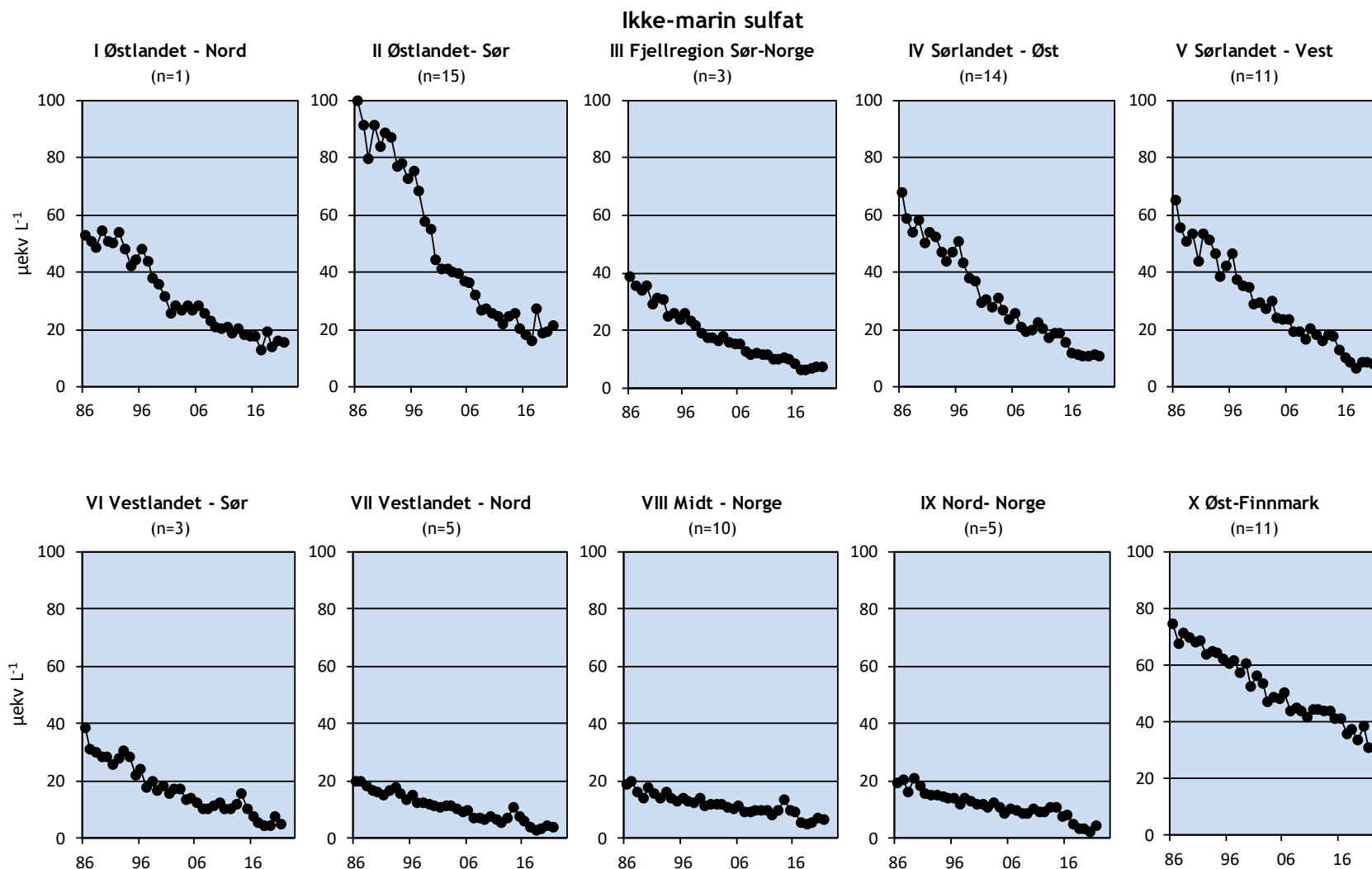
Figur 4. Årlige gjennomsnittskonsentrasjoner av ikke-marin sulfat ( \text{SO}_4^* ) for innsjøene fra hver av de 10 regionene for perioden 1986-2021 beskrevet i Vedlegg 1. Enhet: \mu\text{kv L}^{-1} . n angir antall innsjøer i hver region.
