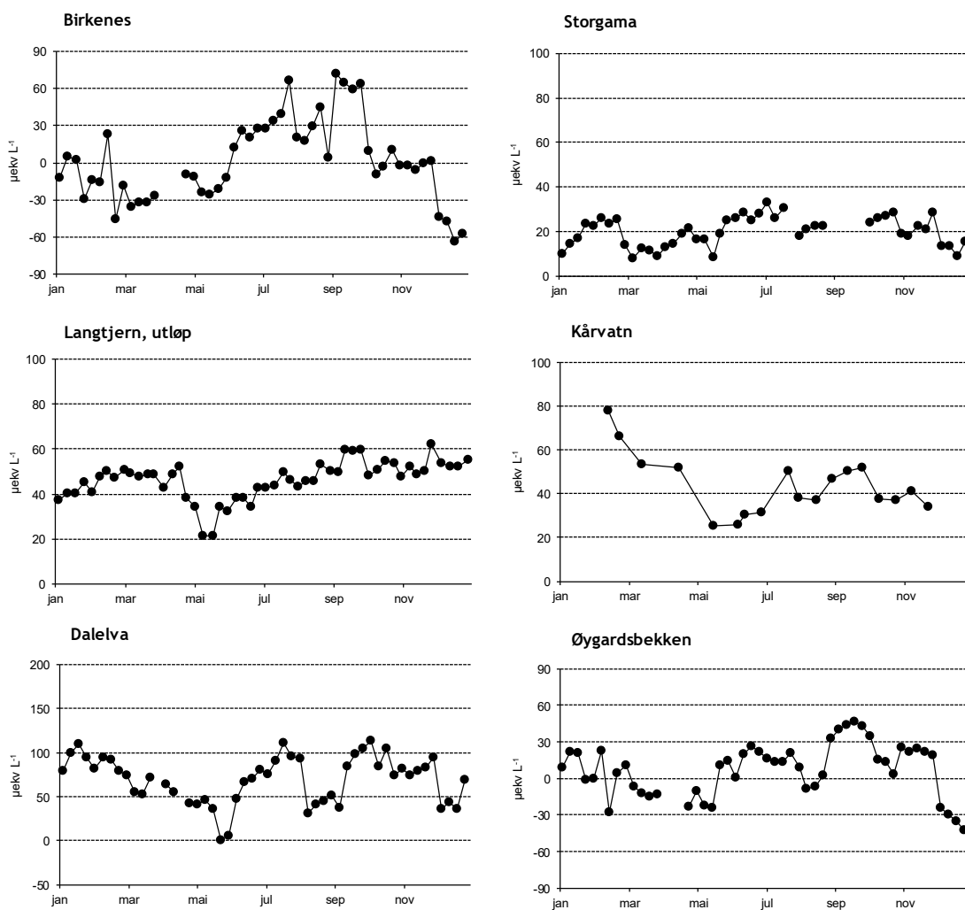
Figur 17. Sesongmessig fluktuasjoner i konsentrasjonene av syrenøytraliserende kapasitet (ANC) ved feltforskningsstasjonene i 2021. NB! Ulik skala på y-aksene. Enhet: \mu\text{ekv L}^{-1} .
