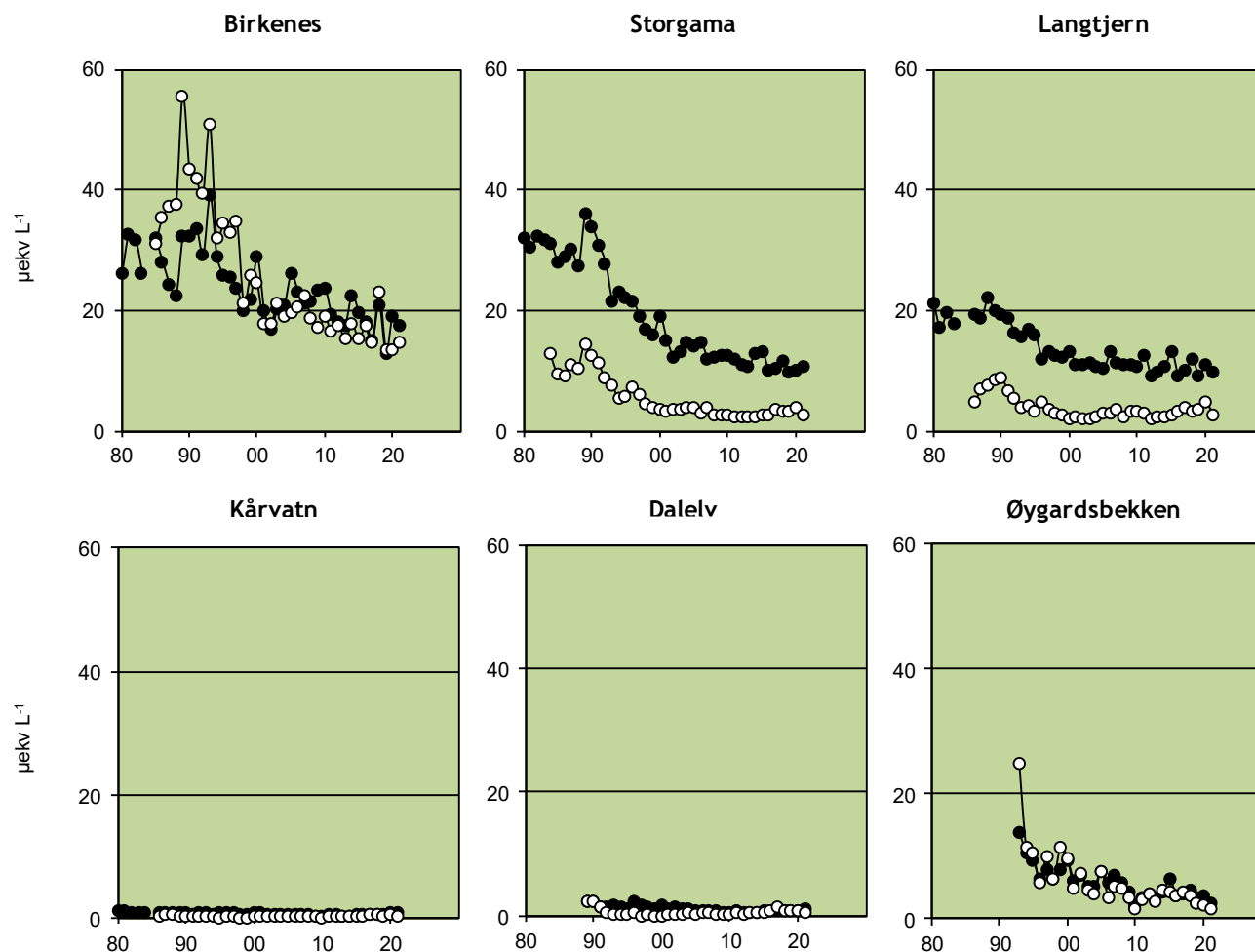
Figur 22. Volumveide konsentrasjoner av hydronium ioner (H + ) og labilt uorganisk aluminium (LAI) ved feltforskningsstasjonene for perioden 1980-2021. H + ● og labilt Al ○. Enhet: µekv L -1 .
