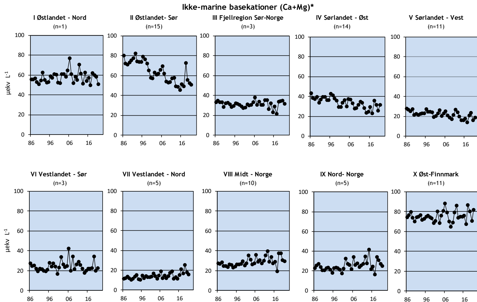
Figur 7. Årlige gjennomsnittskonsentrasjoner av summen av de ikke-marine basekationene Ca og Mg ((Ca+Mg)*) i innsjøene for hver av de 10 regionene for perioden 1986-2021. Enhet: µekv L -1 . n angir antall innsjøer i hver region.
