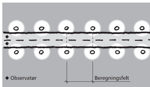
Figur 4.6: 2-felts veg, 2 armaturrekker i siksakk
