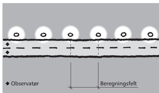
Figur 4.4: 2-felts veg, ensidig armaturrekke
