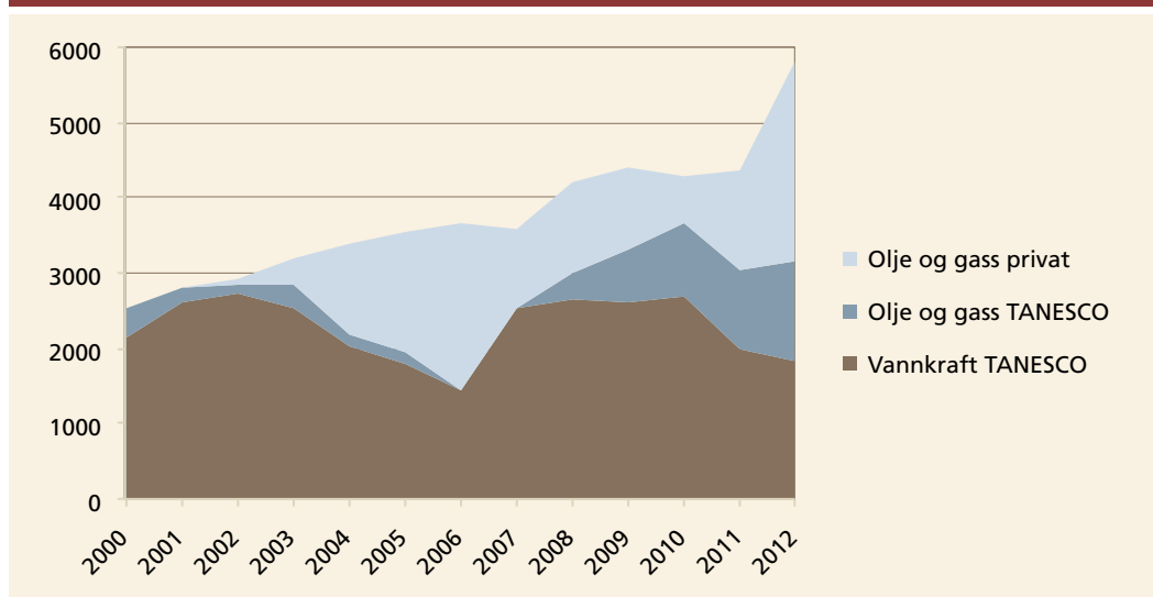
Figur 6 Total kraftproduksjon i Tanzania i perioden 2000–2012 (GWh)
