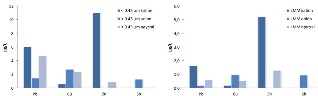
Figur 3.2 Ladningsfordeling av Pb, Cu, Zn og Sb i Kyrkjønn 15. september 2011. Kation = positivt ladet, anion = negativ ladet.
