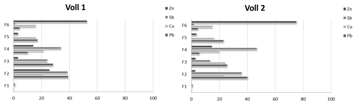
Figur 3.4 Sekvensiell ekstraksjon av jordvollmasse fra et prøvepunkt ovenfor Kyrkjønn (nær prøvepunkt 2B). Figuren viser prosentandelen som hver fraksjon utgjør av totalkonsentrasjonen av henholdsvis Pb, Cu, Sb og Zn. Fraksjon F1-F3 utgjør den lett løselige, biotilgjengelige fraksjonen. Fraksjon F4 og F5 utgjør henholdsvis metall assosiert med for eksempel til Fe- og Mn-oksider og til organisk materiale. Fraksjon F6 utgjør den syreløselige fraksjonen.
