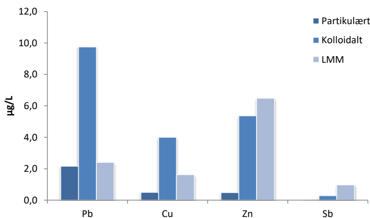
Figur 3.1 Størrelsesfordeling av Pb, Cu, Zn og Sb i Kyrkjønn 15. september 2011 (n=3).
