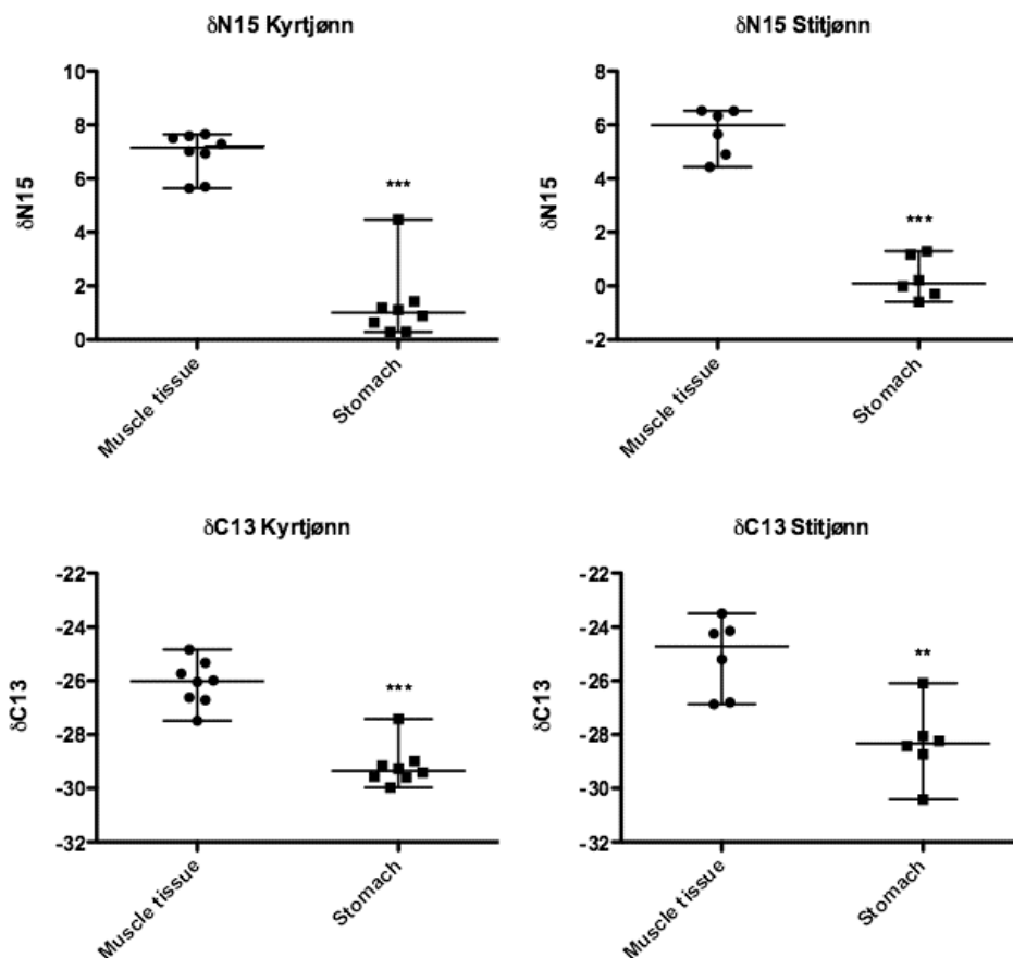
Figur 3.6 Nivået av N15- og C13-isotopen i muskelvev og mageinnhold i ørret fra Kyrkjønn og Stitjønn. Figuren viser medianen og maks- og min-verdier. Det var signifikant forskjell i nivåene av N15- og C13-isotopene mellom ørreten fanget i de to vannene (tosidig Student-t, ** p < 0,01 , *** p < 0,001 ).
