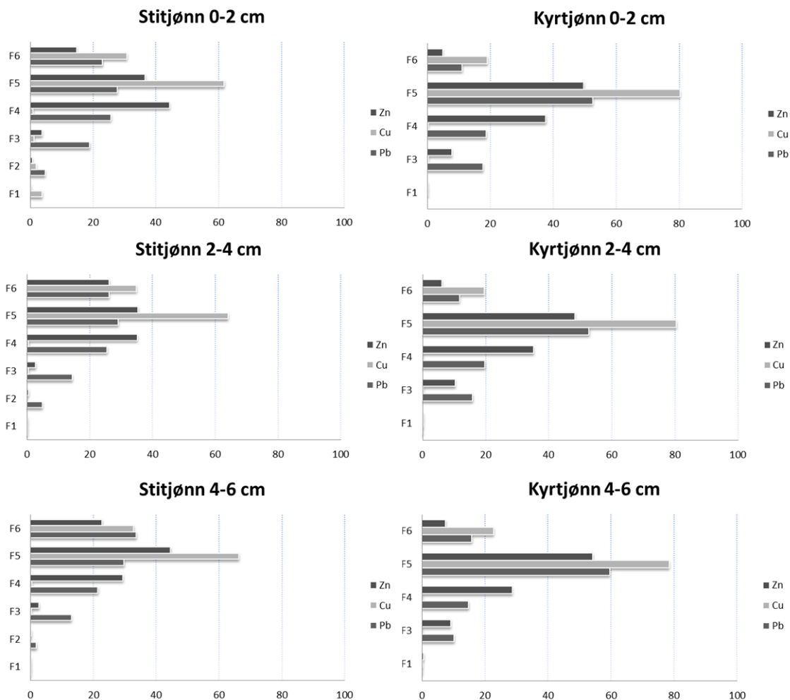
Figur 3.3 Sekvensiell ekstraksjon av bunnsediment fra Stitjønn og Kyrkjønn. Figuren viser prosentandelen som hver fraksjon utgjør av totalkonsentrasjonen av henholdsvis Pb, Cu og Zn. Fraksjon F1-F3 utgjør den lett løselige, biotilgjengelige fraksjonen. Fraksjon F4 og F5 utgjør henholdsvis metall assosiert med for eksempel til Fe- og Mn-oksider og til organisk materiale. Fraksjon F6 utgjør den syreløselige fraksjonen. Konsentrasjonen av Sb var for lav til at man fikk målbare resultater.
