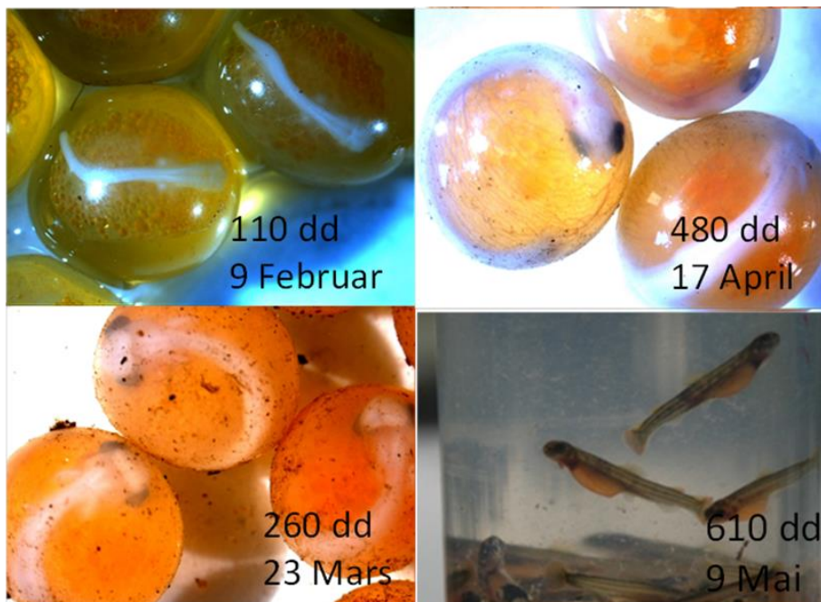
Figur 3.8 Bilder av ørretegg ved forskjellige modningsstadier og nylig utklekket ørret yngel som fortsatt har plommesekken. Dato og antall døgngader (dd) er angitt.
