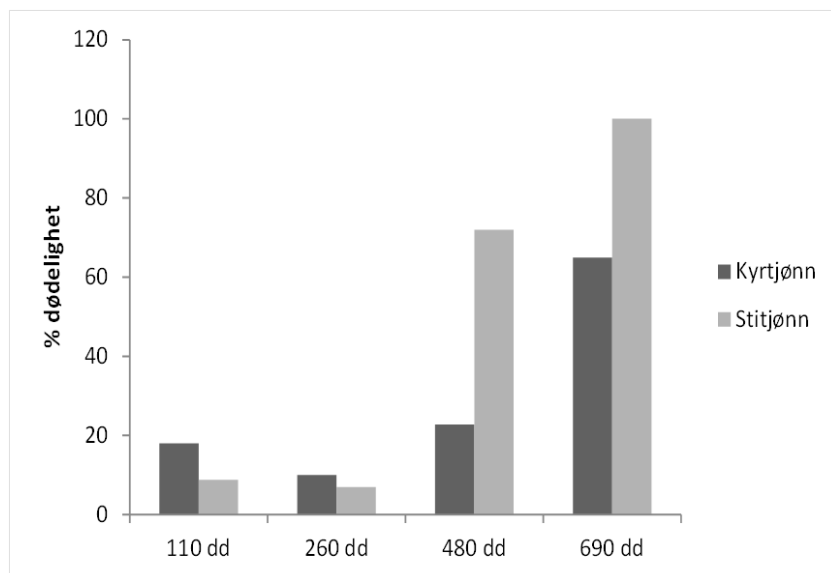
Figur 3.9 Prosent dødelighet blant ørretegg (110 dd og 260 dd) og ørret yngel (480 dd og 690 dd) satt ut i henholdsvis Kyrkjønn og Stitjønn ved fire forskjellige tidspunkter i utviklingen.
