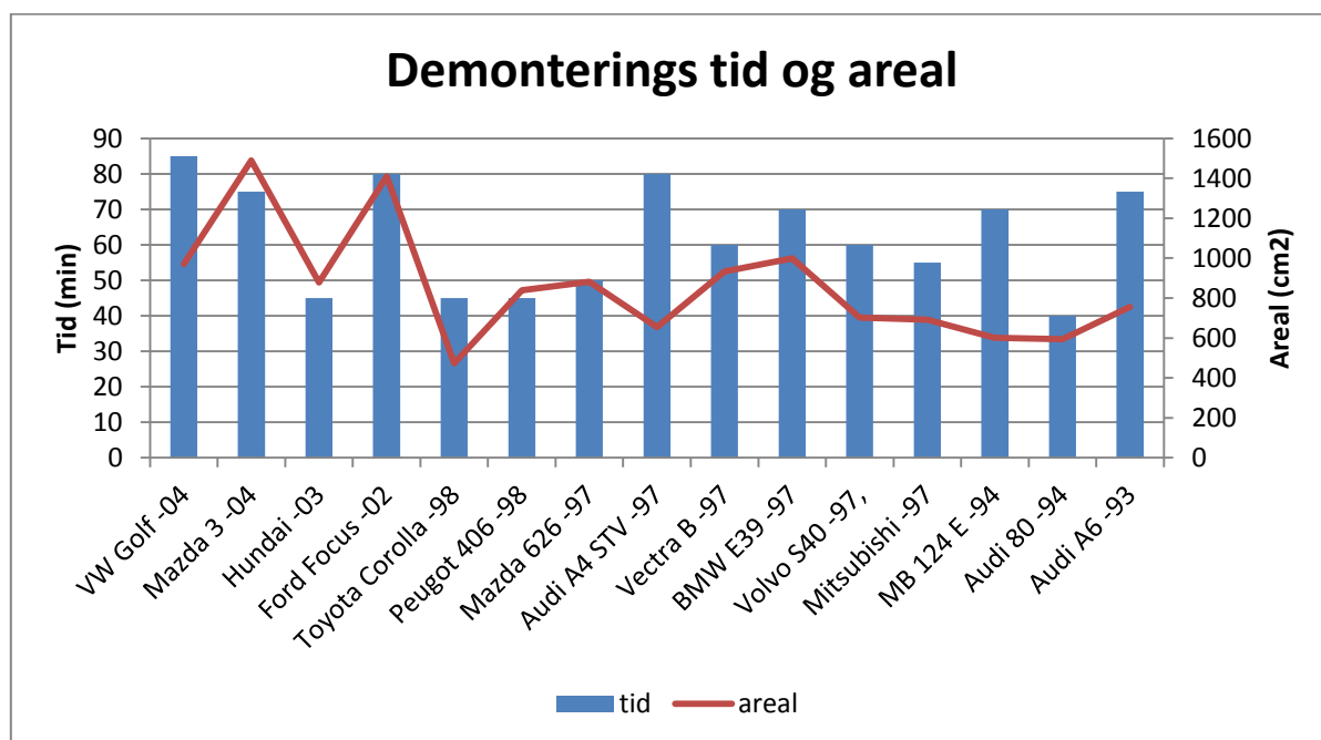
Figur 12. Tidsbruk og areal ved demontering
