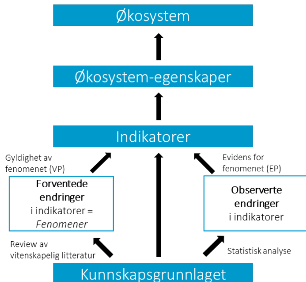
Figur S1. En skematisk oppsummering av hierarkiet i en tilstandsvurdering etter PAEC (fra Pedersen et al. 2021a). De fire primære nivåene i PAEC (blå bokser) er vurderinger av 1) kunnskapsgrunnet, 2) tilstanden til individuelle indikatorer, 3) tilstanden til økosystemegenskaper, og 4) tilstanden til økosystemet som helhet. Vurderingen av individuelle indikatorer baserer seg på i hvilken grad observerte endringer, avdekket ved statistisk analyse (endringsrater) av datagrunnet, er i samsvar med de forventede endringer (uttrykt i fenomenene).
