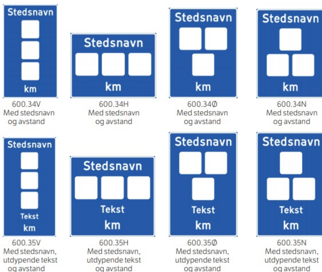
Figur 7.3.7.5—4 — Serviceskilt med 3 symboler
