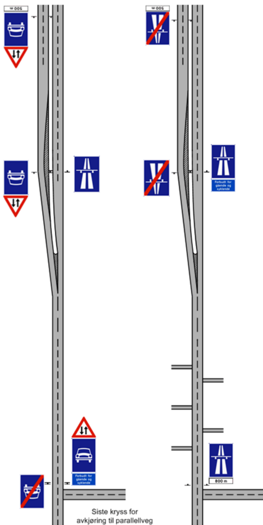
Figur 6.4.1—2 — Eksempler på forvarsling og skilting av motorveg
