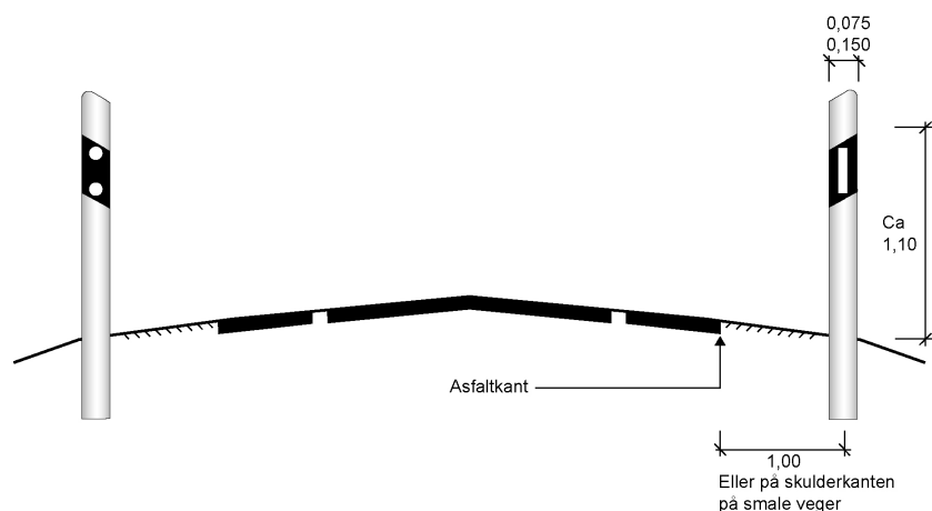
Figur 10.9—5 — Plassering av skilt 920, mål i m
