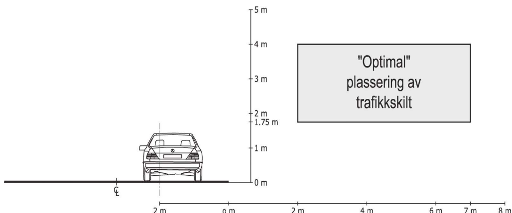
Figur 1.3.3—1 — Område for "optimal" sideplassering av trafikkskilt
