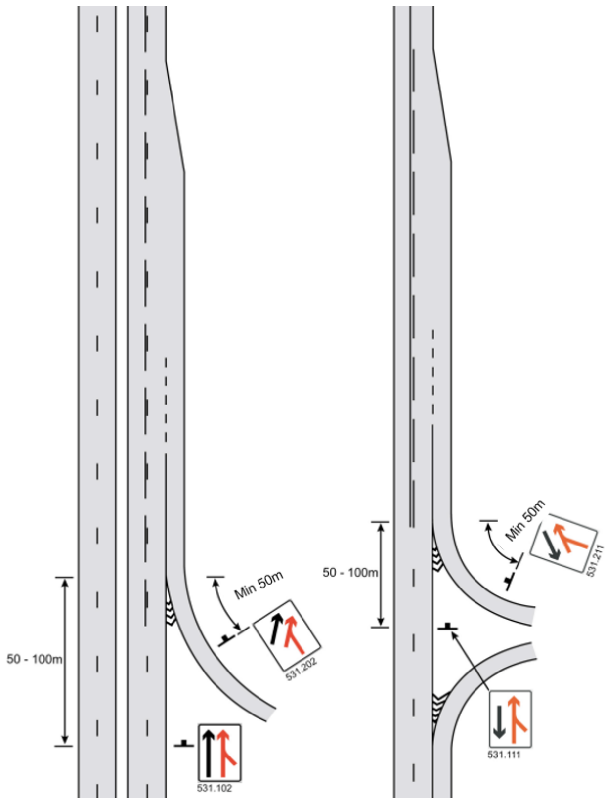
Figur 6.4.25—2 — Skilting av fartsøkingsfelt
