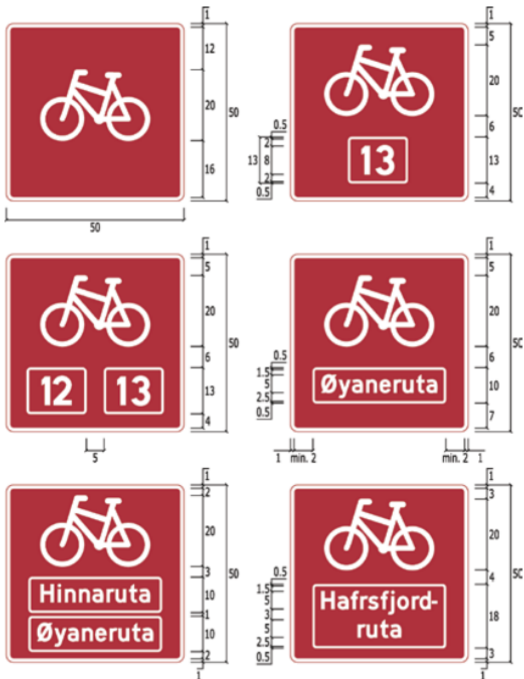
Figur 8.7.3—3 — Eksempler på utforming av skilt 755
