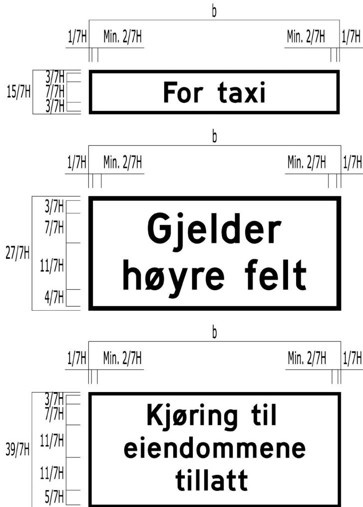
Figur 9.4.5—9 — Plassering av tekst på underskiltene 808.515-557
