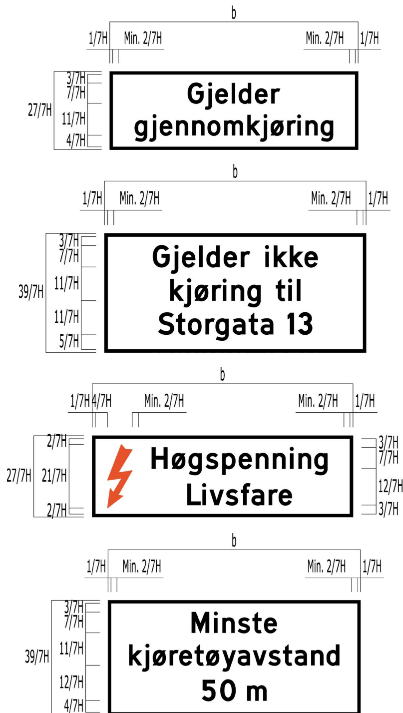
Figur 9.4.5—7 — Plassering av tekst på 808.301-307, 808.339 og 808.343
