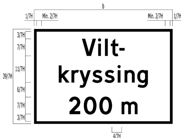
Figur 9.4.5—5 — Eksempel på utforming av kombinert underskilt 808/802
