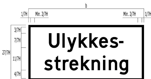
Figur 9.4.5—4 — Plassering av tekst på underskilt 808 - 2 linjer
