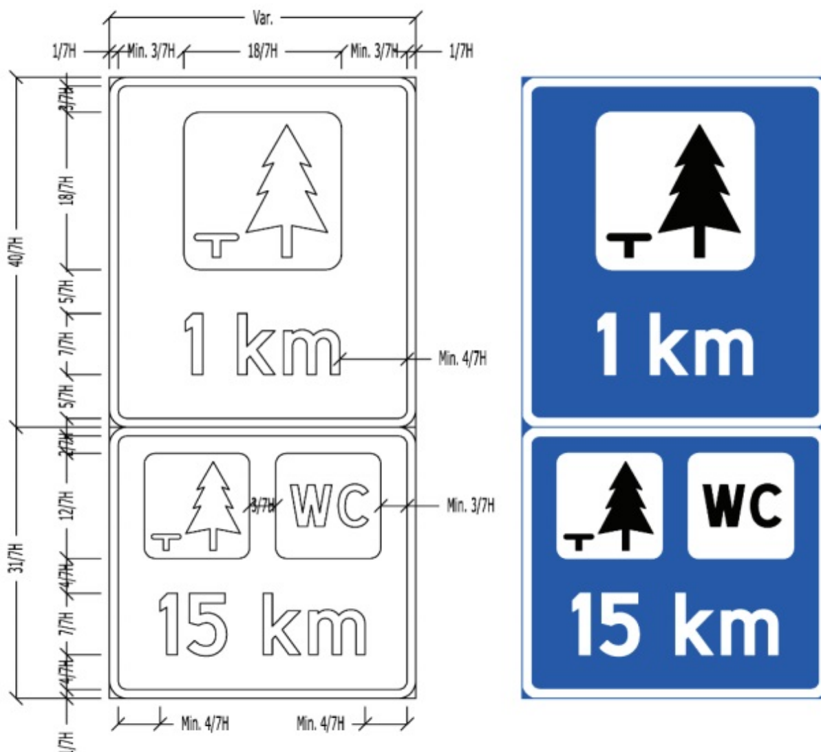
Figur 7.3.7.5—12 — Utforming av skilt som angir avstand til neste tilbud, to symboler (600.12, 600.A2)
