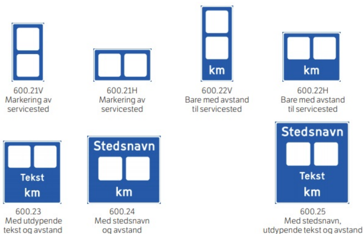
Figur 7.3.7.5—2 — Serviceskilt med 2 symboler
