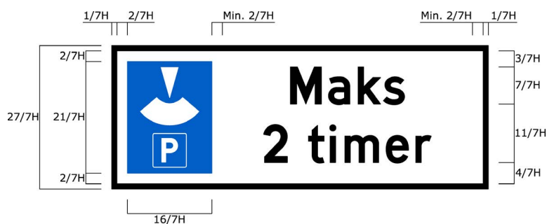
Figur 9.4.17—3 — Utforming av underskilt 831
