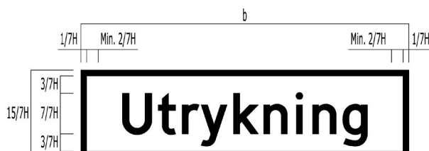
Figur 9.4.5—3 — Plassering av tekst på underskilt 808 - 1 linje
