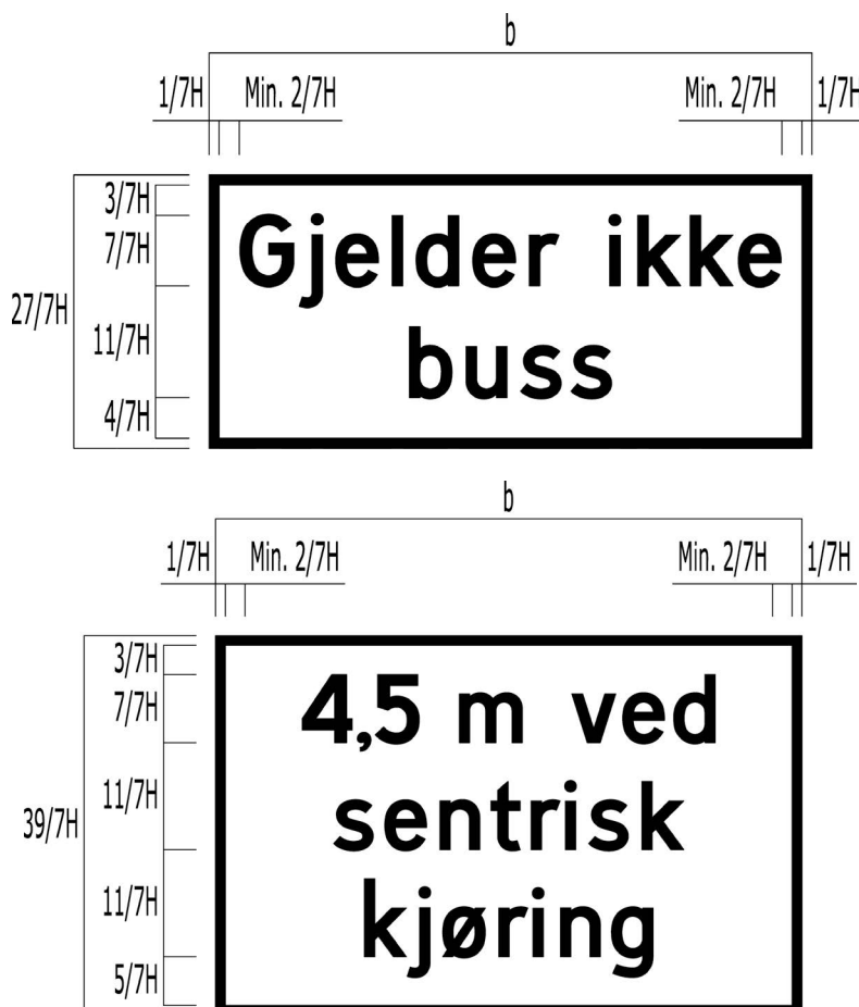
Figur 9.4.5—8 — Plassering av tekst på underskiltene 808.311-333, 808.341 og 808.351
