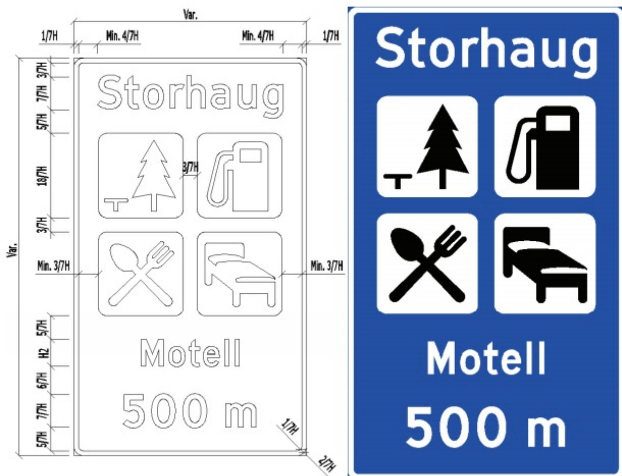
Figur 7.3.7.5—10 — Utforming av serviceskilt med flere symboler, stedsnavn, tekst og avstand (600.45)
