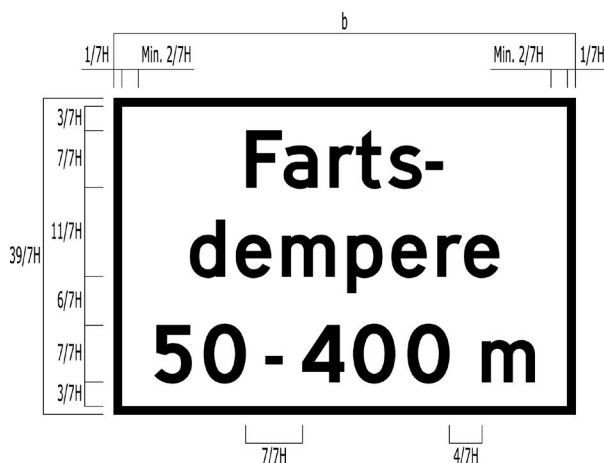
Figur 9.4.5—6 — Eksempel på utforming av kombinert underskilt 808/804
