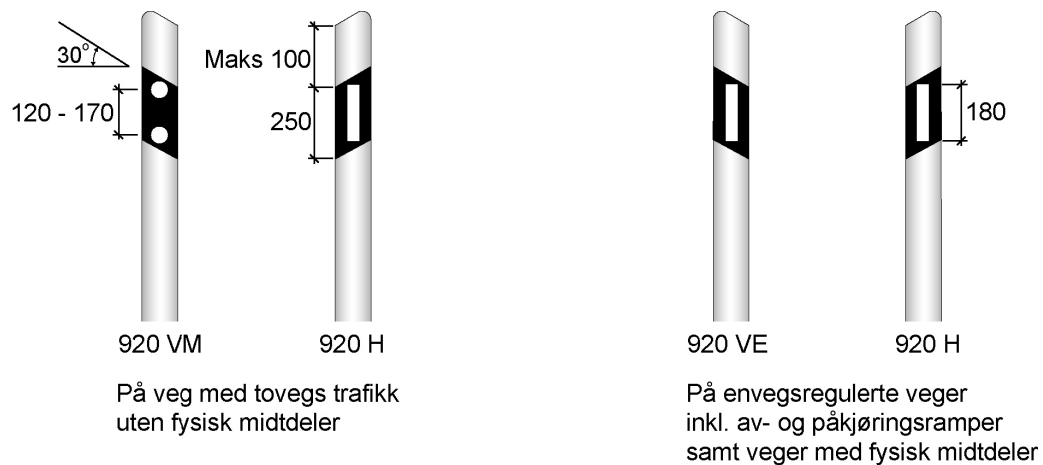
Figur 10.9—6 — Størrelse og utforming av skilt 920, mål i mm
