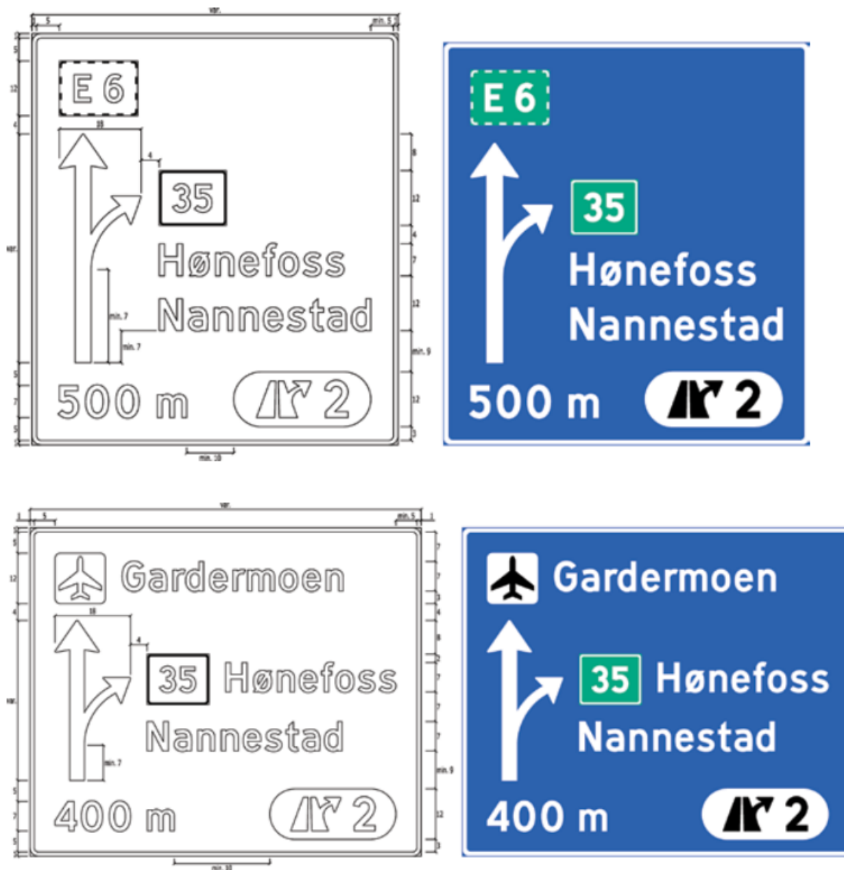
Figur 8.3.5—5 — Eksempler på utforming av avkjøringstavle 705.2
