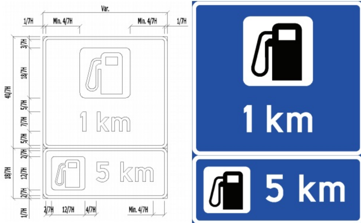
Figur 7.3.7.5—11 — Utforming av skilt som angir avstand til neste tilbud, ett symbol (600.12, 600.A1)
