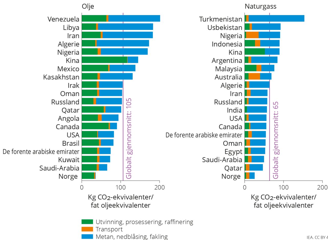
Figur 3.4 Sammenligning av gjennomsnittlig utslippsintensitet i kg CO 2 -ekvivalenter/fat oljeequivalenter i 2022 mellom de største olje- og gassprodusentene. Kilde: IEA (2023b).
