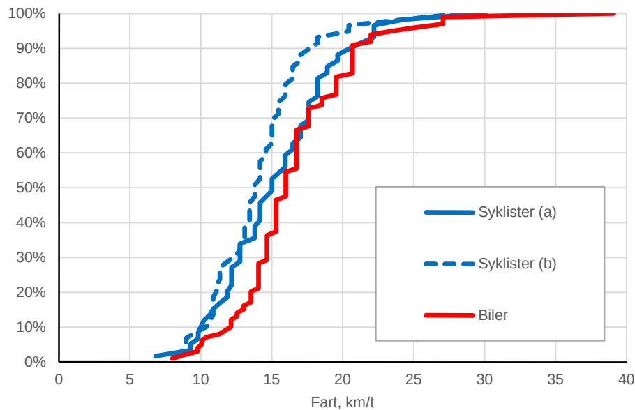
Figur 60. Fartsfordeling blant syklist og biler i krysset Nordre gate/Dronningens gate i Trondheim
