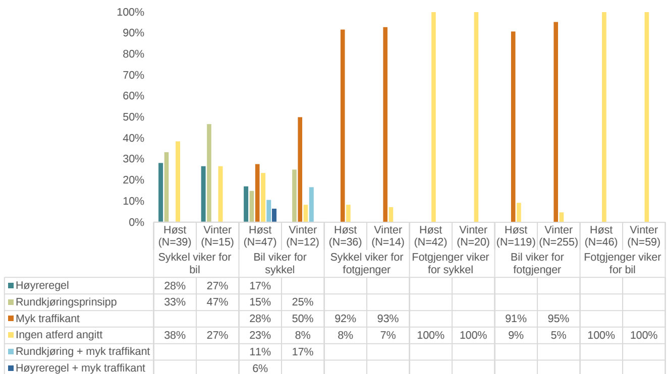
Figur 32. Vikeatferd fordelt ut fra ulike prinsipper for vikepraksis mellom sykkel, bil og fotgjenger på St. Olavs plass, høsten 2016. Prosent.
