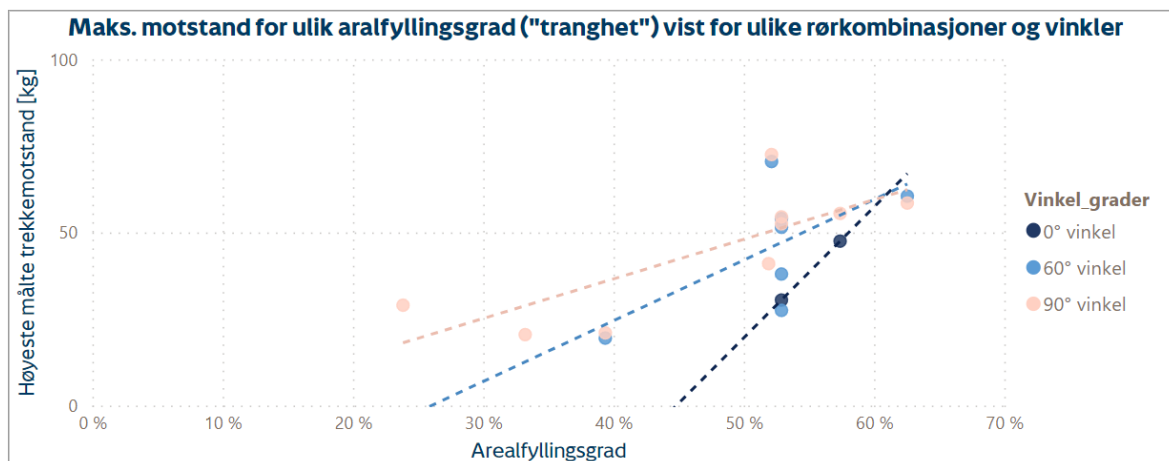
Diagram 8: Sammenstilling av nødvendig trekkekraft for ulike arealfyllingsgrader og vinkler. Her er kun resultatene fra mai vist.
