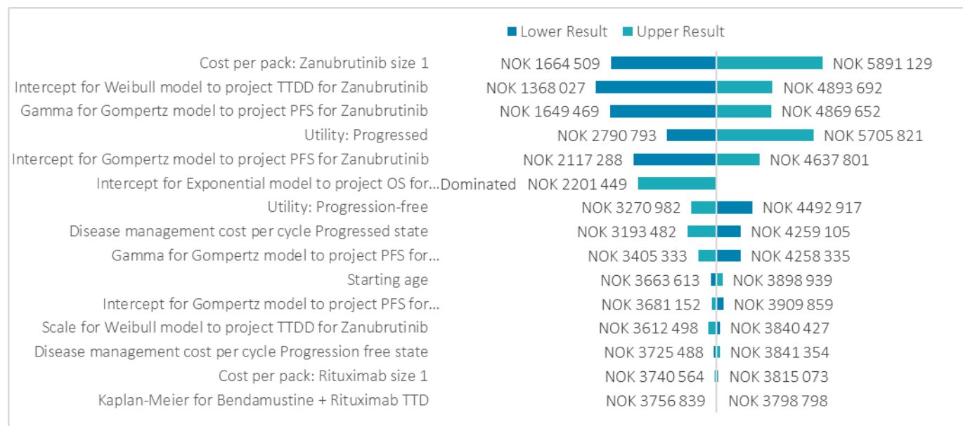
Figur 11. Tornado diagram basert på DMPs analyse 1 (viser hvordan de ulike parameterne påvirker resultatene)
