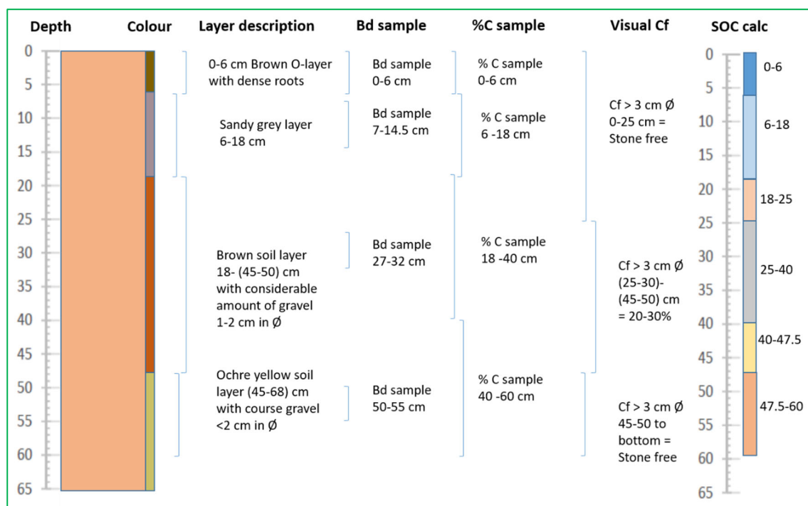
Figur 5.4 Lag i en av profilene (Dindalen G2) i relasjon til parametre beskrevet i teksten over, og jordprøvene som ble tatt
