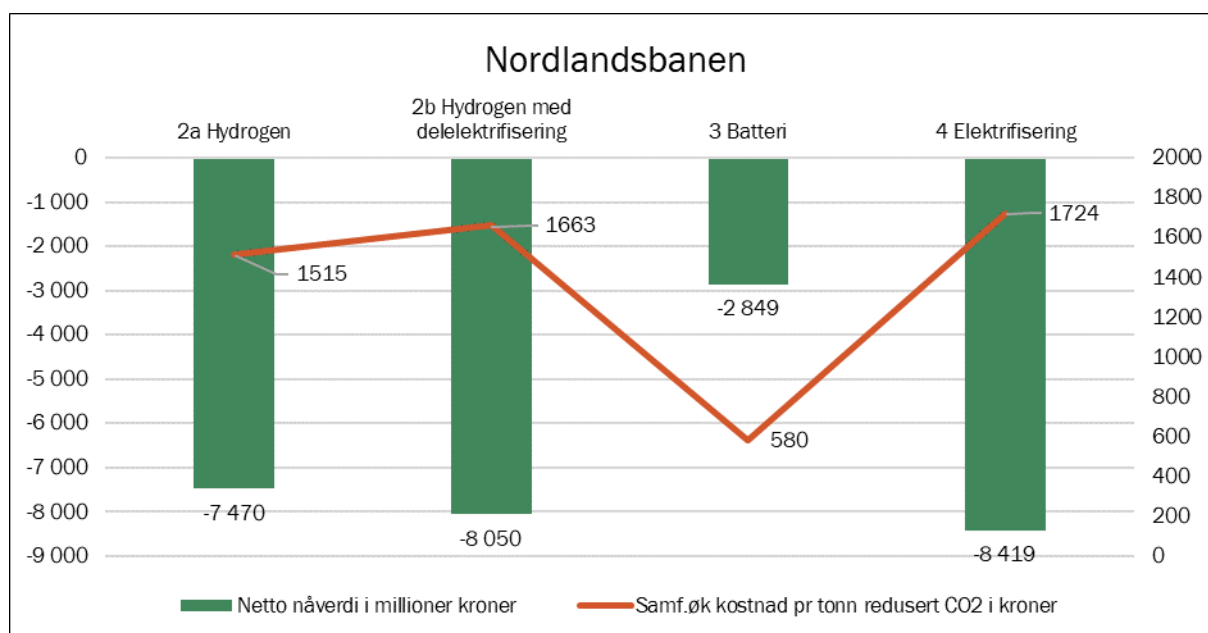
Figur 22: Netto nåverdier og samfunnsøkonomiske kostnader per tonn redusert CO 2 -utslipp for Nordlandsbanen
