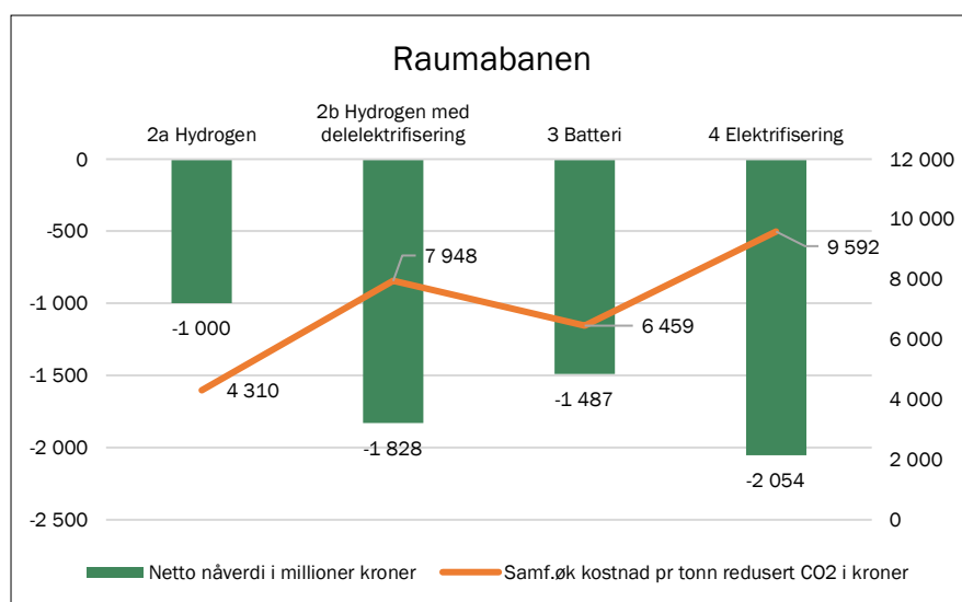
Figur 3 Netto nåverdier og samfunnsøkonomiske kostnader per tonn redusert CO 2 -utslipp på Raumabanen.
