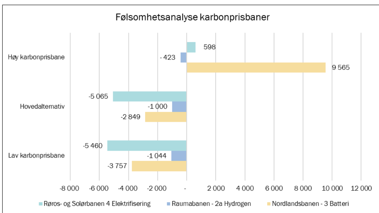
Figur 27: Følsomhetsanalyse karbonprisbaner. Netto nåverdi i millioner kroner
