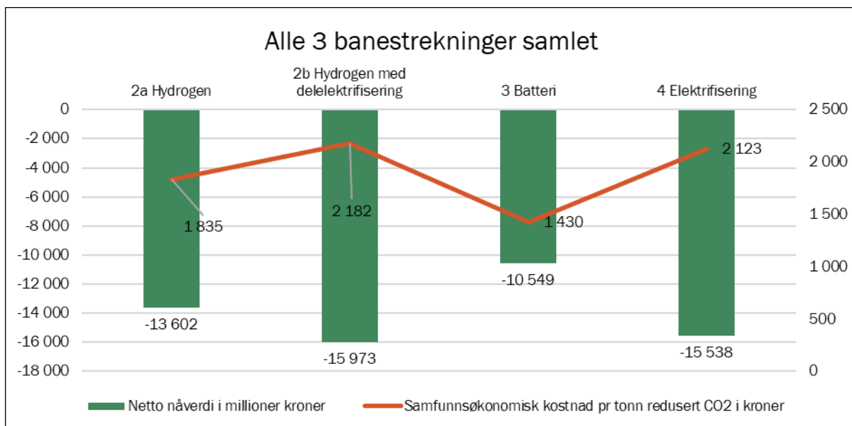
Figur 25: Netto nåverdier og samfunnsøkonomiske kostnader per tonn redusert CO 2 -utslipp for alle 3 banestrekninger samlet
