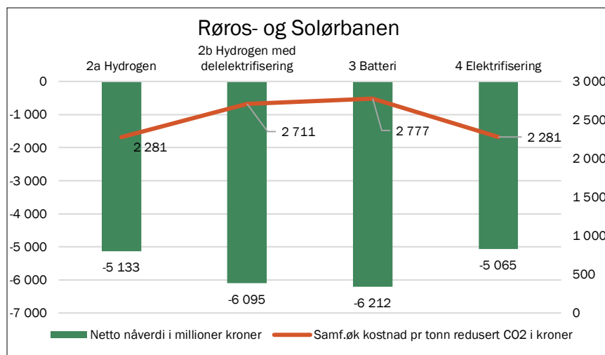
Figur 2 Netto nåverdier og samfunnsøkonomiske kostnader per tonn redusert CO 2 -utslipp på Røros- og Solørbanen.
