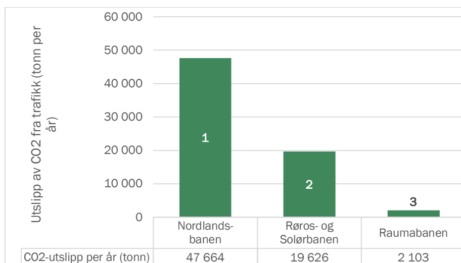
Figur 30 Prioritering av strekninger i KVVU GREEN, samt CO 2 -utslippsreduksjoner per bane, målt opp mot fremtidige beregnede utslipp i 0-alternativet.
