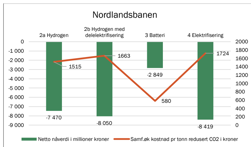
Figur 1 Netto nåverdier og samfunnsøkonomiske kostnader per tonn redusert CO2-utslipp på Nordlandsbanen.
