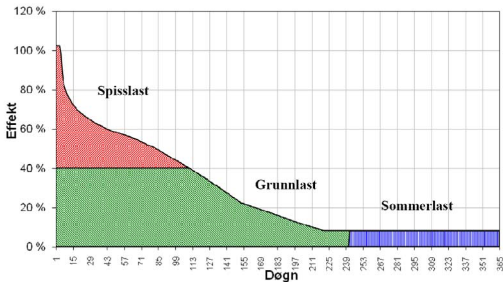
Figur 2.2 Eksempel på varighetsdiagram for oppvarming
