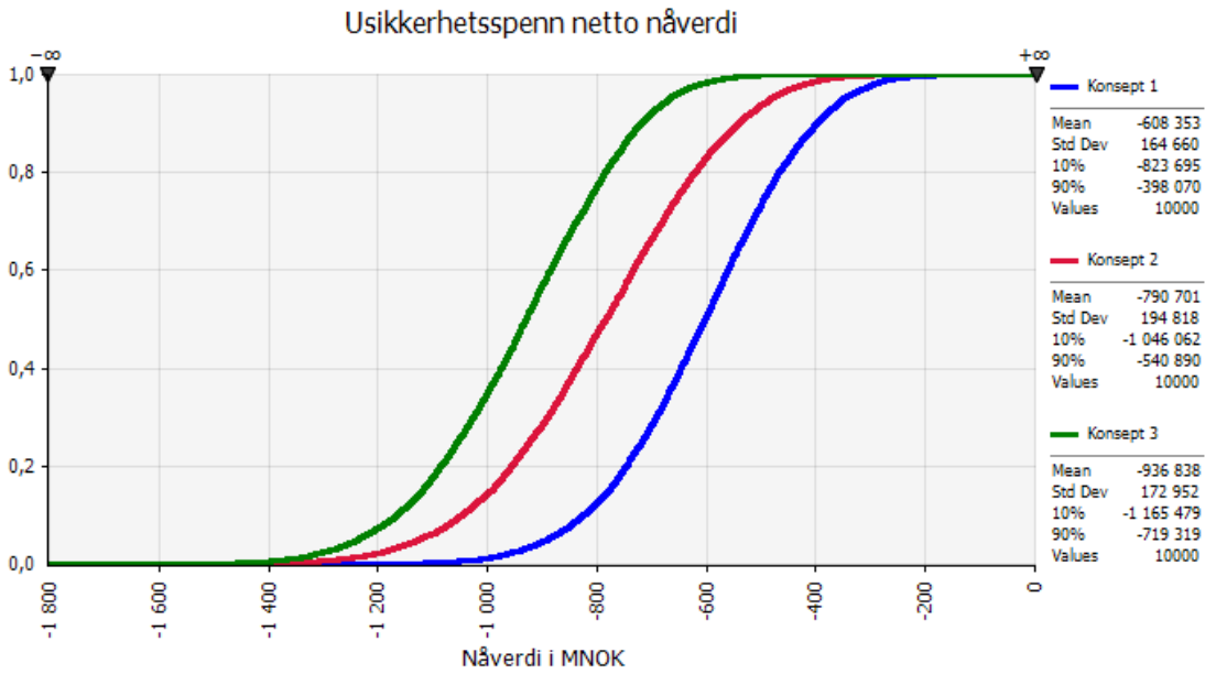
Figur 3: S-kurve netto nåverdi for alternativene
