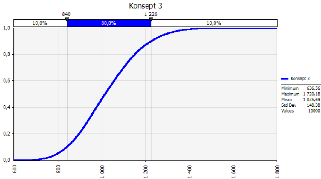
Figur 15: S-kurve Konsept 3 (MNOK)
