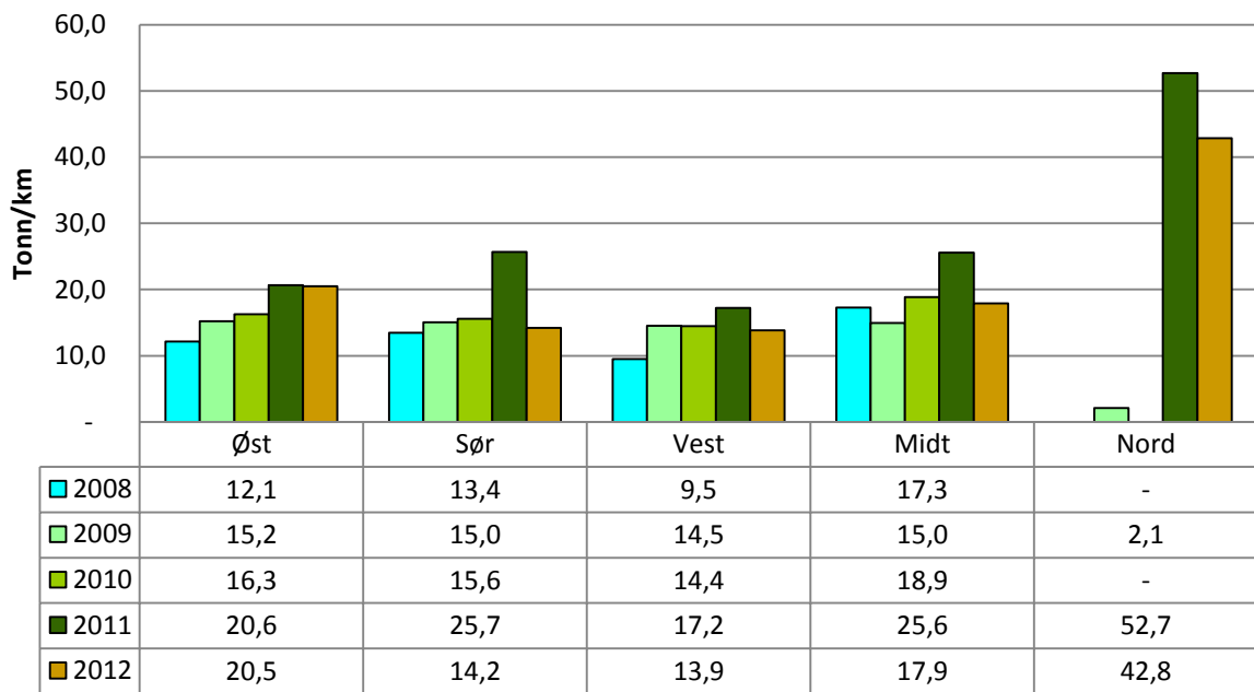
Saltforbruk i tonn/km, strategi bar veg
