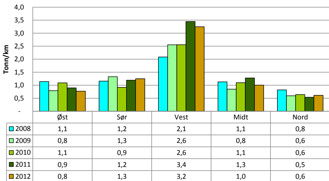
Saltforbruk i tonn/km, strategi vinterveg
