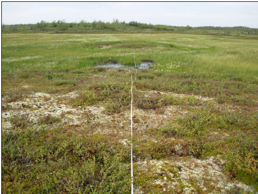
Figur 27: Linje E, krysser to paller og et laggområde mellom de to palsene (posisjon GLE015, se figur 26).
