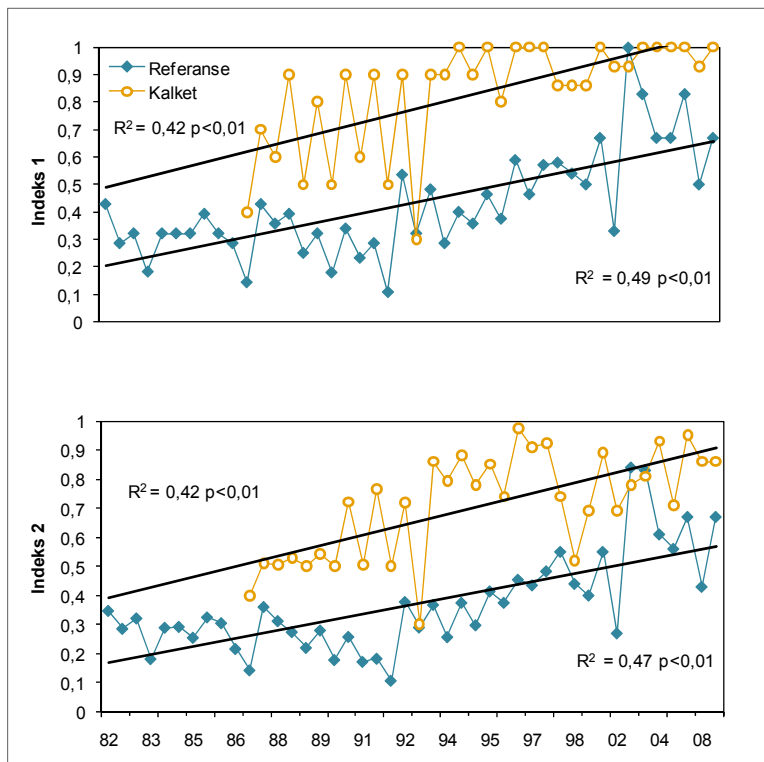
Figur 12.12 Gjenomsnittlig forsuringsindeks for de kalkete stasjonene og for referansestasjonene i Vikedalselva 1982 - 2008. For detaljert beskrivelse av metodikken henvises til Fjellheim & Raddum (1990) (indeks 1) og Raddum (1999) (indeks 2).
