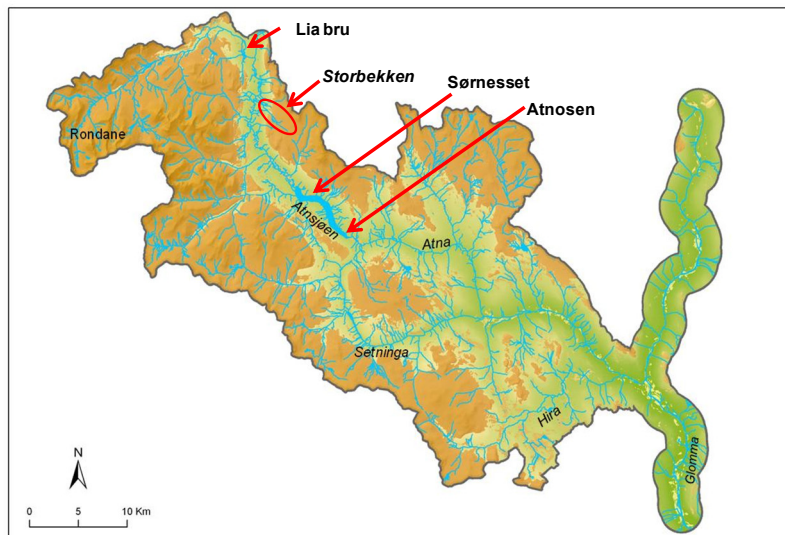
Figur 1.1 Målestasjoner for vanntemperatur (Atnosen), vannføring (Lia bru, Atnosen), snødekke (Storbekken) og lufttemperatur og nedbør (Sørnesset, fram til 1998).
