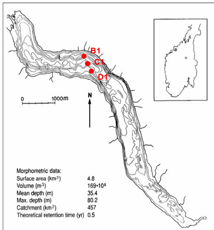
Figur 4.1 Dybdekart (dybdekote 10 m) for Atnsjøen med plassering av dagens stasjoner, stasjonene B1, C1 og D1. (Kilde: NVE).
