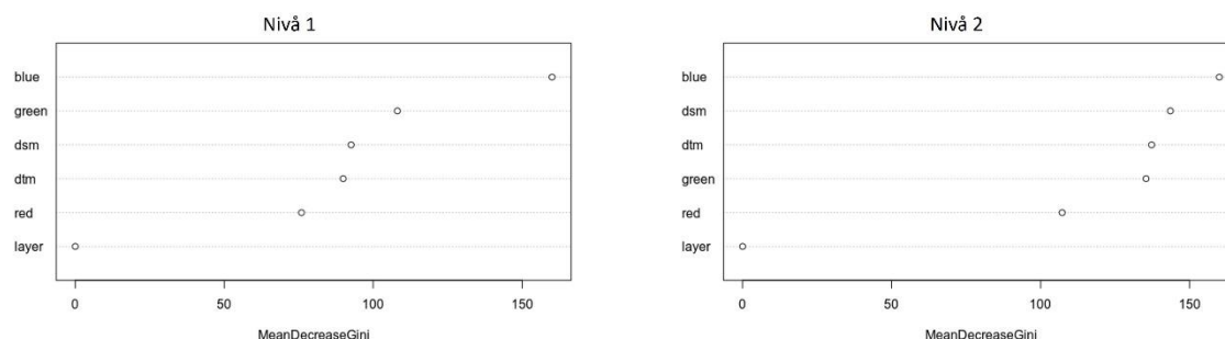
Figur 4.18. Prediktorvariablenes viktighet (langs y-aksen) for å klassifiseringen av arealdekket, på nivå 1 (til venstre) og nivå 2 (til høyre). Variablene som ble brukt, var blått, rødt og grønt bånd. Fra ortofoto, samt digital terrengmodell (DTM) og digital overflatemodell (DEM i figurteksten, DOM i teksten).
