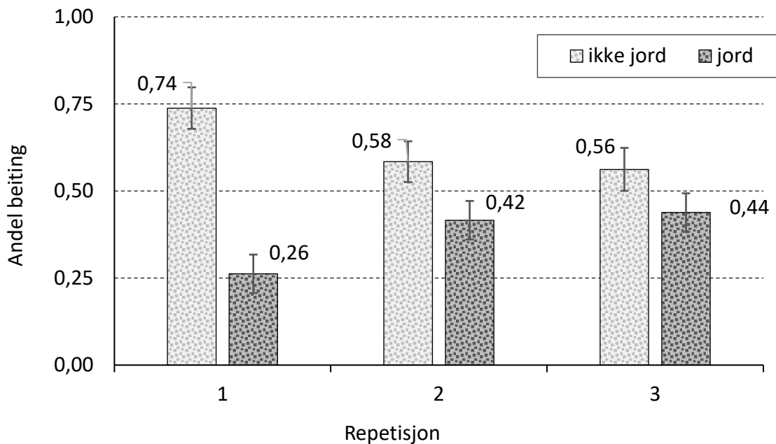
Figur 3.1 Andel av beitetid ( \pm standardfeil) i beiteruter med påstrødd jord (jord) og uten tilført jord (ikke jord), korrigerte snitt (least square means) basert på 9 søyer som beitet i 3 påfølgende repetisjoner i samme forsøksfeltet, med 25 min pause mellom øktene.
