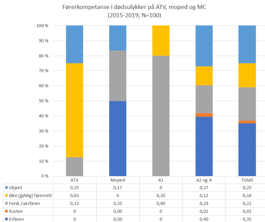
Figur 10. Erfaring/førerkompetanse for fører av ATV (N=8), moped (N=6), lett motorsykel (N=5) og mellom-/tung motorsykel (N=81) ved dødsulykker i perioden 2015-2019 (N=100). Kilde: UAG-rapporter.
