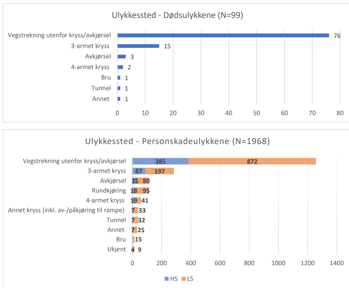
Figur 60. Fordelingen av dødsulykker og personskadeulykker på mellomtung og tung motorsykkel 2-hjul (2015-2020) på ulike ulykkessteder. Presentert i synkende rekkefølge. Kilde: TRULS/TRINE.
