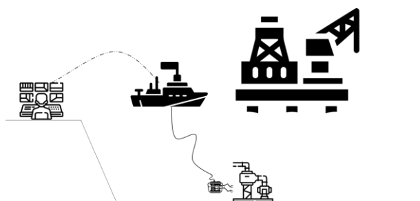
K1. Konvensjonelt ROV-konsept med IMR-fartøy. ROV er forbundet med IMR-fartøy via umbilical. ROV-mannskap om bord IMR-fartøy. Trådløs kommunikasjon til land mulig.
