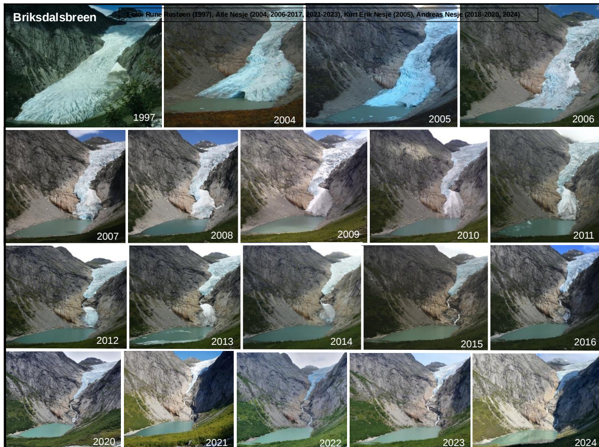
Figur 18. Billedserie av Briksdalsbreen, en utløpsbre på vestsiden av Jostedalsbreen, mellom 1997 og 2024. Navna på fotografene står øverst på figuren
