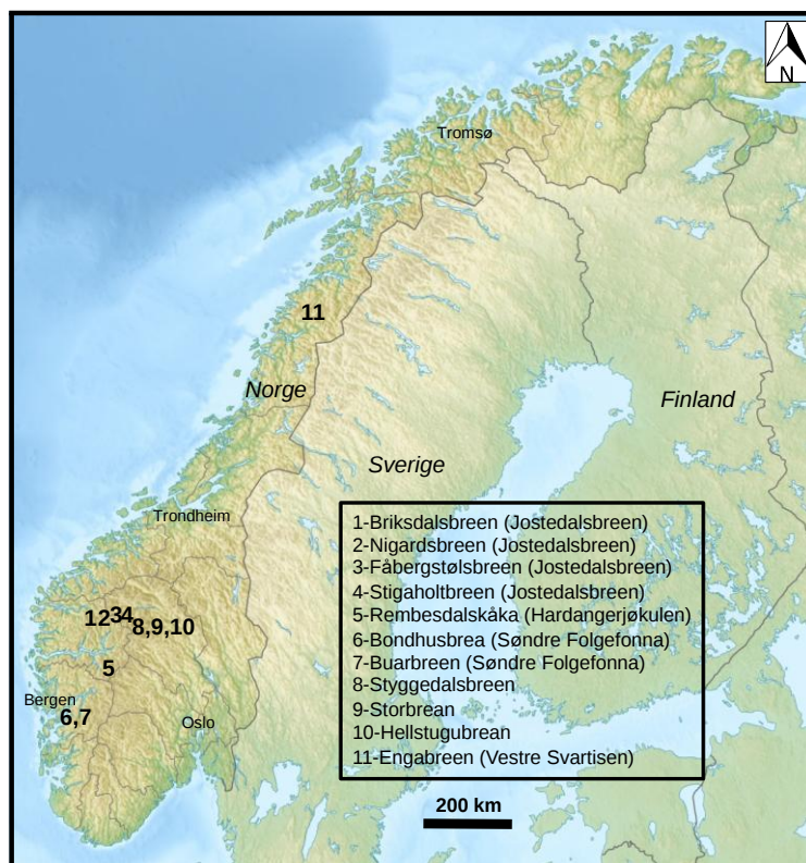
Figur 16. Lokaltetskart over elleve norske breer med lange frontmåleserier (observasjonsperiode i parentes): 1-Briksdalsbreen (1900–2015), 2-Nigardsbreen (1899–), 3-Fåbergstølsbreen (1899–), 4-Stigaholtbreen (1903–), 5-Rembesdalskåka (1917–), 6-Bondhusbrea (1902–), 7-Buarbreen (1900–), 8-Styggedalsbreen (1901–), 9-Storbreen (1902–), 10-Hellstugubreen (1901–), 11-Engabreen (1903–)
