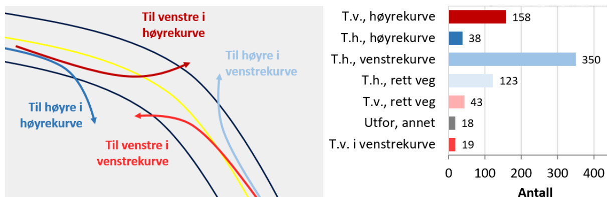
Figur 3.1: Utforkjøringer i kurver. Prinsippsskisse (til venstre) og fordeling av skadde og drept på tung MC (til høyre), (n=749, 2017-2022). Blått = til høyre, og rødt = til venstre; høyrekurve er angitt i mørke farger, og venstrekurve i lysere farger. For utforkjøringer på rette strekninger benytter vi enda lysere blå- og rødfarger for utforkjøringer til henholdsvis høyre og venstre.
