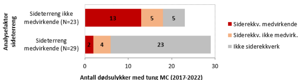
Figur 3.16: Antall dødsulykker med tung MC (2017-2022) som var utforkjøringer, fordelt på ulykker hvor sideterreng var og ikke var medvirkende faktor (henholdsvis nederste og øverste stolpe) og hvor sideterreng var og ikke var til stede eller medvirkende faktor (fargene innenfor stolpene).
