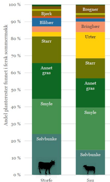
Figur 18. Artssamansetting i diett hos storfe og sau på skogsbeite i Sør-Noreg 2013, snitt av tre område: Ringsaker, Nannestad, Vestskauen. Basert på mikrohologisk identifisering av planterestar i fersk møkk (juli-sept.) (Wam og Herfindal 2020).
