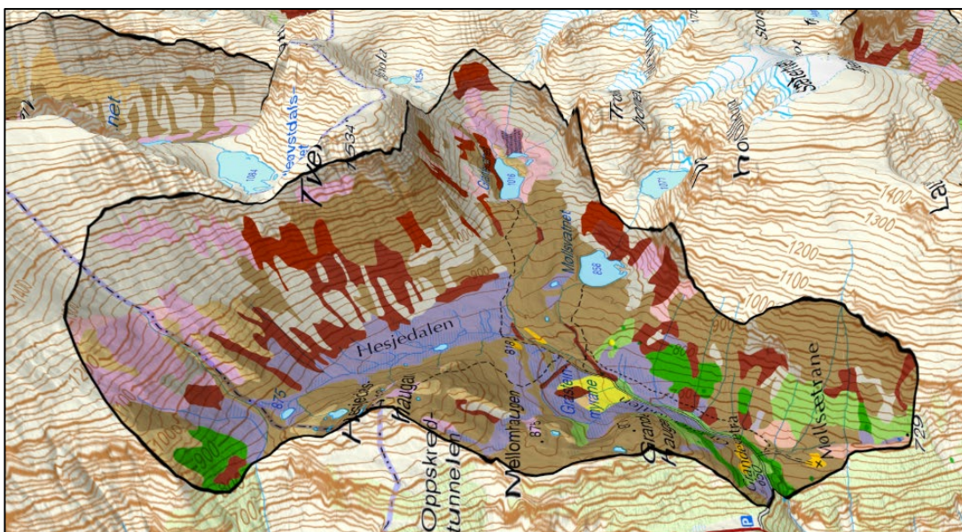
Ortofoto og vegetasjonskart i 3D over Gråsteindalen sett frå vest.
